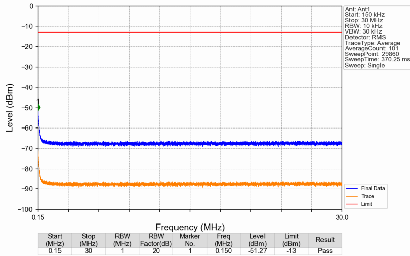
3700MHz-3900MHz_3700.1MHz_GMSK_SISO_Ant1_NTNV
