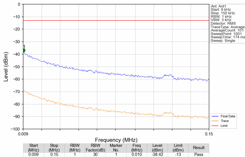
3700MHz-3900MHz_3897.5MHz_AWGN_SISO_Ant1_NTNV
