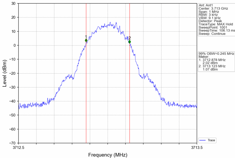
3700MHz-3900MHz_3713MHz_GMSK_SISO_Ant1_NTNV_AGC+3
