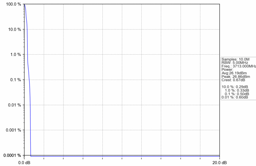
3700MHz-3900MHz_3713MHz_GMSK_SISO_Ant1_NTNV_AGC+3
