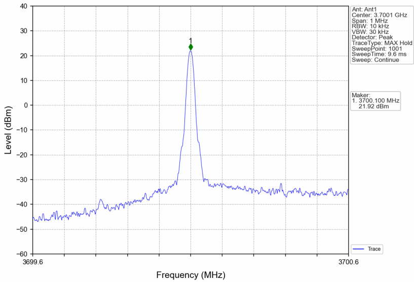
3700MHz-3900MHz_3700.1MHz_CW_SISO_Ant1_NTNV
