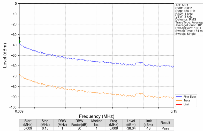
3700MHz-3900MHz_3700.1MHz_GMSK_SISO_Ant1_NTNV
