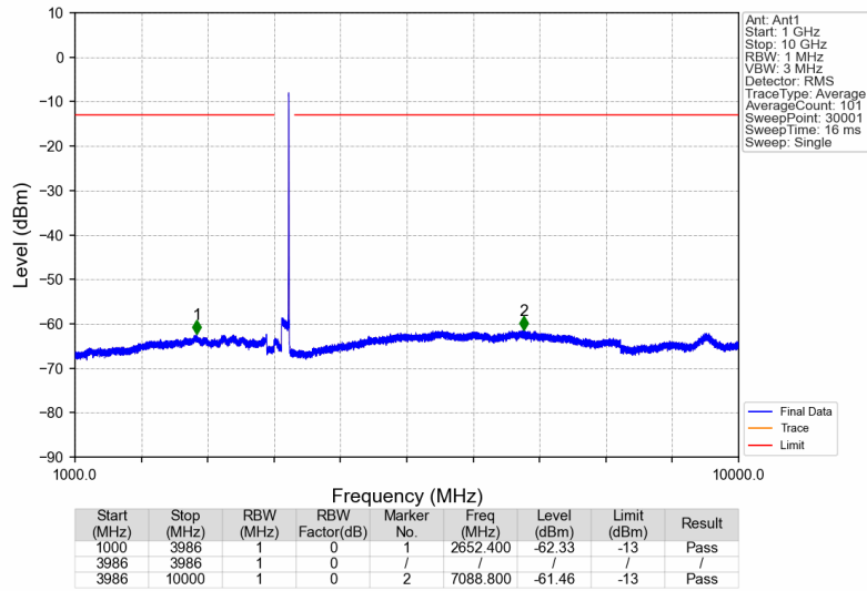
3700MHz-3900MHz_3897.5MHz_AWGN_SISO_Ant1_NTNV
