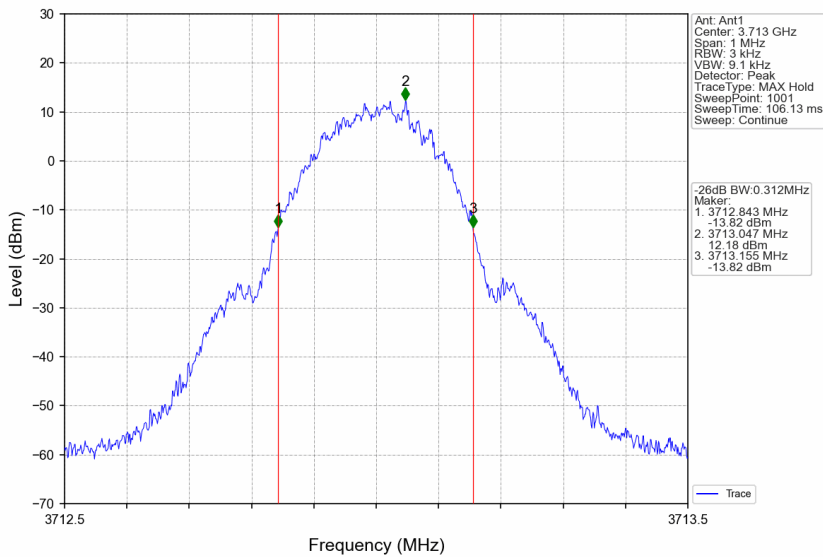
3700MHz-3900MHz_3713MHz_GMSK_SISO_Ant1_NTNV_AGC+3
