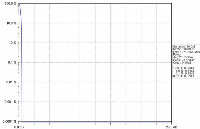
3700MHz-3900MHz_3713MHz_GMSK_SISO_Ant1_NTNV_AGC
