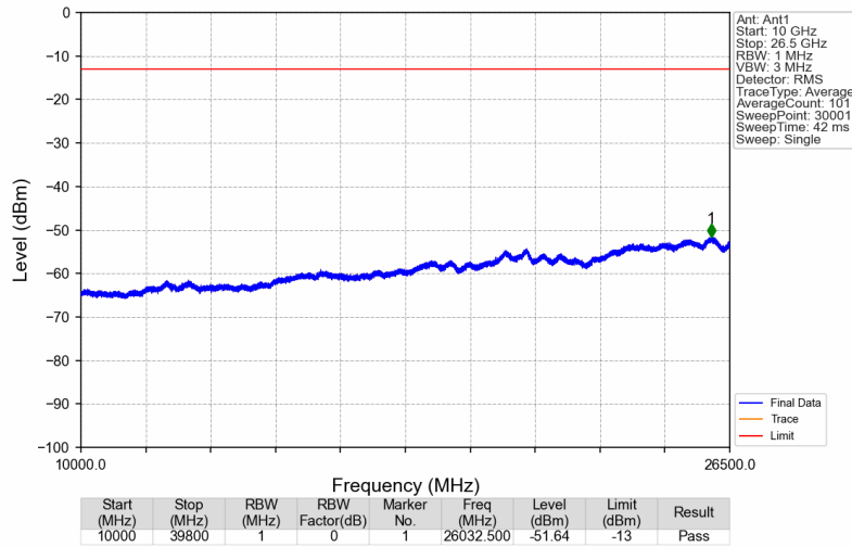
3700MHz-3900MHz_3897.5MHz_AWGN_SISO_Ant1_NTNV
