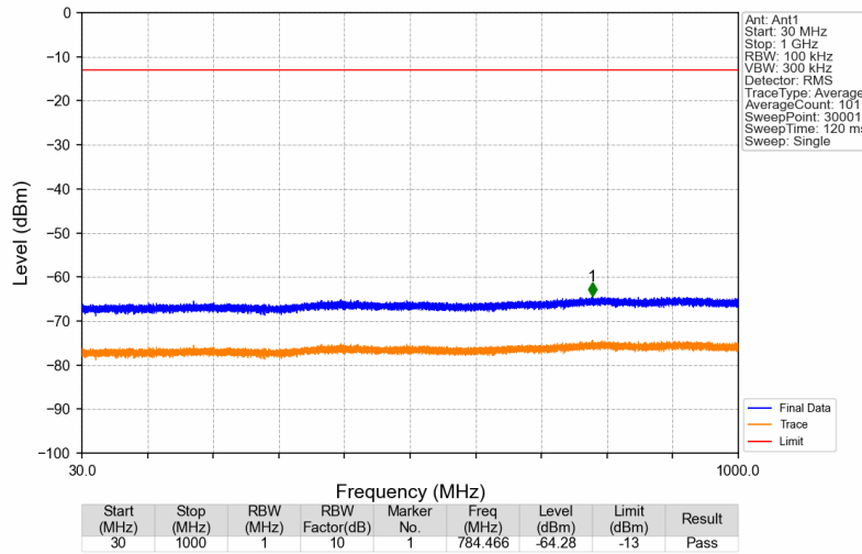
3700MHz-3900MHz_3700.1MHz_GMSK_SISO_Ant1_NTNV
