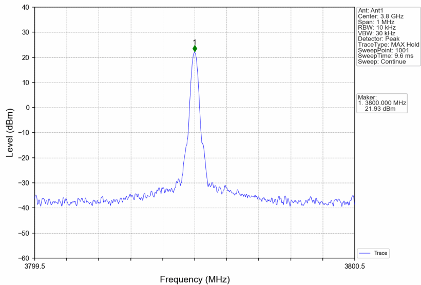
3700MHz-3900MHz_3800MHz_CW_SISO_Ant1_NTNV
