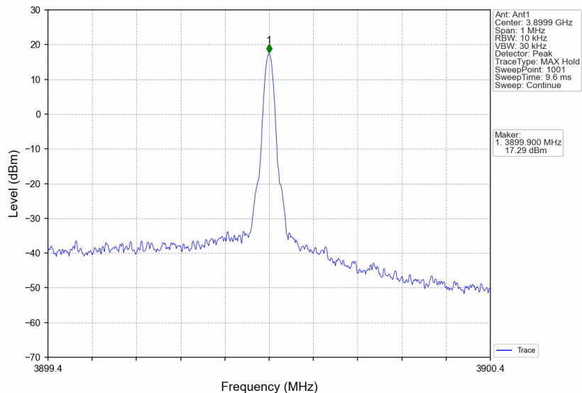
3700MHz-3900MHz_3899.9MHz_CW_SISO_Ant1_NTNV
