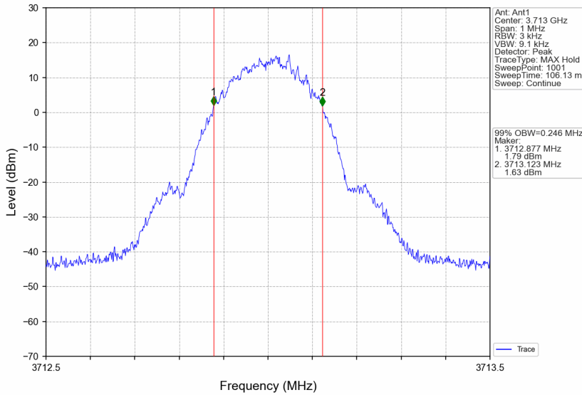
3700MHz-3900MHz_3713MHz_GMSK_SISO_Ant1_NTNV_AGC+3
