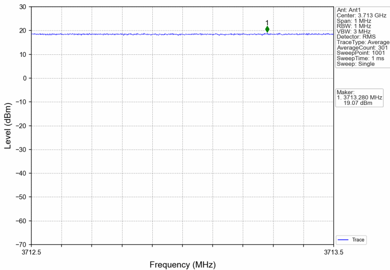
3700MHz-3900MHz_3713MHz_GMSK_SISO_Ant1_NTNV_AGC+3
