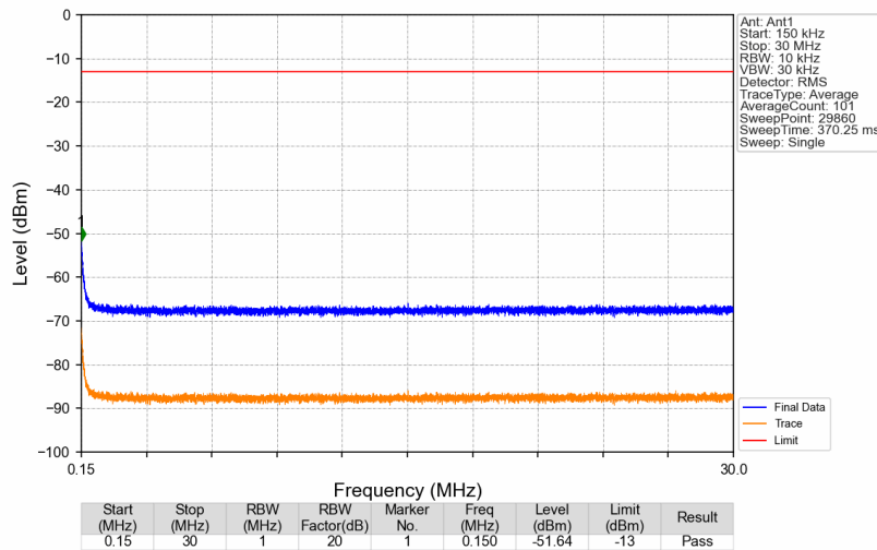
3700MHz-3900MHz_3897.5MHz_AWGN_SISO_Ant1_NTNV
