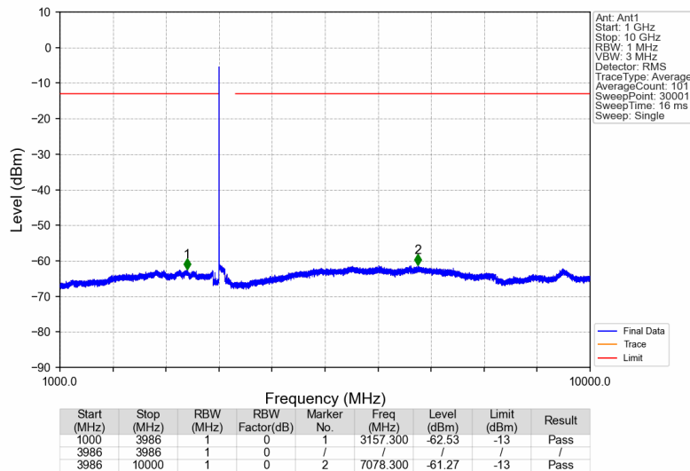
3700MHz-3900MHz_3700.1MHz_GMSK_SISO_Ant1_NTNV
