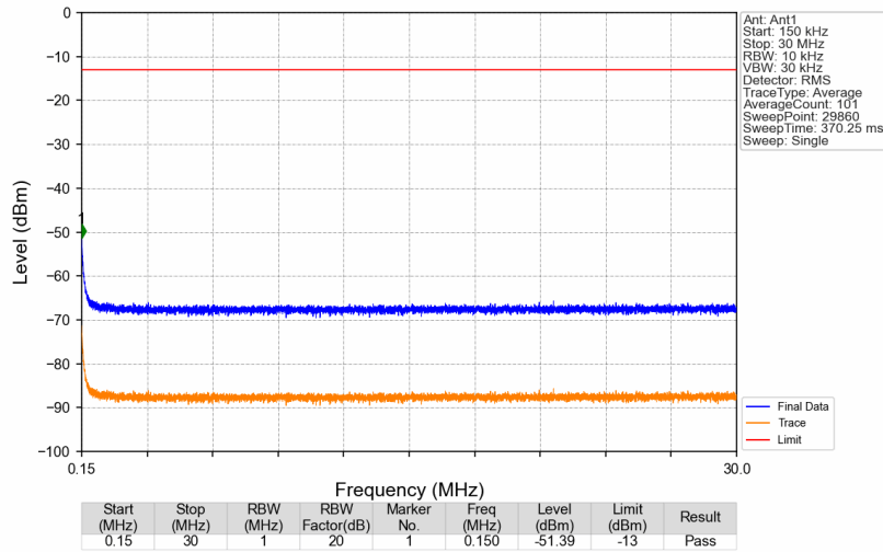
3780MHz-3980MHz_3780.1MHz_GMSK_SISO_Ant1_NTNV
