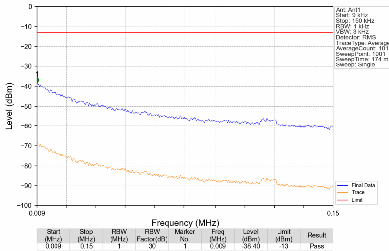
3780MHz-3980MHz_3780.1MHz_GMSK_SISO_Ant1_NTNV
