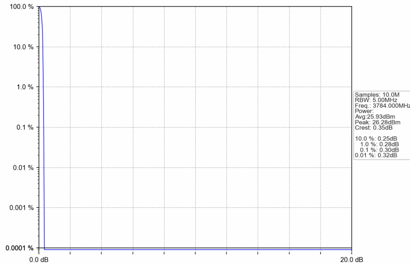
3780MHz-3980MHz_3784MHz_GMSK_SISO_Ant1_NTNV_AGC+3
