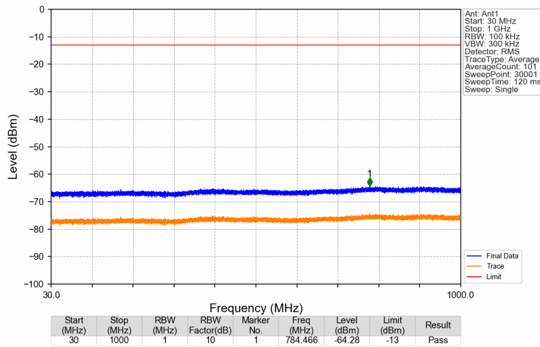
3700MHz-3900MHz_3700.1MHz_GMSK_SISO_Ant1_NTNV
