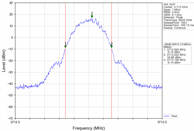
3700MHz-3900MHz_3713MHz_GMSK_SISO_Ant1_NTNV_AGC
