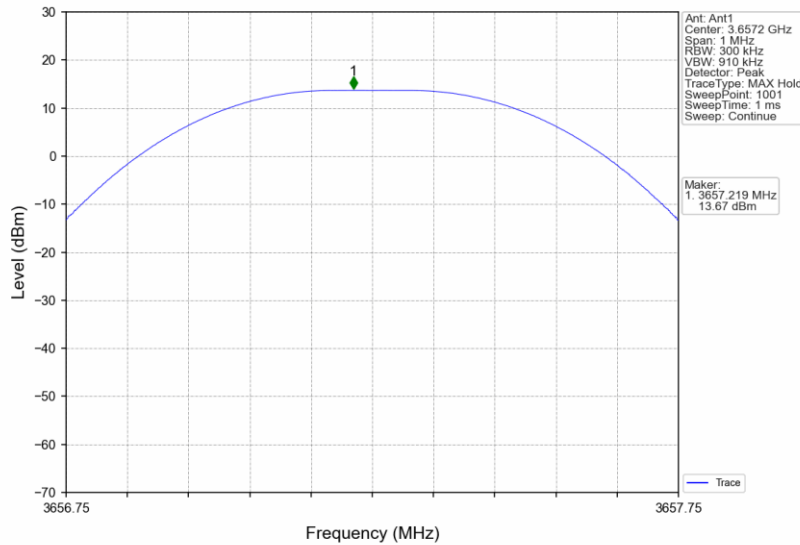
Band48_3657.25MHz_GMSK_SISO_Ant1_NTNV_AGC+3
