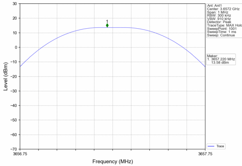
Band48_3657.25MHz_GMSK_SISO_Ant1_NTNV_AGC+3
