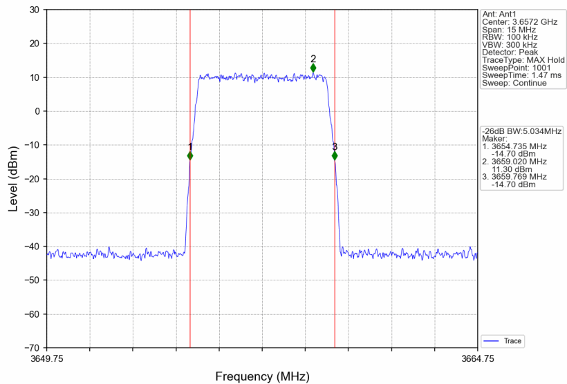
3550MHz-3700MHz_3657.25MHz_AWGN_SISO_Ant1_NTNV_AGC
