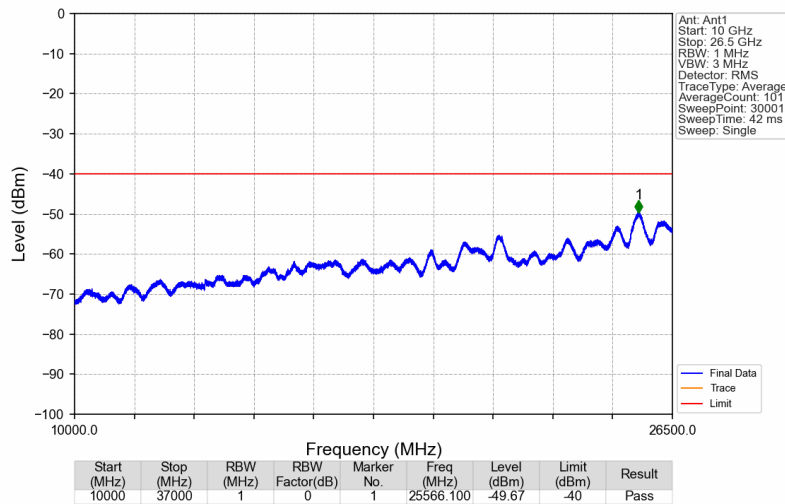
3550MHz-3700MHz_3625MHz_GMSK_SISO_Ant1_NTNV
