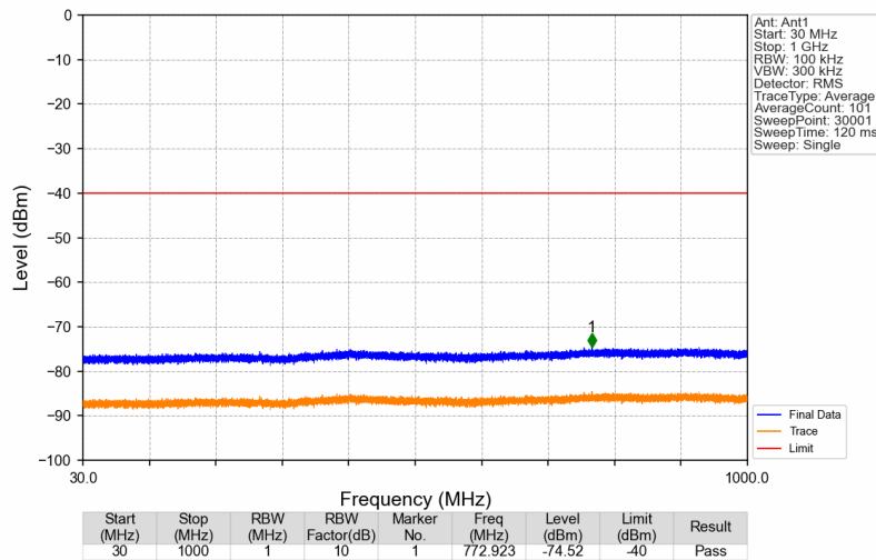
3550MHz-3700MHz_3550.1MHz_GMSK_SISO_Ant1_NTNV
