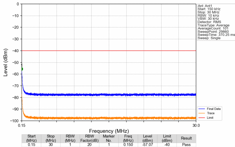
3550MHz-3700MHz_3550.1MHz_GMSK_SISO_Ant1_NTNV
