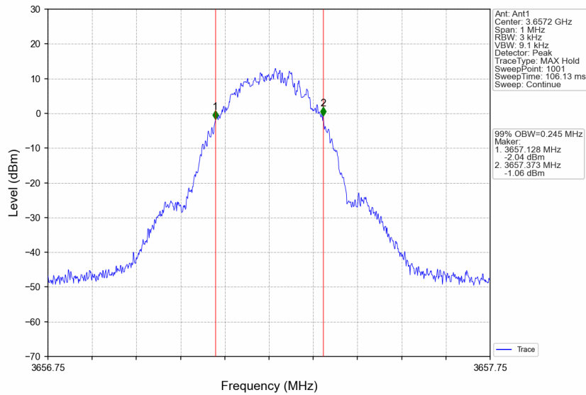
3550MHz-3700MHz_3657.25MHz_GMSK_SISO_Ant1_NTNV_AGC+3
