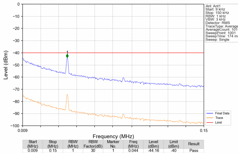
3550MHz-3700MHz_3550.1MHz_GMSK_SISO_Ant1_NTNV
