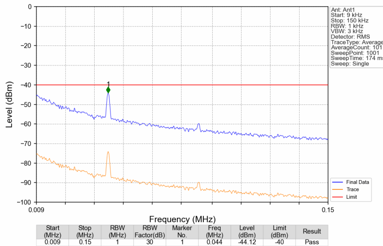
3550MHz-3700MHz_3699.9MHz_GMSK_SISO_Ant1_NTNV
