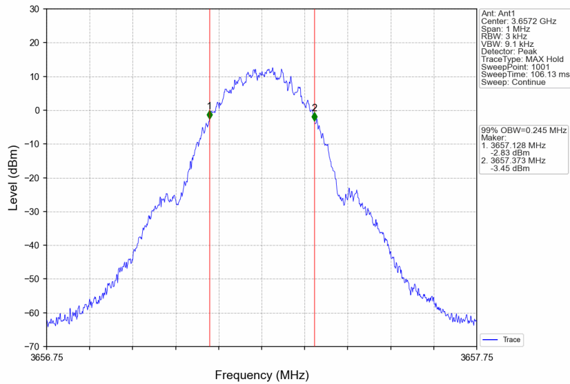
3550MHz-3700MHz_3657.25MHz_GMSK_SISO_Ant1_NTNV_AGC
