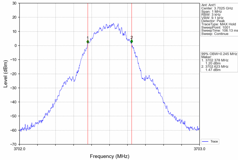
3700MHz-3800MHz_3702.5MHz_GMSK_SISO_Ant1_NTNV_AGC
