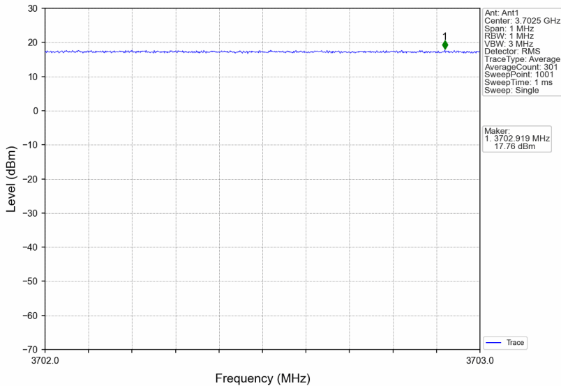
3700MHz-3800MHz_3702.5MHz_GMSK_SISO_Ant1_NTNV_AGC+3
