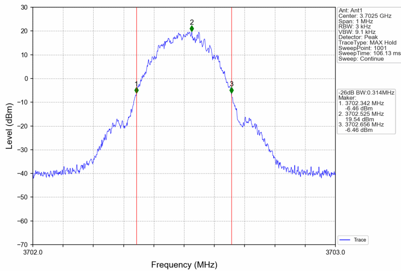
3700MHz-3800MHz_3702.5MHz_GMSK_SISO_Ant1_NTNV_AGC+3
