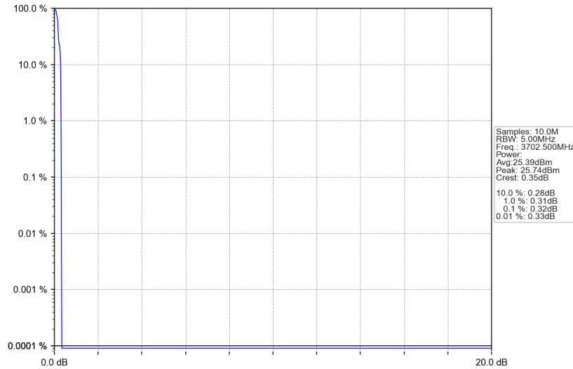
3700MHz-3800MHz_3702.5MHz_GMSK_SISO_Ant1_NTNV_AGC+3
