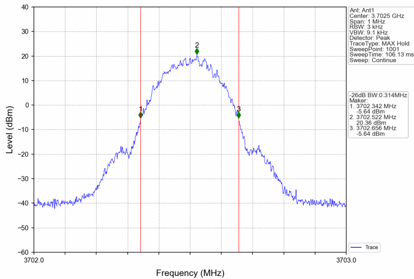
3700MHz-3800MHz_3702.5MHz_GMSK_SISO_Ant1_NTNV_AGC
