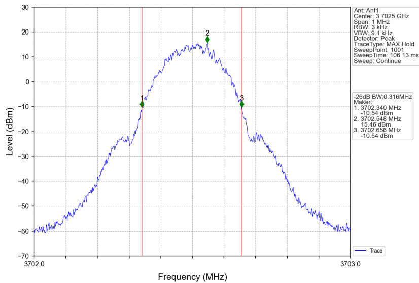
3700MHz-3800MHz_3702.5MHz_GMSK_SISO_Ant1_NTNV_AGC+3
