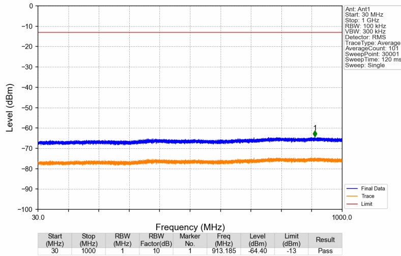
3700MHz-3800MHz_3702.5MHz_AWGN_SISO_Ant1_NTNV
