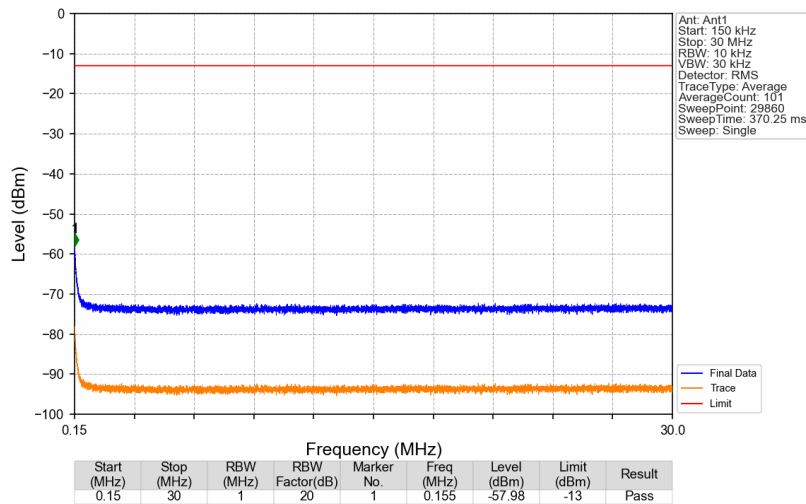
3700MHz-3800MHz_3750MHz_AWGN_SISO_Ant1_NTNV
