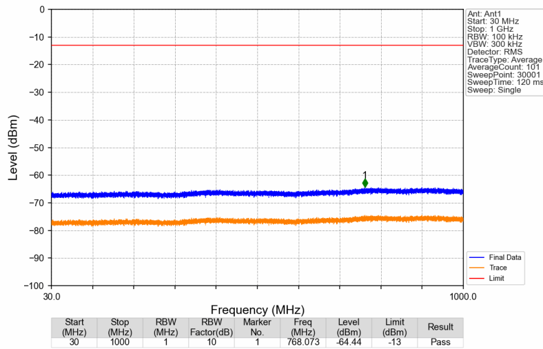
3700MHz-3800MHz_3700.1MHz_GMSK_SISO_Ant1_NTNV
