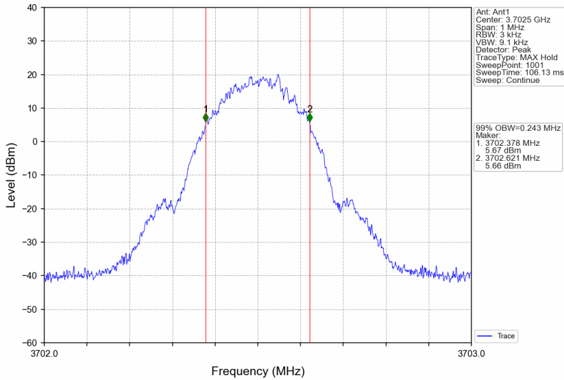
3700MHz-3800MHz_3702.5MHz_GMSK_SISO_Ant1_NTNV_AGC+3
