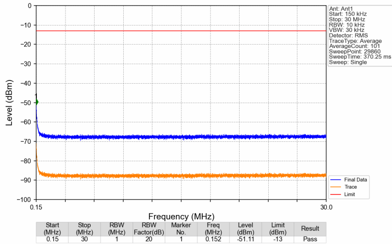
3700MHz-3800MHz_3700.1MHz_GMSK_SISO_Ant1_NTNV
