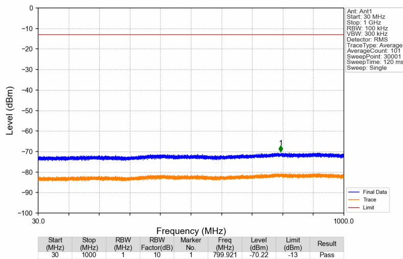
3700MHz-3800MHz_3750MHz_AWGN_SISO_Ant1_NTNV
