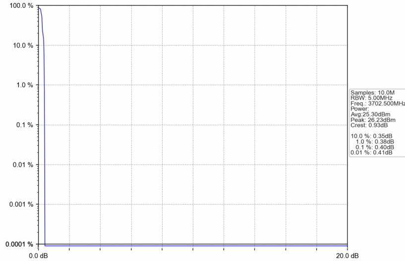
3700MHz-3800MHz_3702.5MHz_GMSK_SISO_Ant1_NTNV_AGC
