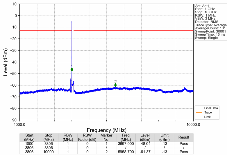
3700MHz-3800MHz_3702.5MHz_AWGN_SISO_Ant1_NTNV
