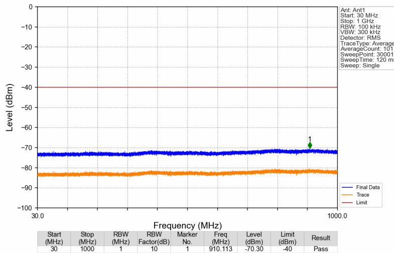
3450MHz-3550MHz_3549.9MHz_GMSK_SISO_Ant1_NTNV
