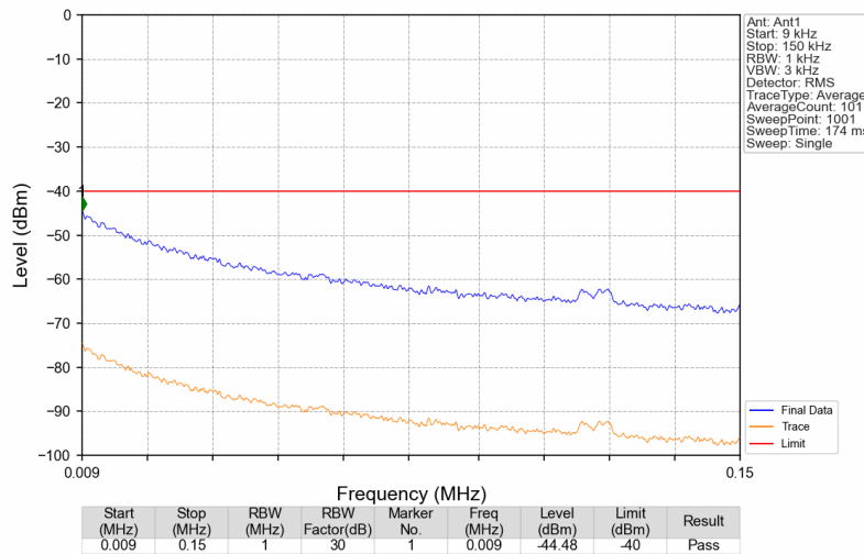
3450MHz-3550MHz_3450.1MHz_GMSK_SISO_Ant1_NTNV
