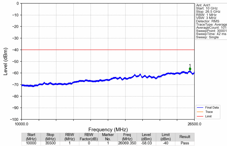
3450MHz-3550MHz_3500MHz_GMSK_SISO_Ant1_NTNV
