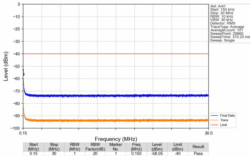
3450MHz-3550MHz_3549.9MHz_GMSK_SISO_Ant1_NTNV
