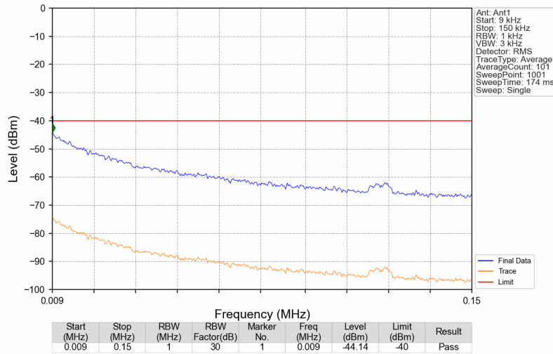
3450MHz-3550MHz_3500MHz_GMSK_SISO_Ant1_NTNV
