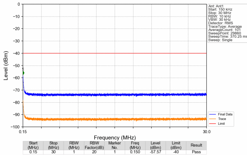
3450MHz-3550MHz_3500MHz_GMSK_SISO_Ant1_NTNV
