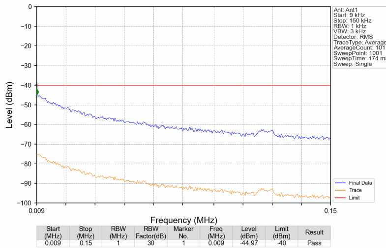
3450MHz-3550MHz_3549.9MHz_GMSK_SISO_Ant1_NTNV
