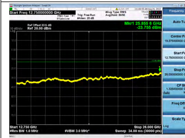
QPSK - 12.75GHz~26GHz
