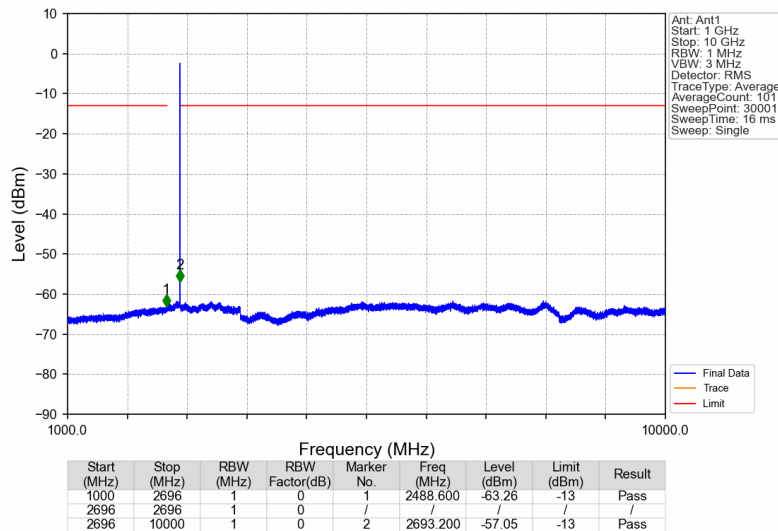
Band41_2689.9MHz_GMSK_SISO_Ant1_NTNV
