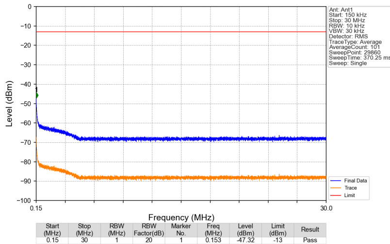
Band41_2687.5MHz_AWGN_SISO_Ant1_NTNV
