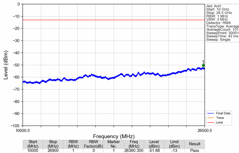
Band41_2689.9MHz_GMSK_SISO_Ant1_NTNV
