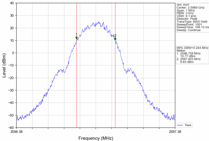
Band41_2596.88MHz_GMSK_SISO_Ant1_NTNV_AGC
