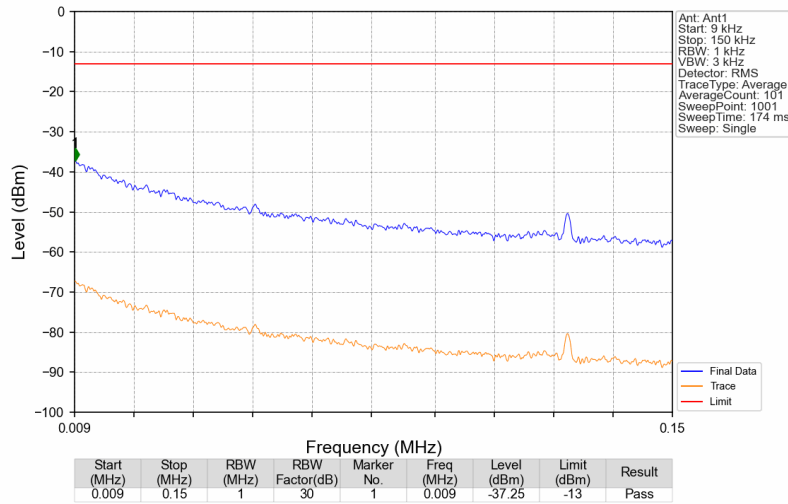
Band41_2687.5MHz_AWGN_SISO_Ant1_NTNV
