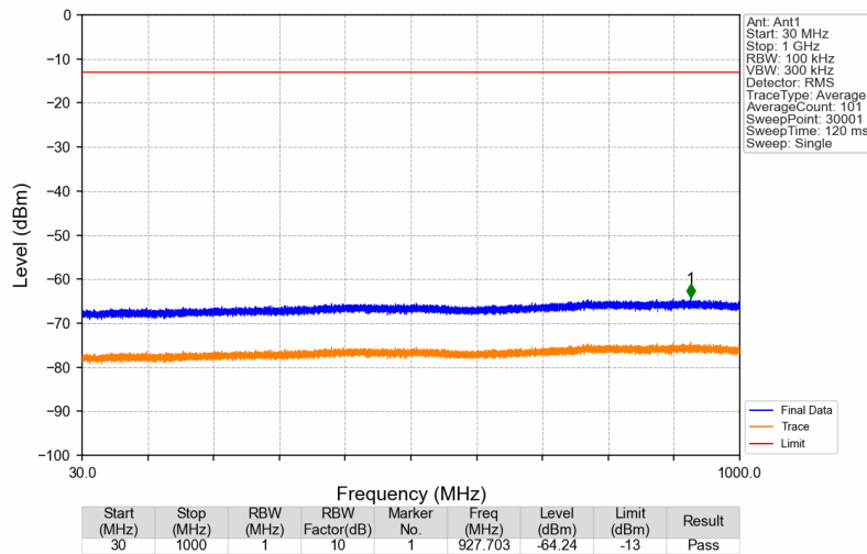
Band41_2496.1MHz_GMSK_SISO_Ant1_NTNV
