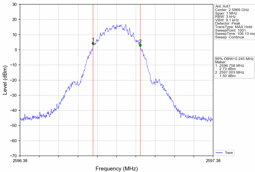
Band41_2596.88MHz_GMSK_SISO_Ant1_NTNV_AGC+3
