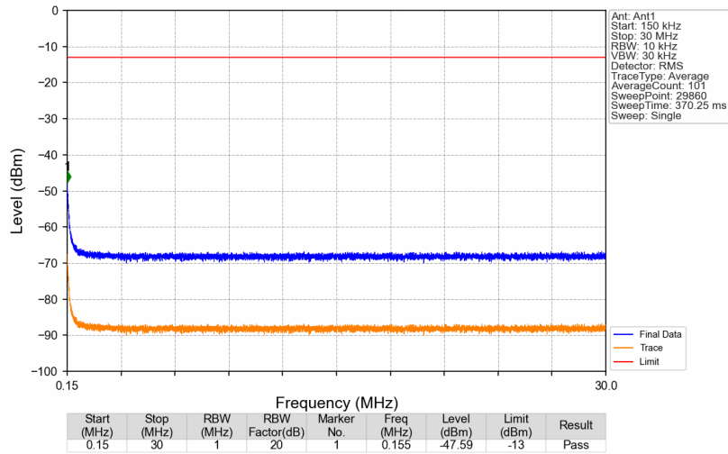
Band41_2689.9MHz_GMSK_SISO_Ant1_NTNV
