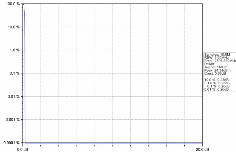
Band41_2596.88MHz_GMSK_SISO_Ant1_NTNV_AGC
