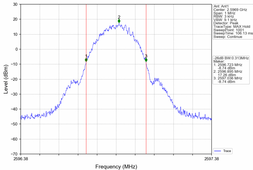
Band41_2596.88MHz_GMSK_SISO_Ant1_NTNV_AGC+3
