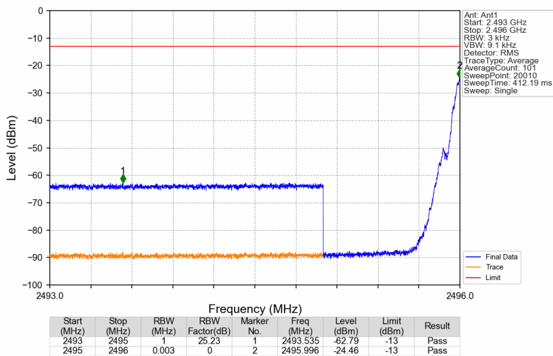
Band41_2496.1MHz_GMSK_SISO_Ant1_NTNV_AGC+3
