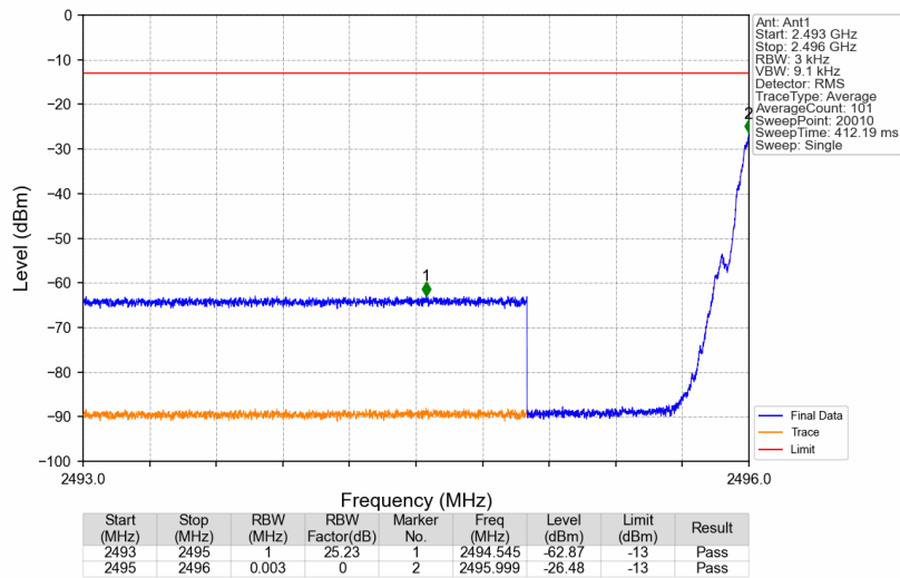
Band41_2496.1MHz_GMSK_SISO_Ant1_NTNV_AGC
