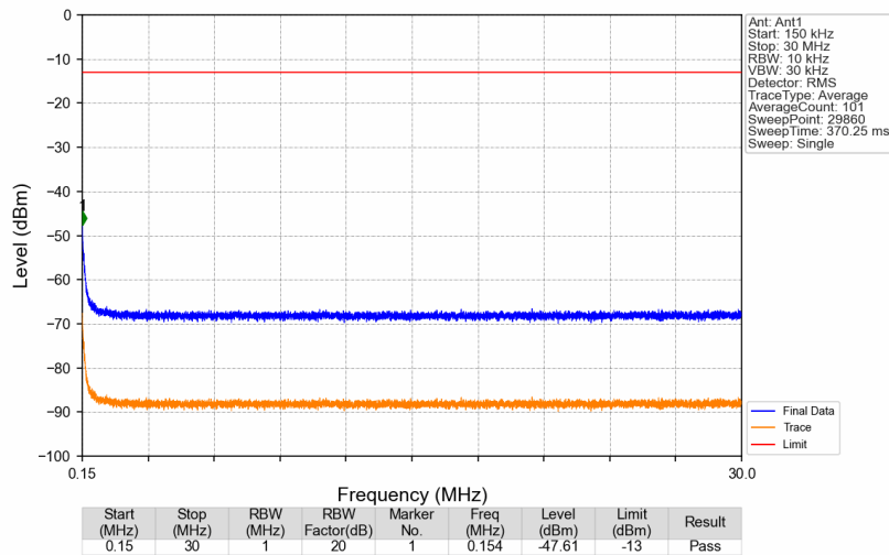
Band41_2496.1MHz_GMSK_SISO_Ant1_NTNV
