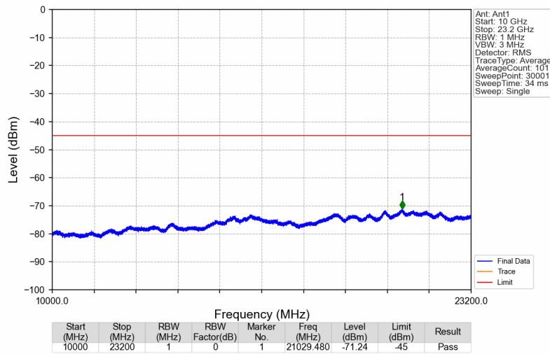
Band30_2359.9MHz_GMSK_SISO_Ant1_NTNV
