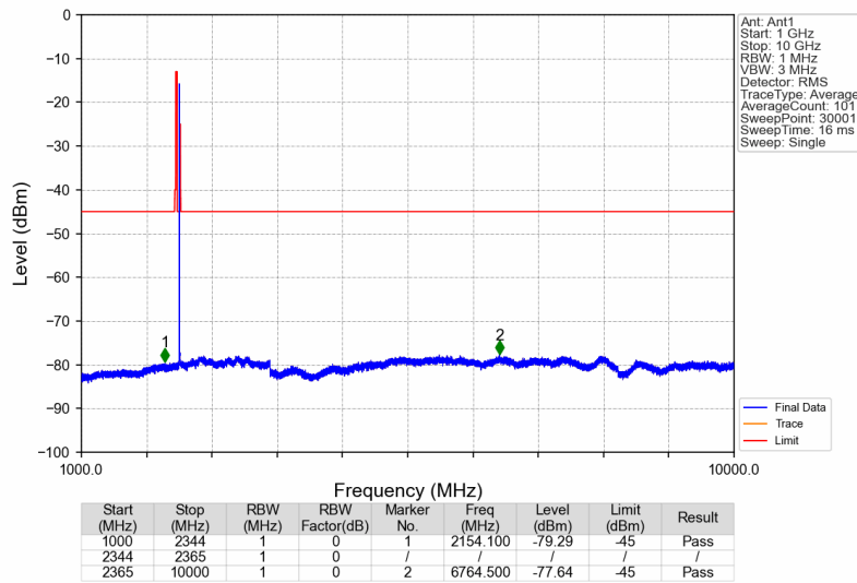
Band30_2350.1MHz_GMSK_SISO_Ant1_NTNV
