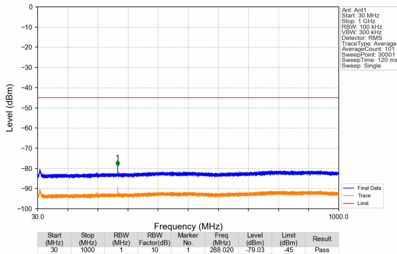
Band30_2359.9MHz_GMSK_SISO_Ant1_NTNV
