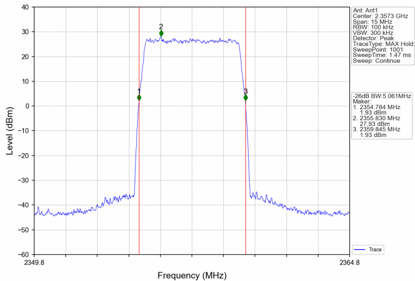
Band30_2357.3MHz_AWGN_SISO_Ant1_NTNV_AGC
