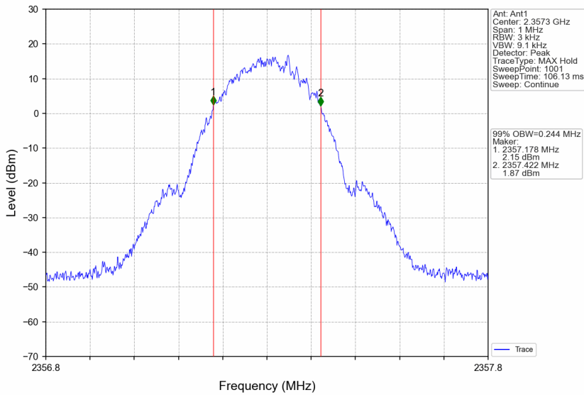
Band30_2357.3MHz_GMSK_SISO_Ant1_NTNV_AGC+3
