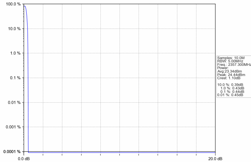
Band30_2357.3MHz_GMSK_SISO_Ant1_NTNV_AGC
