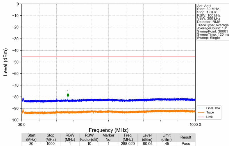
Band30_2352.5MHz_AWGN_SISO_Ant1_NTNV
