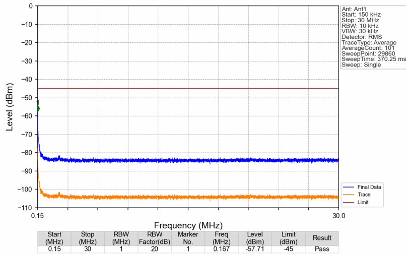
Band30_2359.9MHz_GMSK_SISO_Ant1_NTNV
