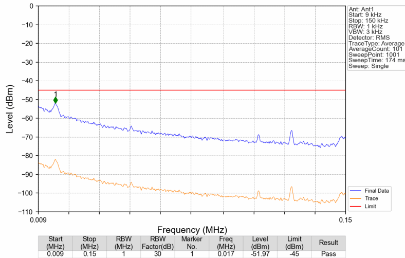
Band30_2357.5MHz_AWGN_SISO_Ant1_NTNV
