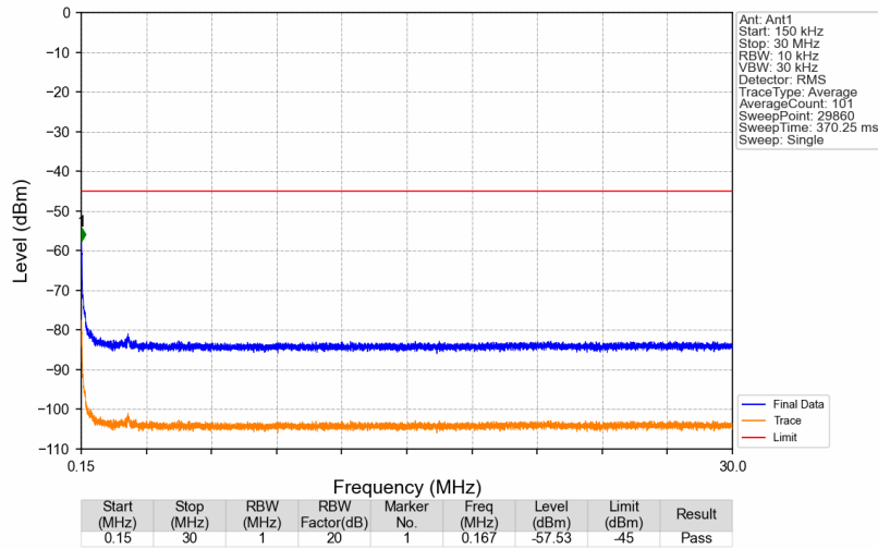
Band30_2350.1MHz_GMSK_SISO_Ant1_NTNV
