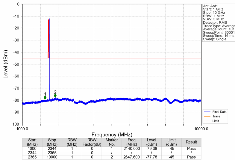
Band30_2359.9MHz_GMSK_SISO_Ant1_NTNV
