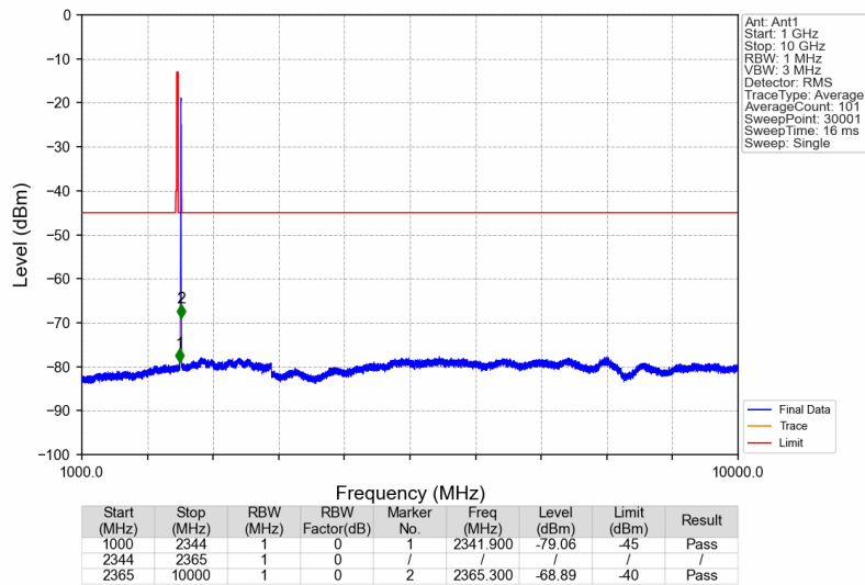
Band30_2357.5MHz_AWGN_SISO_Ant1_NTNV
