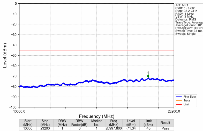
Band30_2350.1MHz_GMSK_SISO_Ant1_NTNV
