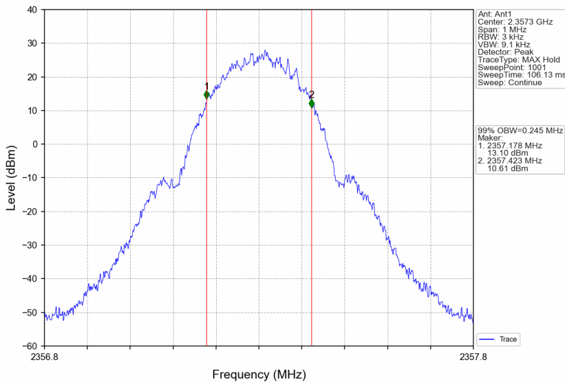
Band30_2357.3MHz_GMSK_SISO_Ant1_NTNV_AGC
