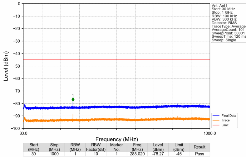
Band30_2350.1MHz_GMSK_SISO_Ant1_NTNV
