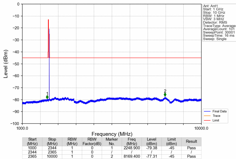
Band30_2352.5MHz_AWGN_SISO_Ant1_NTNV
