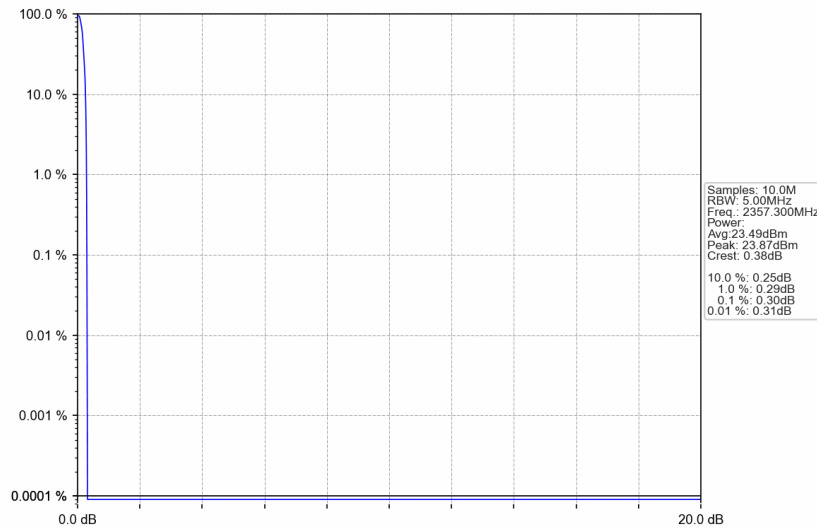
Band30_2357.3MHz_GMSK_SISO_Ant1_NTNV_AGC+3
