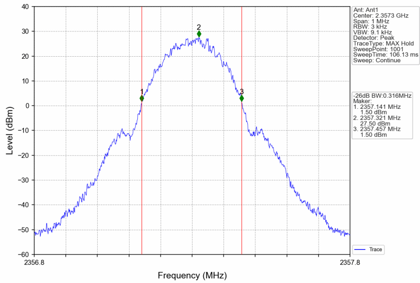
Band30_2357.3MHz_GMSK_SISO_Ant1_NTNV_AGC
