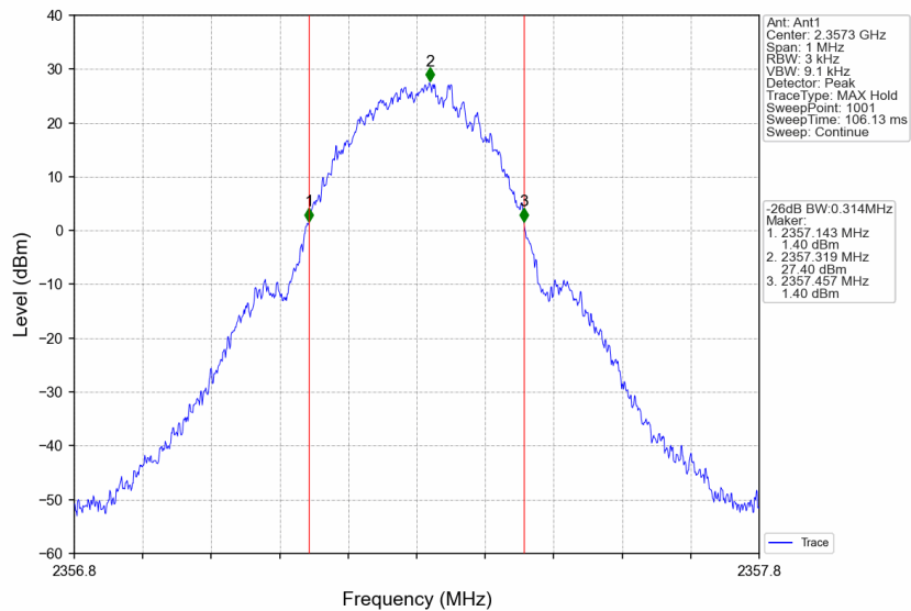
Band30_2357.3MHz_GMSK_SISO_Ant1_NTNV_AGC
