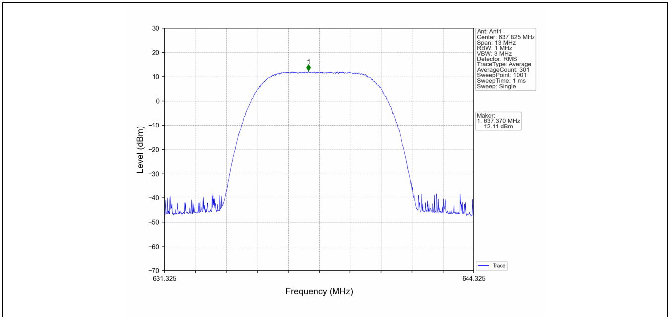
Band71_637.825MHz_GMSK_SISO_Ant1_NTNV_AGC
