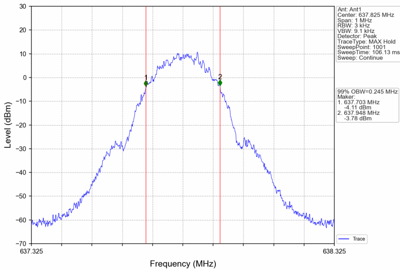
Band71_637.825MHz_GMSK_SISO_Ant1_NTNV_AGC+3
