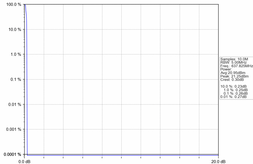
Band71_637.825MHz_GMSK_SISO_Ant1_NTNV_AGC+3
