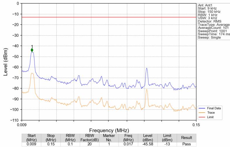
Band71_649.5MHz_AWGN_SISO_Ant1_NTNV
