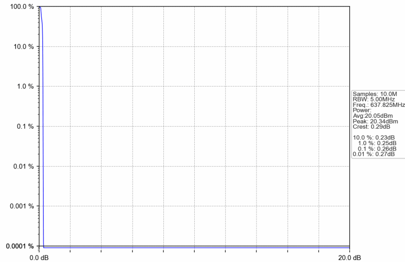
Band71_637.825MHz_GMSK_SISO_Ant1_NTNV_AGC
