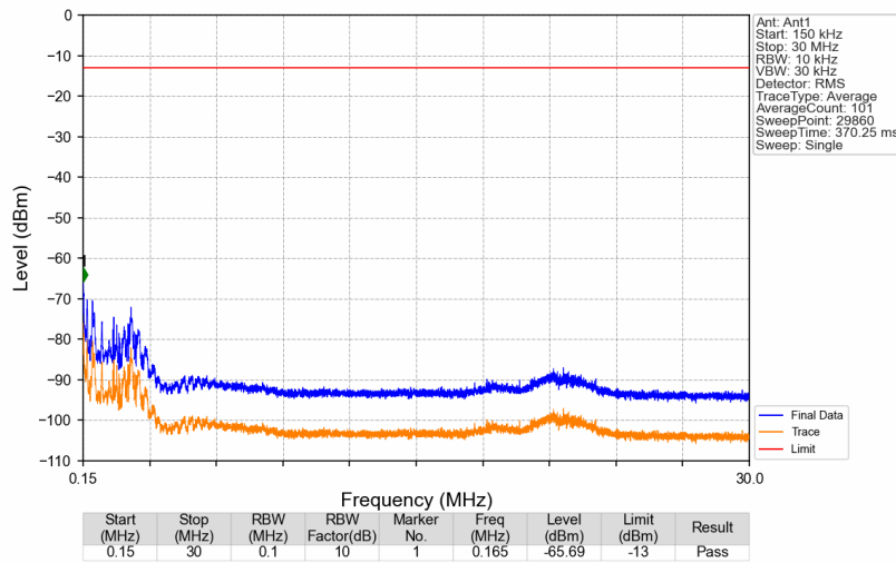
Band71_651.9MHz_GMSK_SISO_Ant1_NTNV
