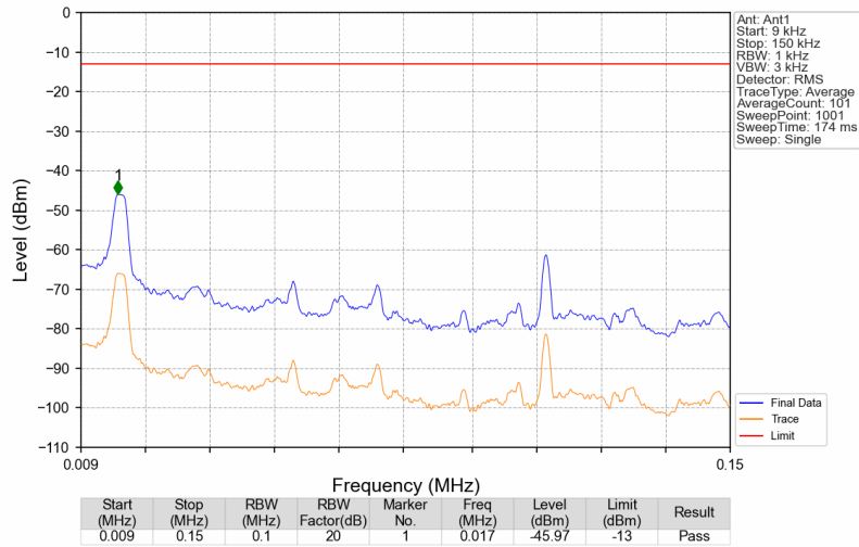
Band71_651.9MHz_GMSK_SISO_Ant1_NTNV
