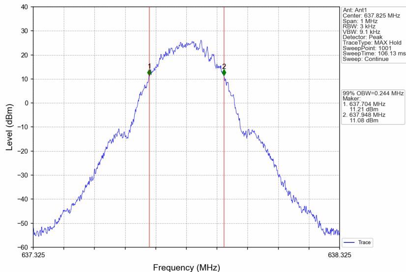
Band71_637.825MHz_GMSK_SISO_Ant1_NTNV_AGC
