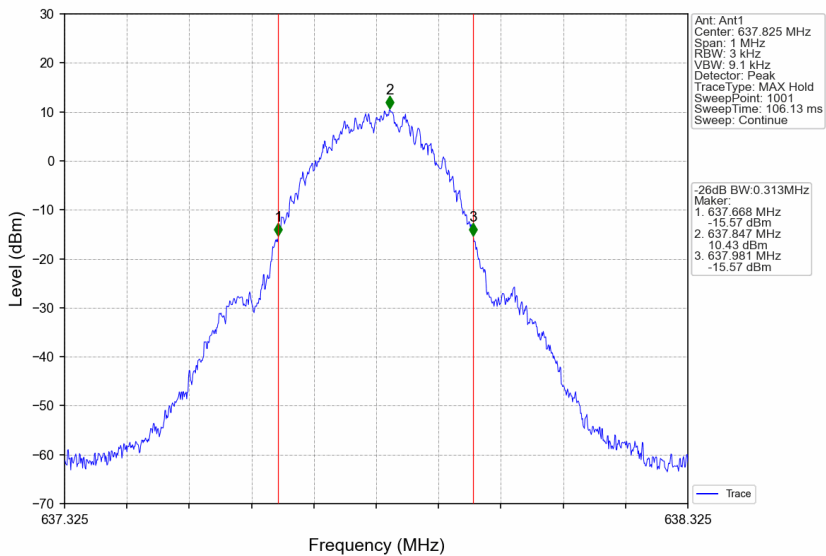
Band71_637.825MHz_GMSK_SISO_Ant1_NTNV_AGC+3
