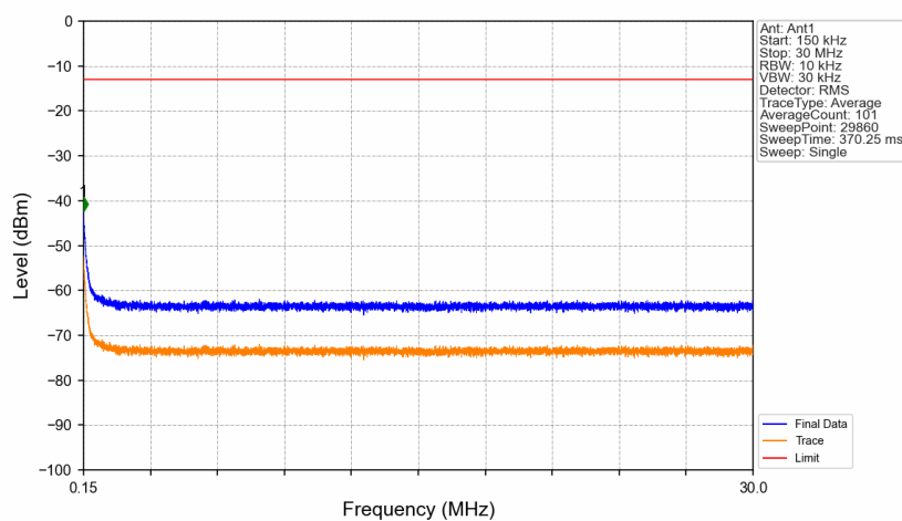
Band14_758.1MHz_GMSK_SISO_Ant1_NTNV
