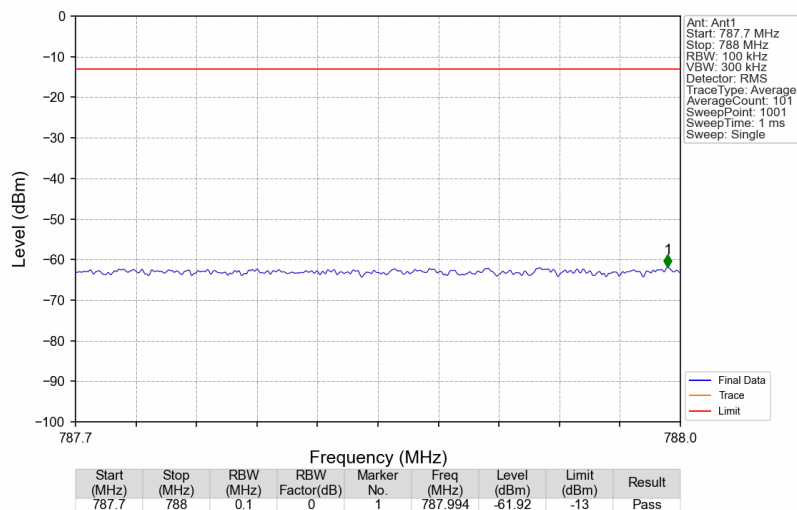
Band14_758.1MHz_GMSK_SISO_Ant1_NTNV_AGC
