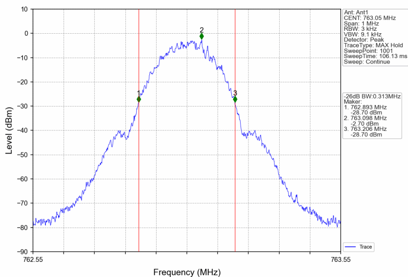
Band14_763.05MHz_GMSK_SISO_Ant1_NTNV_Input_AGC+3
