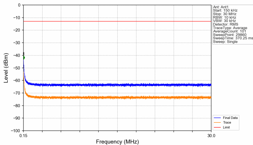
Band14_763MHz_GMSK_SISO_Ant1_NTNV
