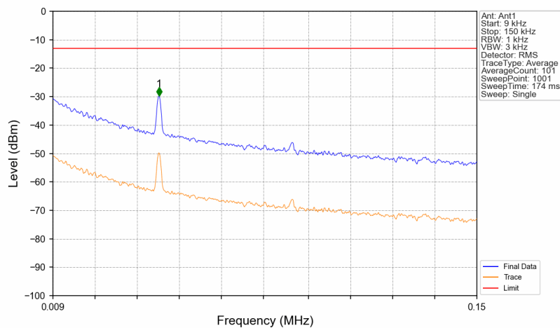
Band14_758.1MHz_GMSK_SISO_Ant1_NTNV
