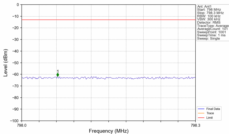
Band14_767.9MHz_GMSK_SISO_Ant1_NTNV_AGC+3
