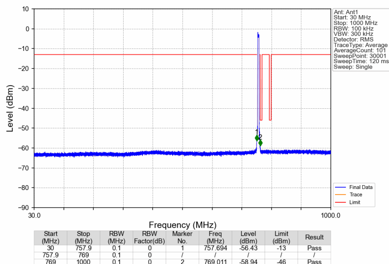
Band14_763MHz_AWGN_SISO_Ant1_NTNV
