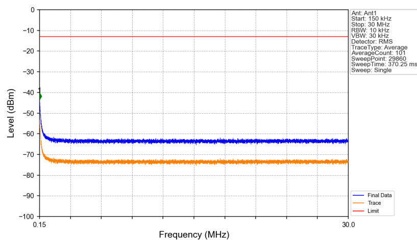
Band14_763MHz_AWGN_SISO_Ant1_NTNV
