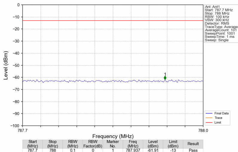
Band14_758.1MHz_GMSK_SISO_Ant1_NTNV_AGC+3
