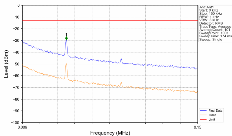
Band14_763MHz_AWGN_SISO_Ant1_NTNV
