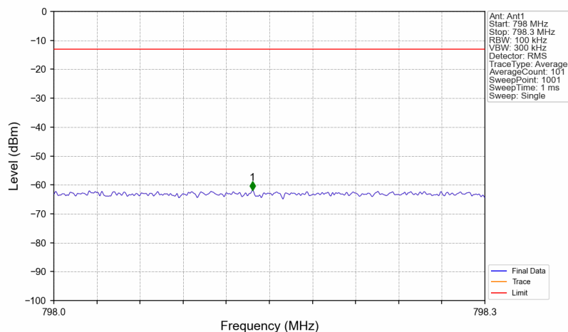
Band14_767.9MHz_GMSK_SISO_Ant1_NTNV_AGC
