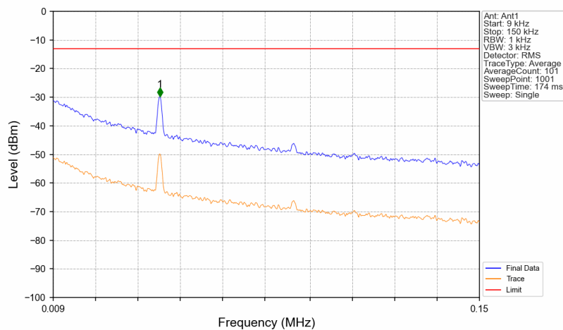
Band14_763MHz_GMSK_SISO_Ant1_NTNV
