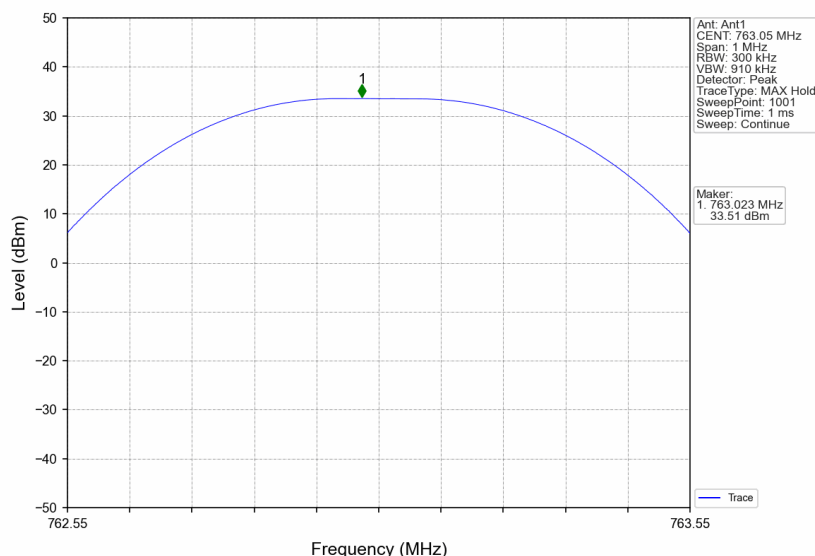
Band14_763.05MHz_GMSK_SISO_Ant1_NTNV_AGC+3
