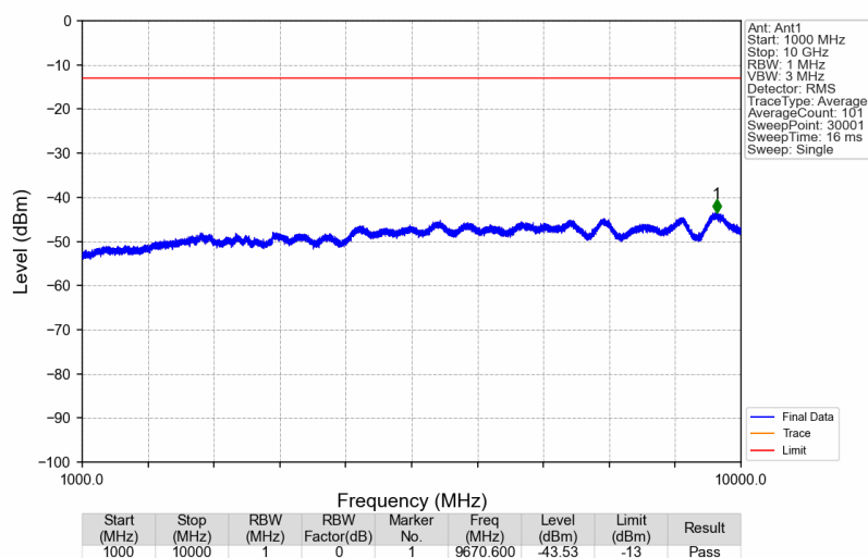
Band14_767.9MHz_GMSK_SISO_Ant1_NTNV
