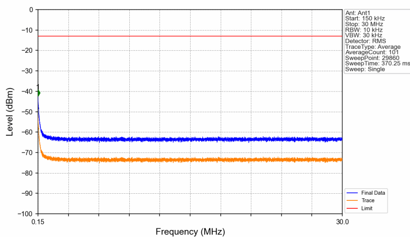
Band14_767.9MHz_GMSK_SISO_Ant1_NTNV
