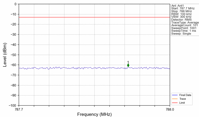
Band14_758.1MHz_GMSK_SISO_Ant1_NTNV_AGC+3
