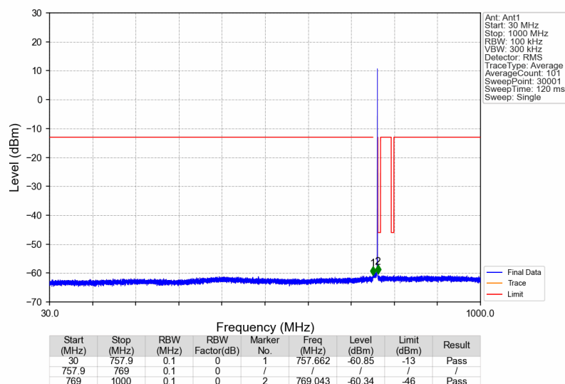
Band14_767.9MHz_GMSK_SISO_Ant1_NTNV
