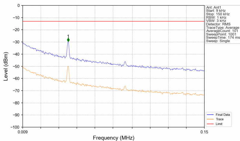
Band14_767.9MHz_GMSK_SISO_Ant1_NTNV
