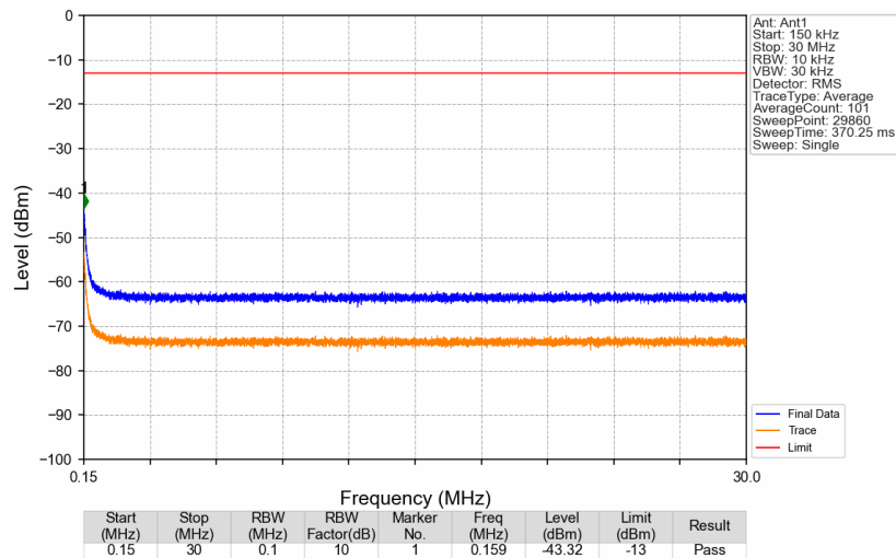
Band71_634.5MHz_GMSK_SISO_Ant1_NTNV
