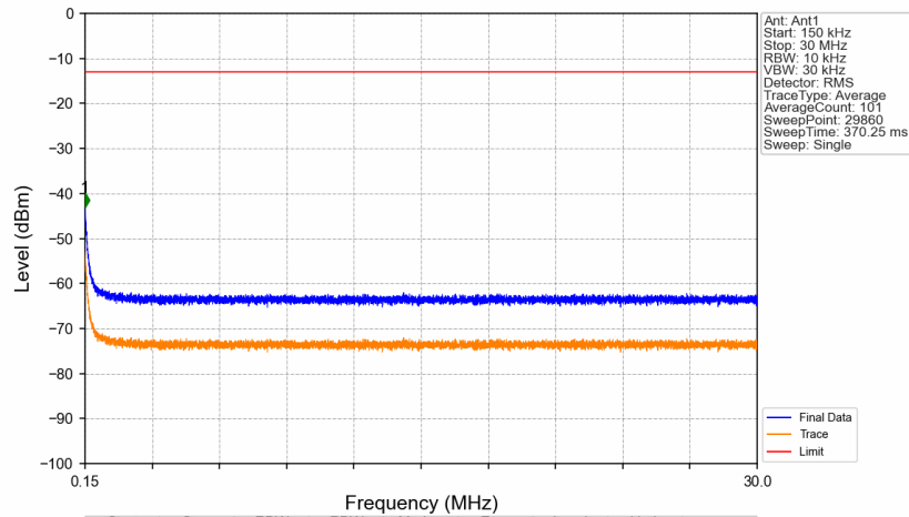
Band71_649.5MHz_AWGN_SISO_Ant1_NTNV
