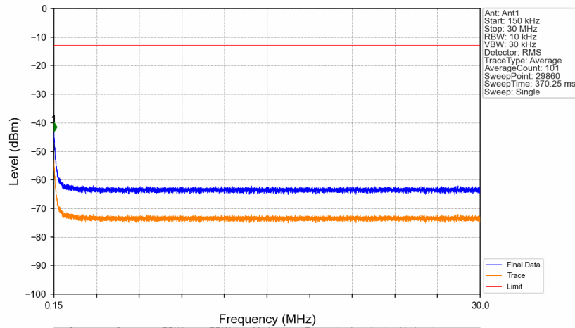
Band71_651.9MHz_GMSK_SISO_Ant1_NTNV
