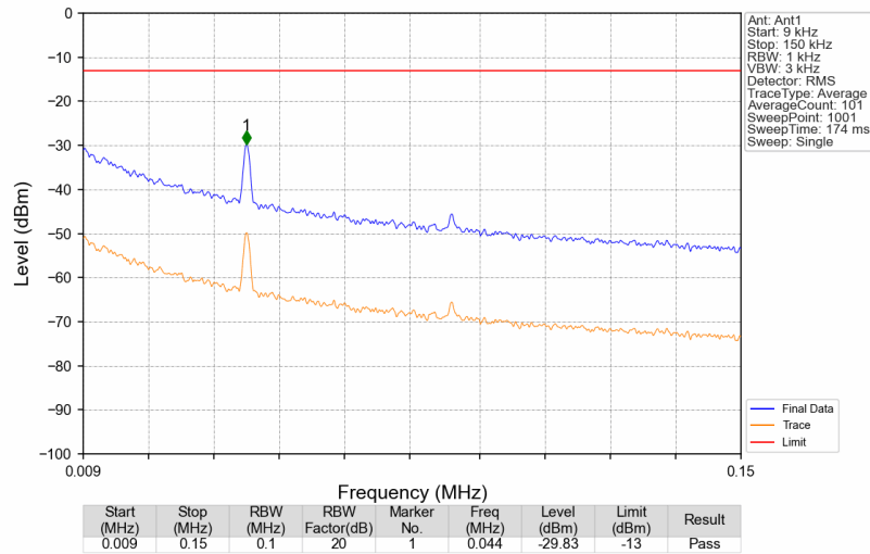
Band71_634.5MHz_GMSK_SISO_Ant1_NTNV
