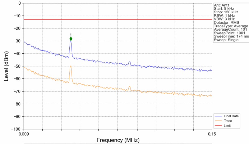
Band71_649.5MHz_AWGN_SISO_Ant1_NTNV
