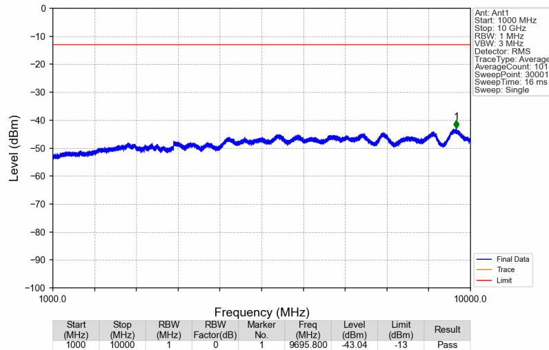
Band71_649.5MHz_AWGN_SISO_Ant1_NTNV
