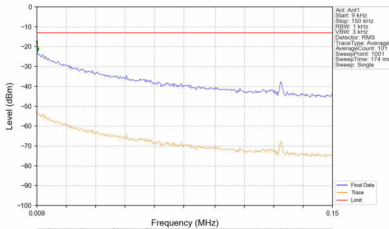
Band41_2689.9MHz_GMSK_SISO_Ant1_NTNV
