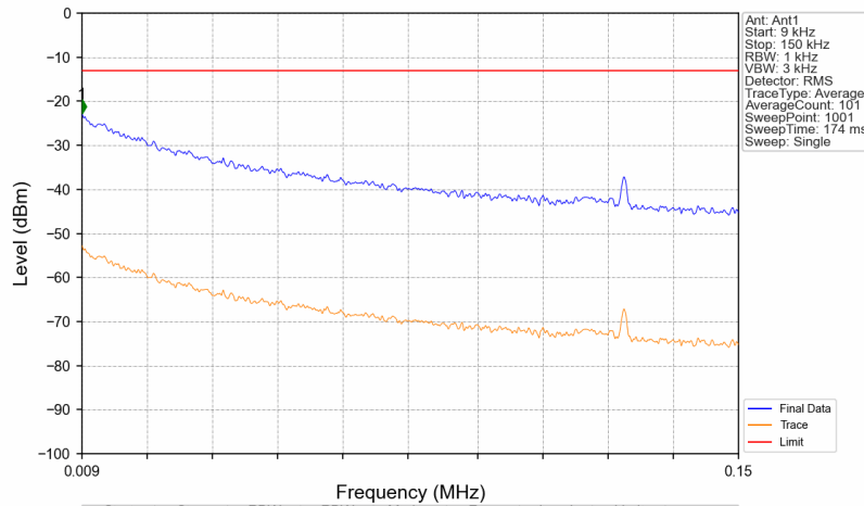
Band41_2496.1MHz_GMSK_SISO_Ant1_NTNV
