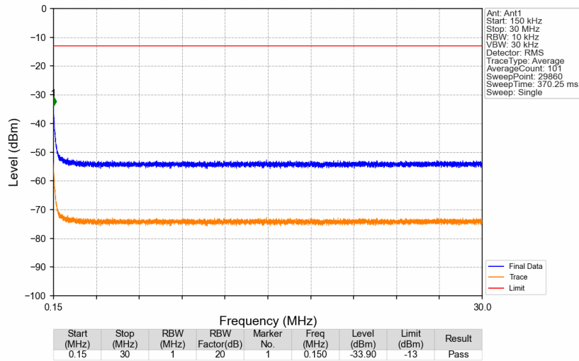
Band41_2689.9MHz_GMSK_SISO_Ant1_NTNV
