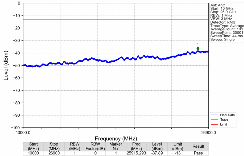
Band41_2498.5MHz_AWGN_SISO_Ant1_NTNV
