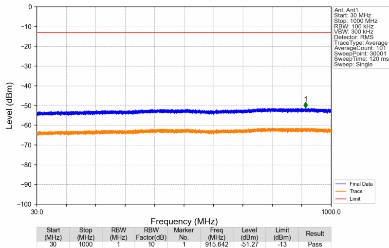
Band41_2689.9MHz_GMSK_SISO_Ant1_NTNV
