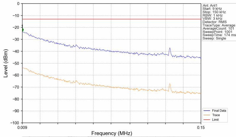
Band41_2687.5MHz_AWGN_SISO_Ant1_NTNV
