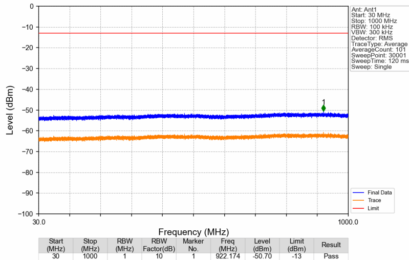
Band41_2496.1MHz_GMSK_SISO_Ant1_NTNV
