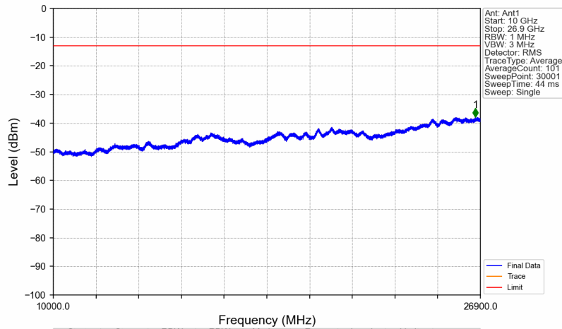
Band41_2593MHz_GMSK_SISO_Ant1_NTNV
