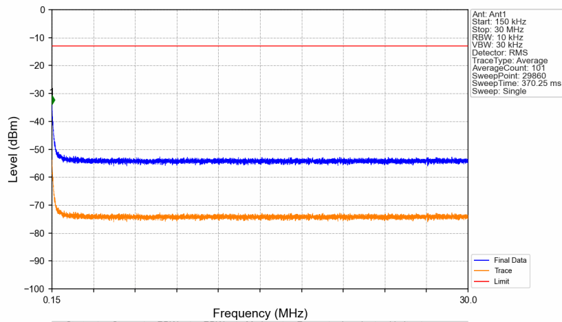
Band41_2687.5MHz_AWGN_SISO_Ant1_NTNV
