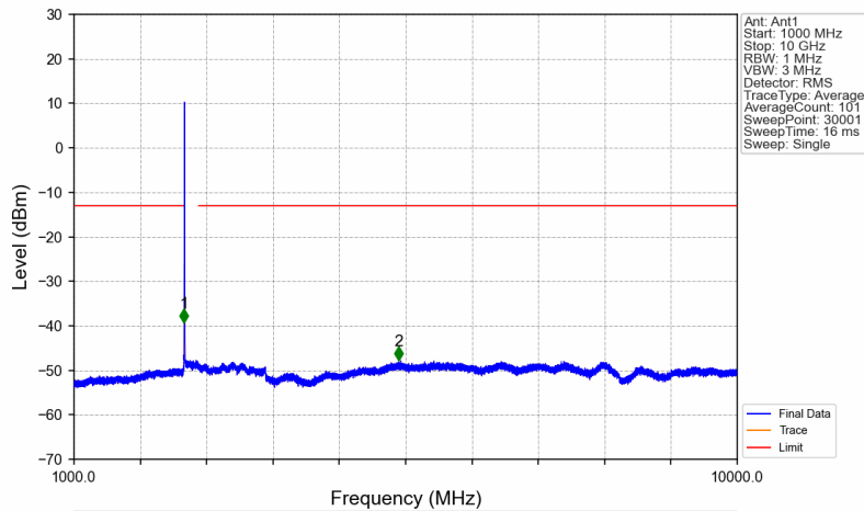
Band41_2498.5MHz_AWGN_SISO_Ant1_NTNV
