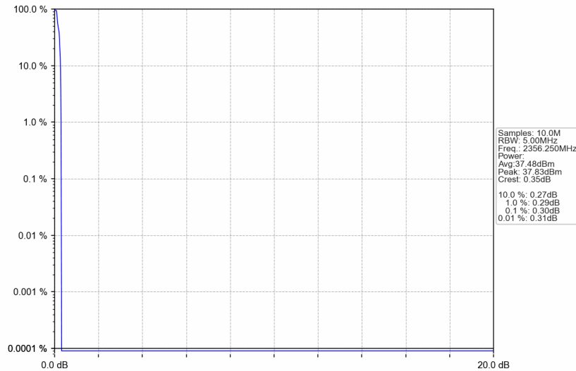
Band30_2356.25MHz_GMSK_SISO_Ant1_NTNV_AGC+3
