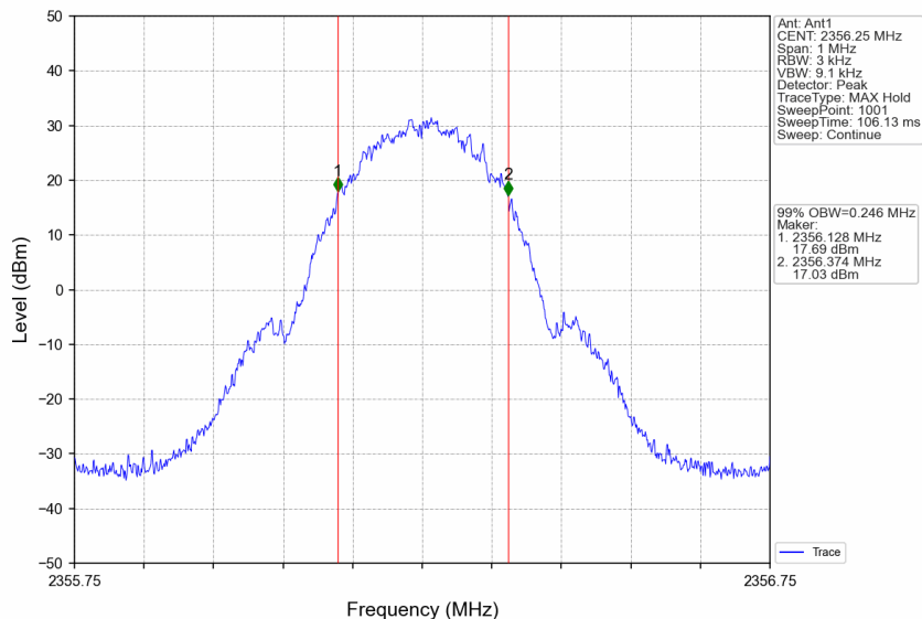
Band30_2356.25MHz_GMSK_SISO_Ant1_NTNV_Output_AGC+3
