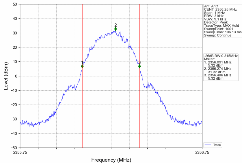
Band30_2356.25MHz_GMSK_SISO_Ant1_NTNV_Output_AGC+3
