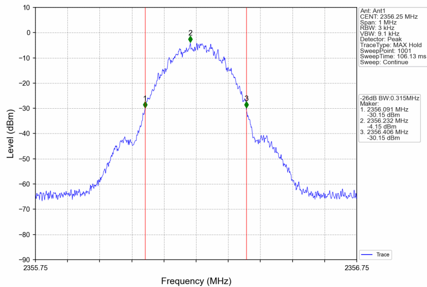
Band30_2356.25MHz_GMSK_SISO_Ant1_NTNV_Input_AGC+3
