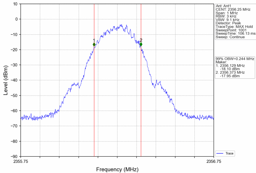
Band30_2356.25MHz_GMSK_SISO_Ant1_NTNV_Input_AGC+3
