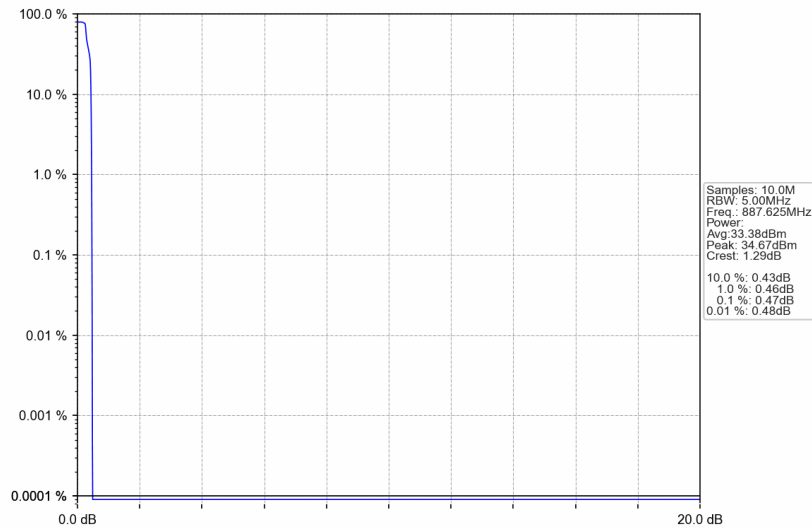
Band26b_887.625MHz_GMSK_SISO_Ant1_NTNV_AGC
