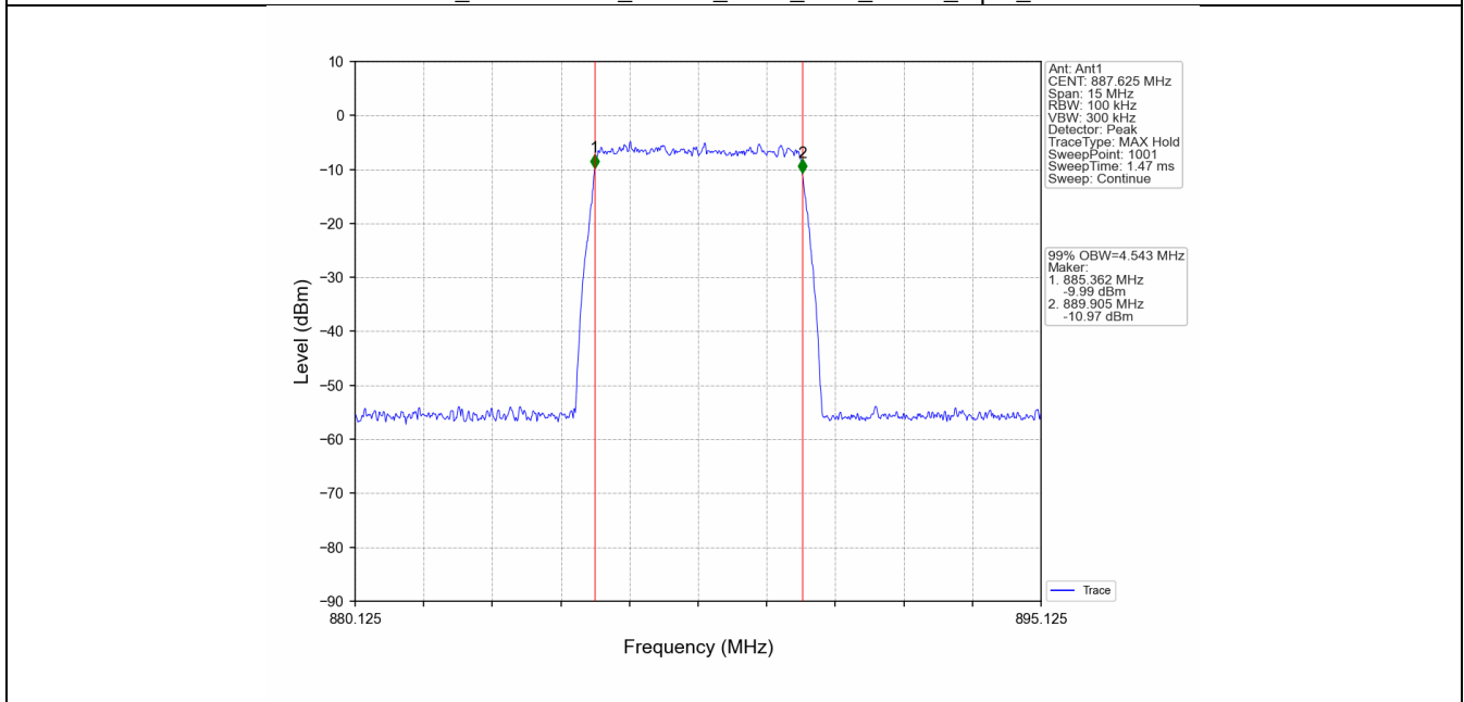
Band26b_887.625MHz_AWGN_SISO_Ant1_NTNV_Input_AGC+3
