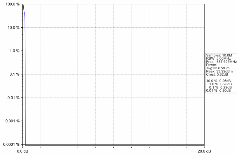
Band26b_887.625MHz_GMSK_SISO_Ant1_NTNV_AGC+3
