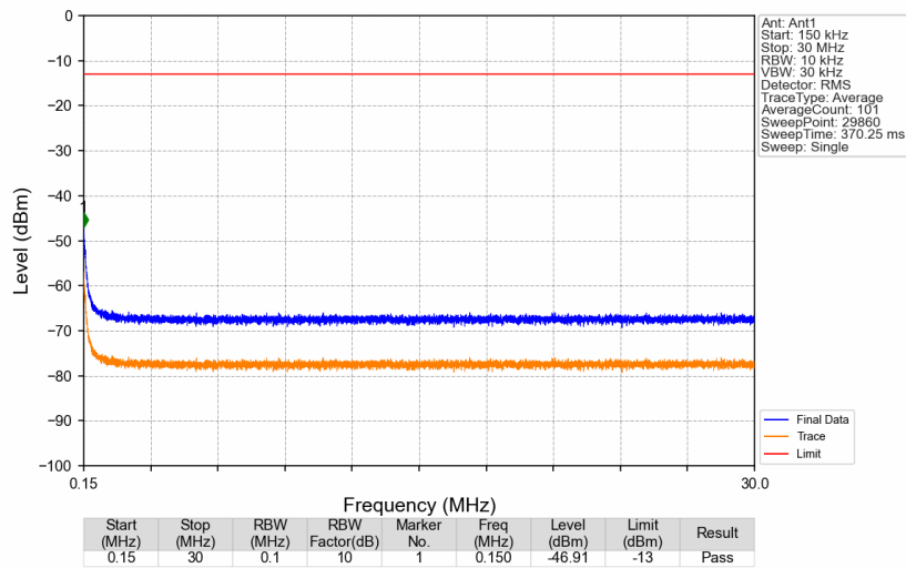
Band26b_891.5MHz_AWGN_SISO_Ant1_NTNV
