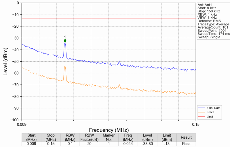
Band26b_881.5MHz_GMSK_SISO_Ant1_NTNV
