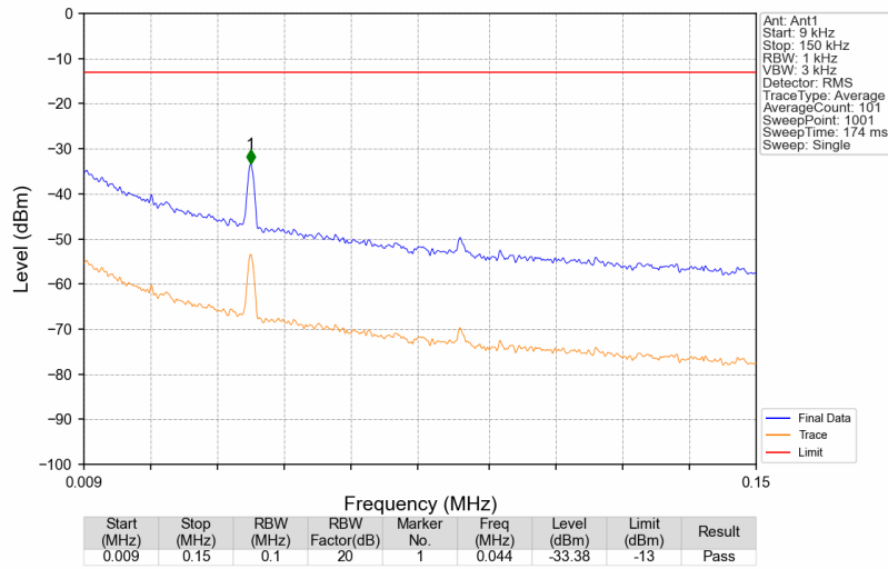
Band26b_891.5MHz_AWGN_SISO_Ant1_NTNV
