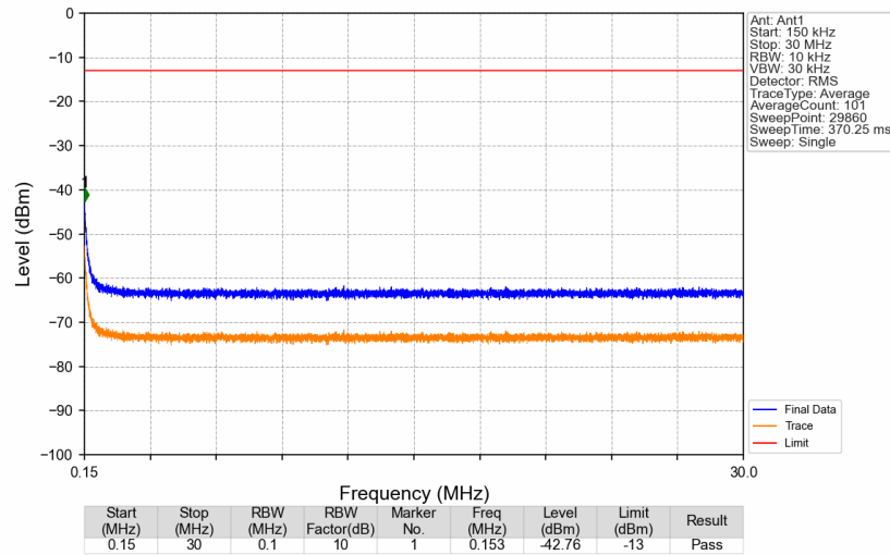
Band26b_869.1MHz_GMSK_SISO_Ant1_NTNV
