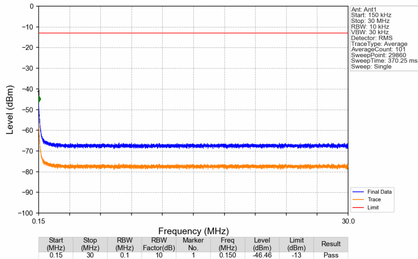
Band26b_893.9MHz_GMSK_SISO_Ant1_NTNV
