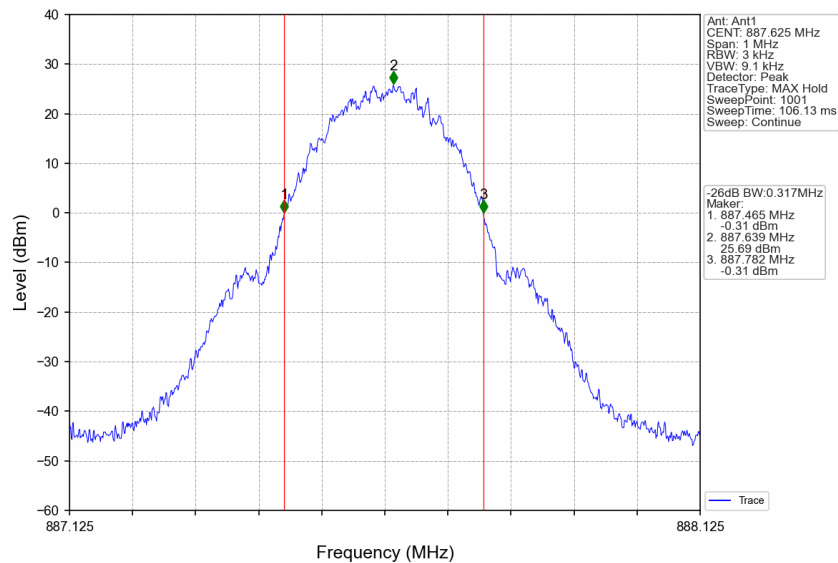
Band26b_887.625MHz_GMSK_SISO_Ant1_NTNV_Output_AGC+3
