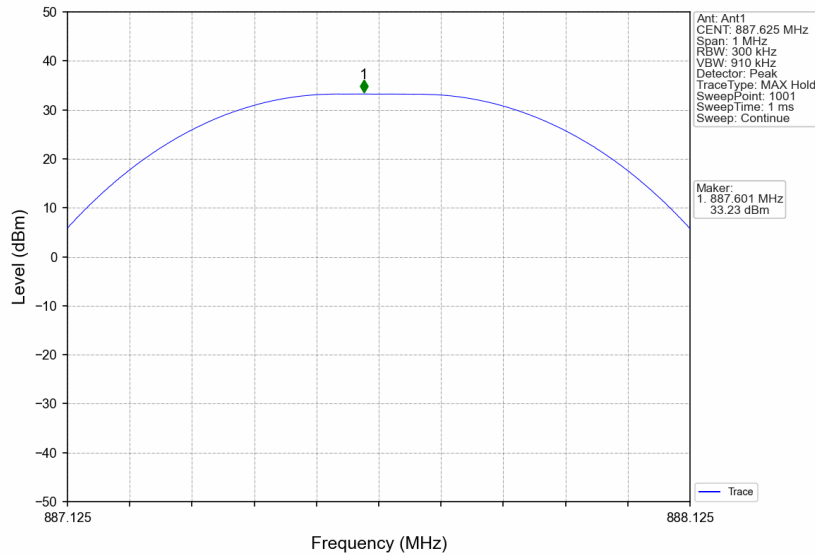
Band26b_887.625MHz_GMSK_SISO_Ant1_NTNV_AGC+3
