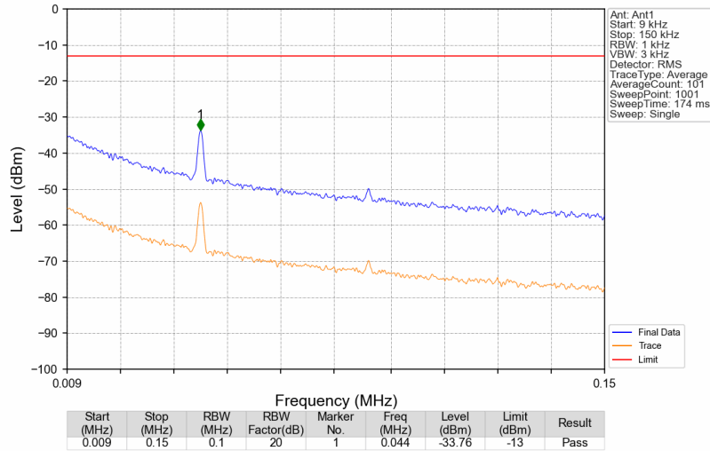
Band26b_893.9MHz_GMSK_SISO_Ant1_NTNV
