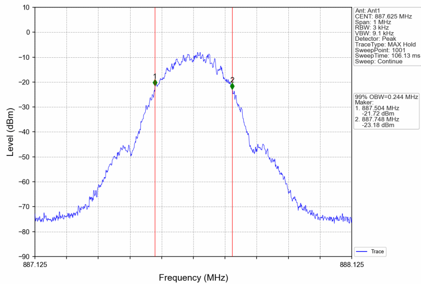
Band26b_887.625MHz_GMSK_SISO_Ant1_NTNV_Input_AGC+3
