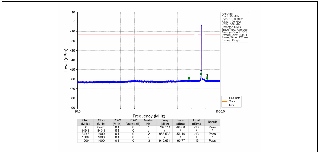
Band26b_871.5MHz_AWGN_SISO_Ant1_NTNV
