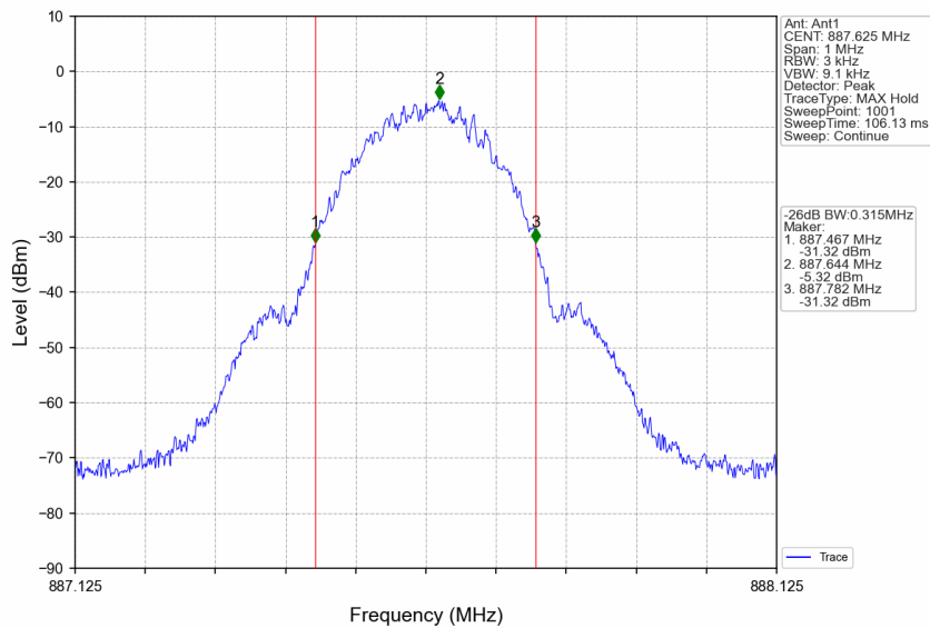
Band26b_887.625MHz_GMSK_SISO_Ant1_NTNV_Input_AGC+3
