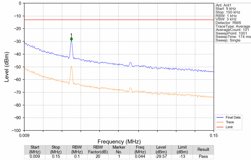
Band26b_869.1MHz_GMSK_SISO_Ant1_NTNV
