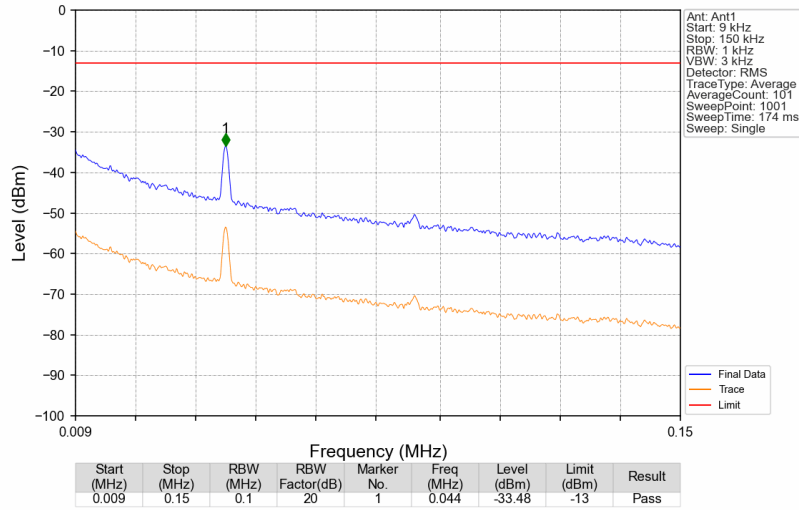
Band26b_881.5MHz_AWGN_SISO_Ant1_NTNV
