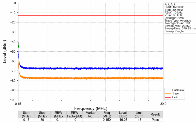
Band26b_881.5MHz_AWGN_SISO_Ant1_NTNV
