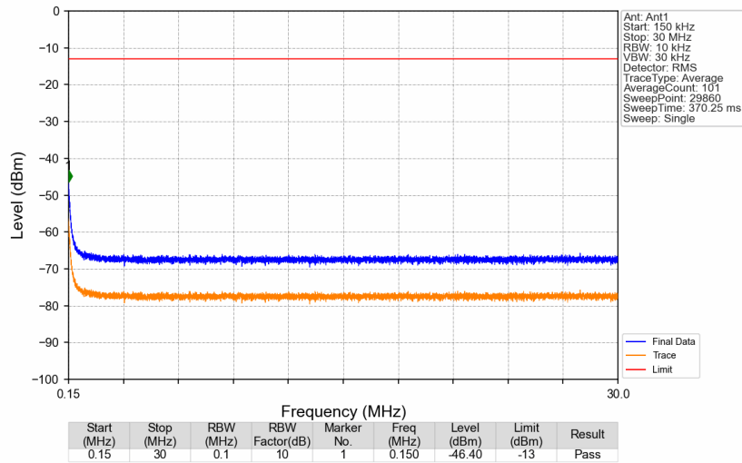
Band26b_881.5MHz_GMSK_SISO_Ant1_NTNV
