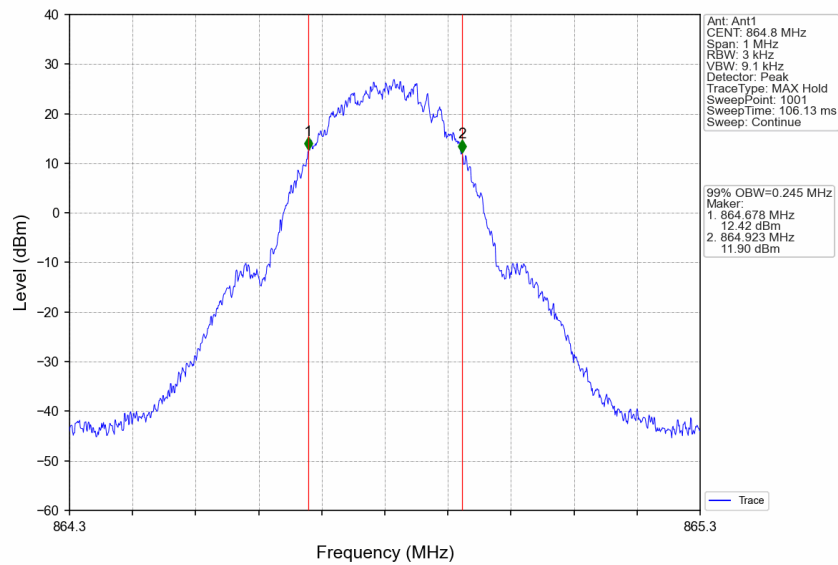
Band26a_864.8MHz_GMSK_SISO_Ant1_NTNV_Output_AGC+3
