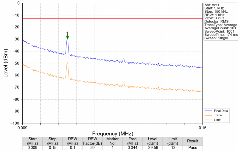
Band26a_866.5MHz_AWGN_SISO_Ant1_NTNV
