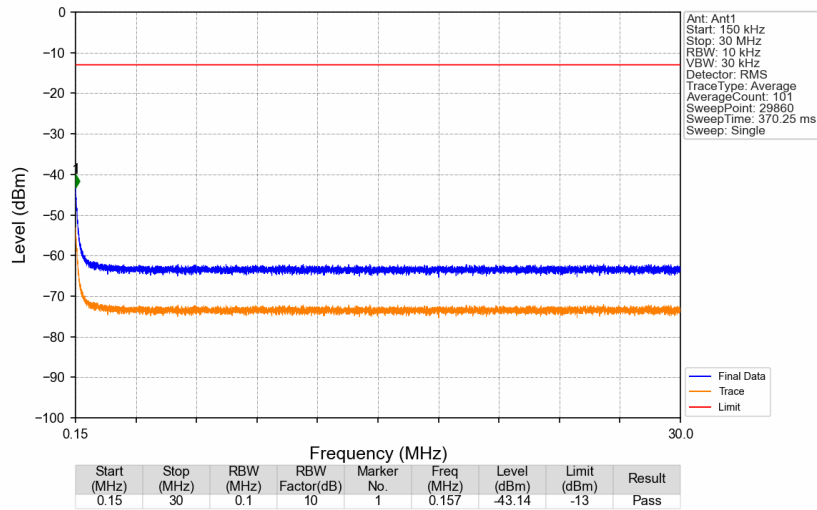
Band13_751MHz_AWGN_SISO_Ant1_NTNV
