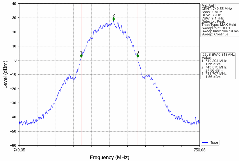
Band13_749.55MHz_GMSK_SISO_Ant1_NTNV_Output_AGC+3
