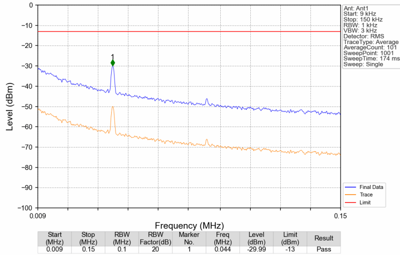
Band13_751MHz_AWGN_SISO_Ant1_NTNV
