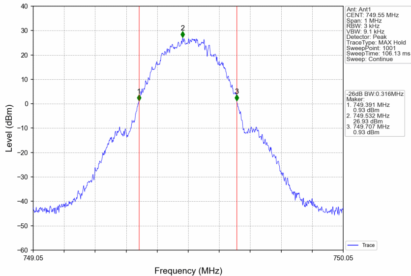
Band13_749.55MHz_GMSK_SISO_Ant1_NTNV_Output_AGC+3
