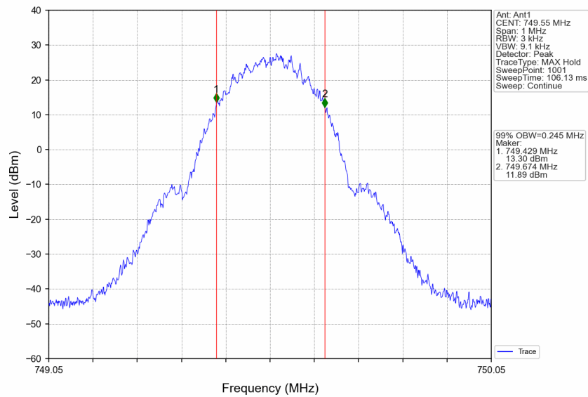
Band13_749.55MHz_GMSK_SISO_Ant1_NTNV_Output_AGC+3
