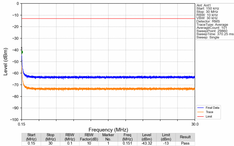
Band13_755.9MHz_GMSK_SISO_Ant1_NTNV
