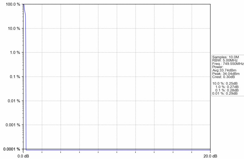
Band13_749.55MHz_GMSK_SISO_Ant1_NTNV_AGC+3
