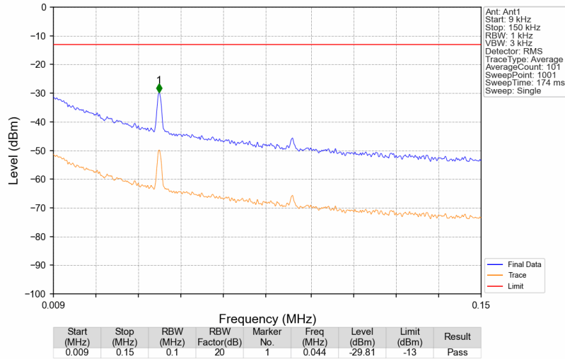
Band13_751MHz_GMSK_SISO_Ant1_NTNV
