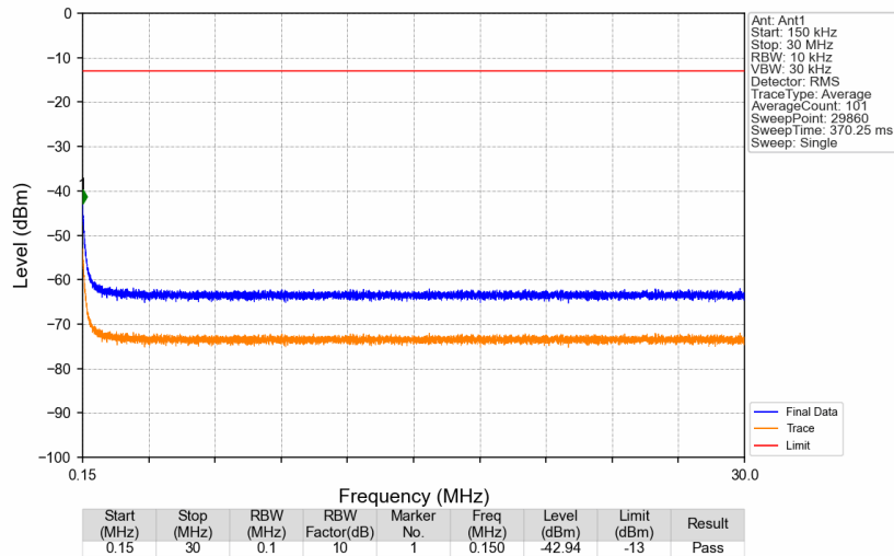
Band13_751MHz_GMSK_SISO_Ant1_NTNV
