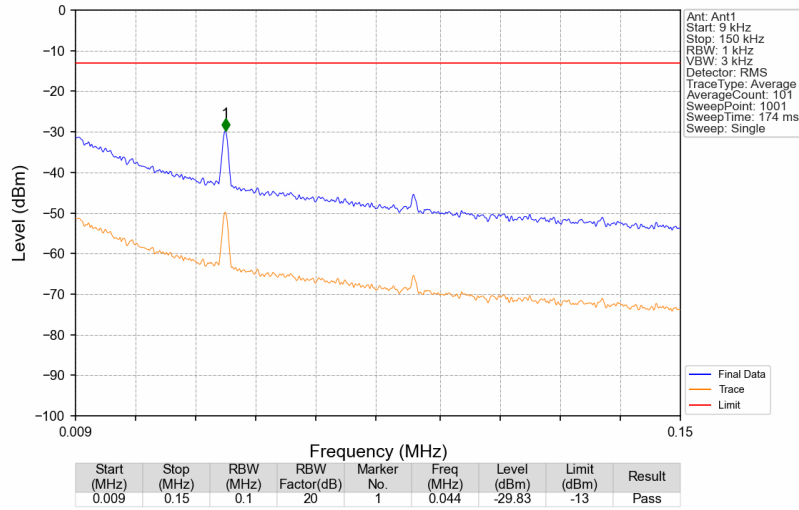
Band13_755.9MHz_GMSK_SISO_Ant1_NTNV
