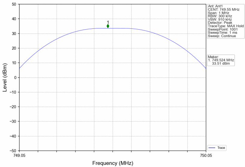
Band13_749.55MHz_GMSK_SISO_Ant1_NTNV_AGC+3
