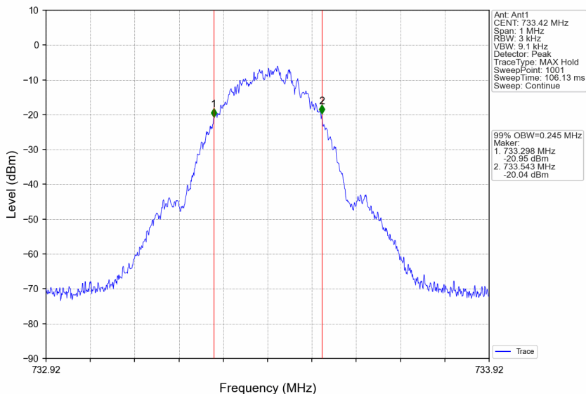
Band12_733.42MHz_GMSK_SISO_Ant1_NTNV_Input_AGC+3
