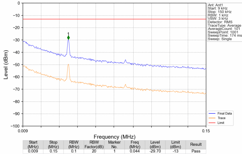
Band12_737.5MHz_AWGN_SISO_Ant1_NTNV
