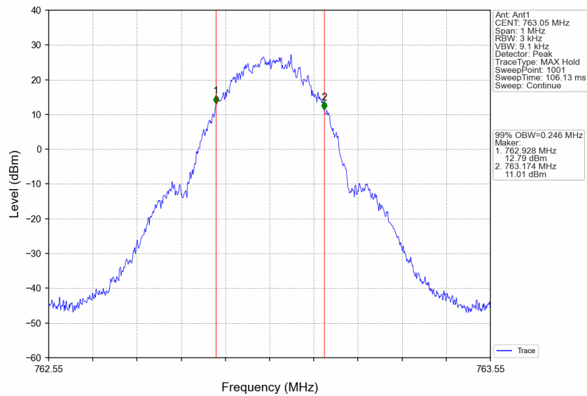
Band14_763.05MHz_GMSK_SISO_Ant1_NTNV_Output_AGC+3
