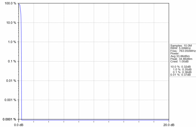
Band14_763.05MHz_GMSK_SISO_Ant1_NTNV_AGC
