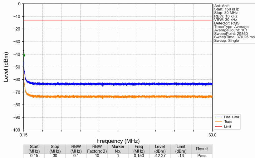
Band14_758.1MHz_GMSK_SISO_Ant1_NTNV
