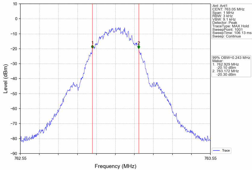
Band14_763.05MHz_GMSK_SISO_Ant1_NTNV_Input_AGC+3
