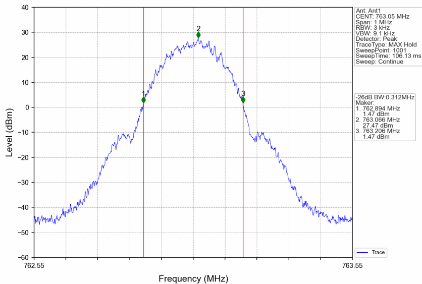
Band14_763.05MHz_GMSK_SISO_Ant1_NTNV_Output_AGC+3
