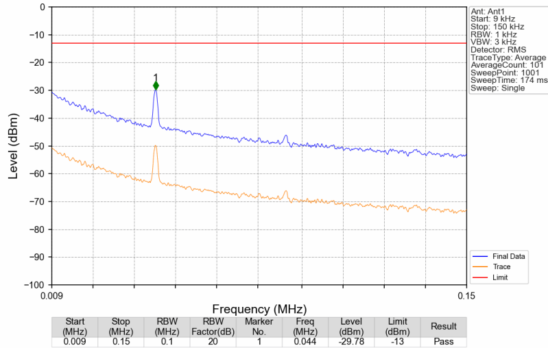
Band14_758.1MHz_GMSK_SISO_Ant1_NTNV
