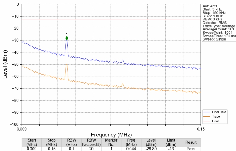
Band14_763MHz_GMSK_SISO_Ant1_NTNV
