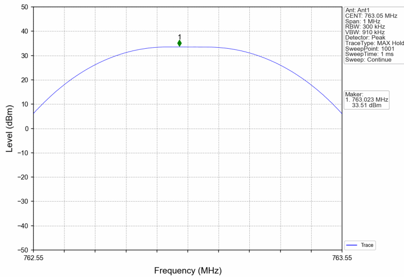
Band14_763.05MHz_GMSK_SISO_Ant1_NTNV_AGC+3
