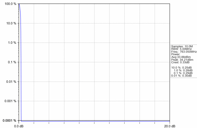
Band14_763.05MHz_GMSK_SISO_Ant1_NTNV_AGC+3
