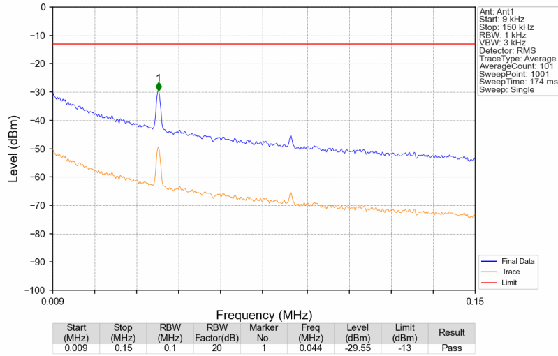
Band14_763MHz_AWGN_SISO_Ant1_NTNV
