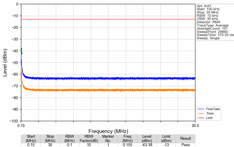
Band14_763MHz_GMSK_SISO_Ant1_NTNV
