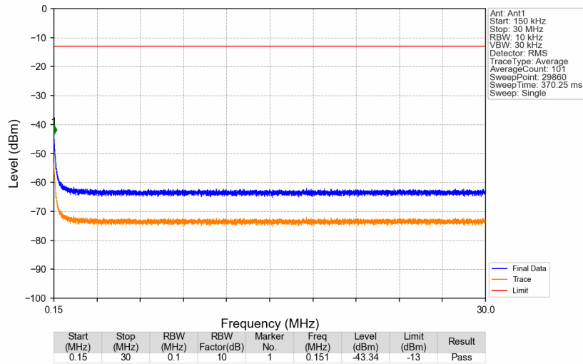
Band14_763MHz_AWGN_SISO_Ant1_NTNV
