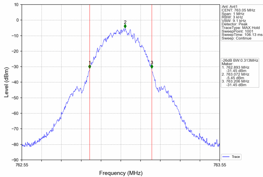
Band14_763.05MHz_GMSK_SISO_Ant1_NTNV_Input_AGC+3
