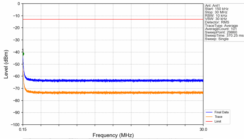
Band71_651.9MHz_GMSK_SISO_Ant1_NTNV
