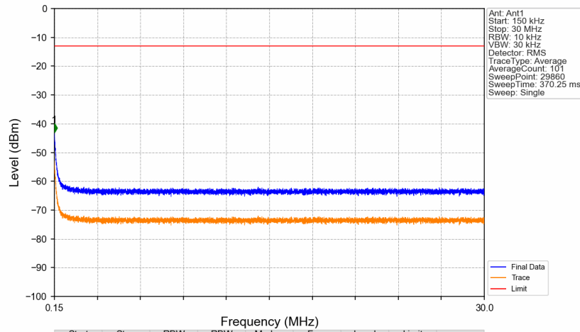
Band71_649.5MHz_AWGN_SISO_Ant1_NTNV
