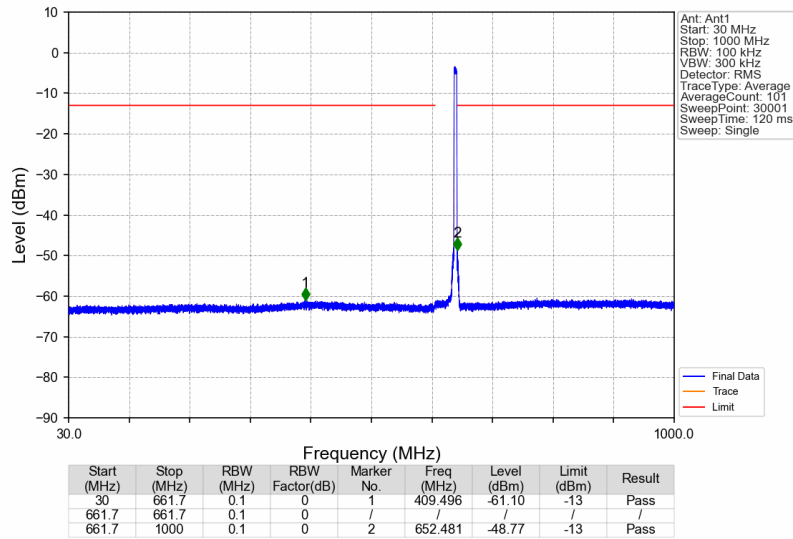
Band71_649.5MHz_AWGN_SISO_Ant1_NTNV
