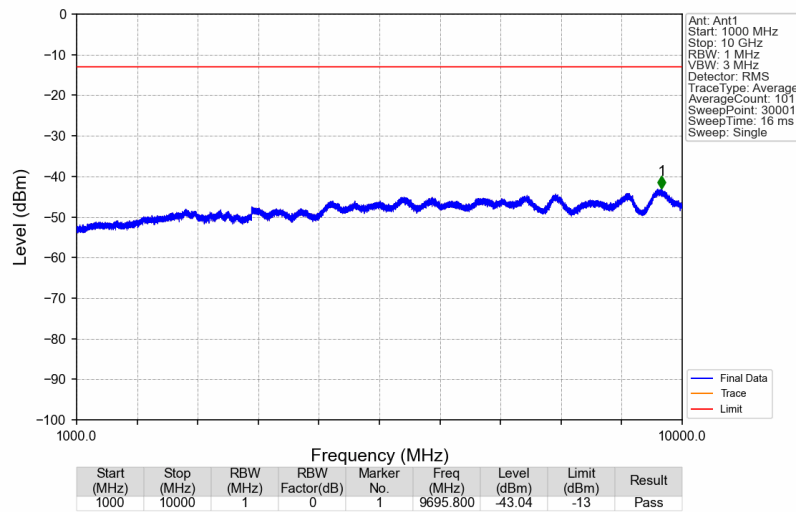
Band71_649.5MHz_AWGN_SISO_Ant1_NTNV
