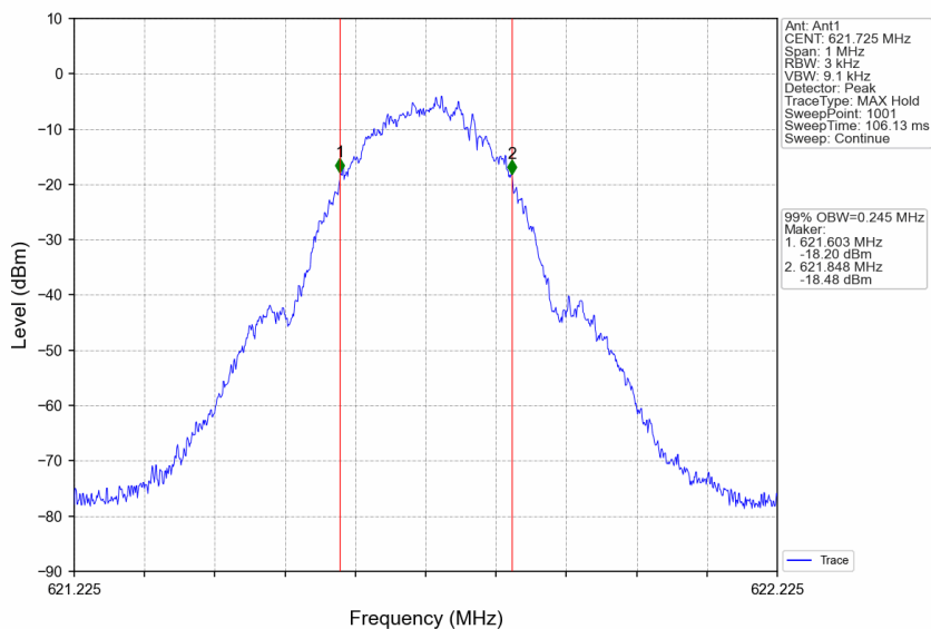
Band71_621.725MHz_GMSK_SISO_Ant1_NTNV_Input_AGC+3
