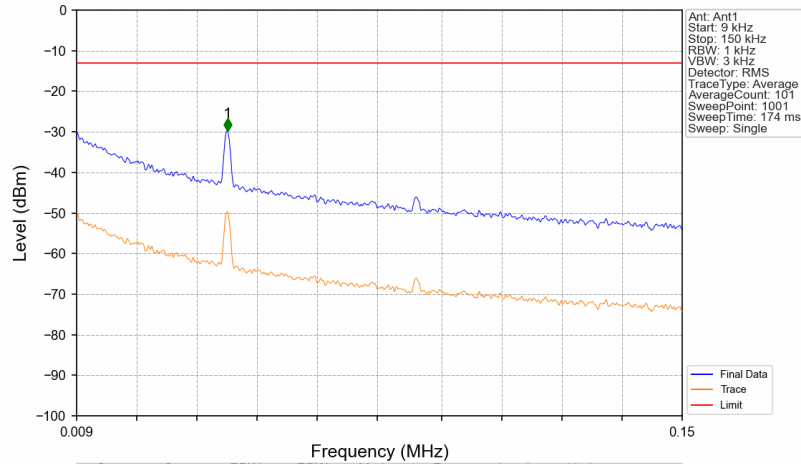
Band71_651.9MHz_GMSK_SISO_Ant1_NTNV
