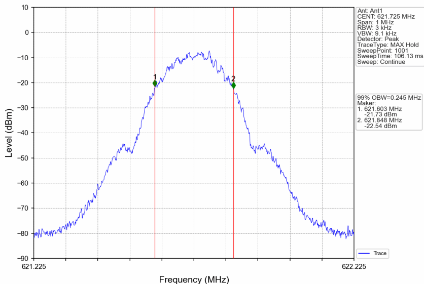
Band71_621.725MHz_GMSK_SISO_Ant1_NTNV_Input_AGC+3
