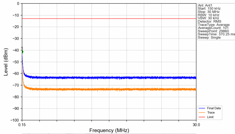
Band71_617.1MHz_GMSK_SISO_Ant1_NTNV
