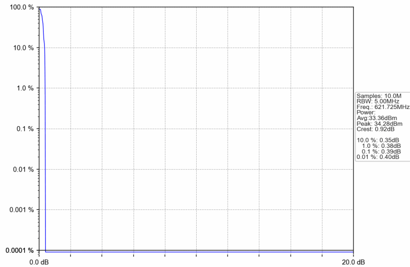
Band71_621.725MHz_GMSK_SISO_Ant1_NTNV_AGC
