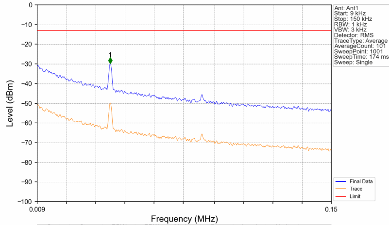
Band71_634.5MHz_GMSK_SISO_Ant1_NTNV
