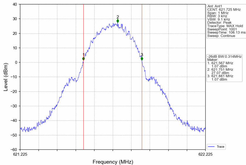
Band71_621.725MHz_GMSK_SISO_Ant1_NTNV_Output_AGC+3
