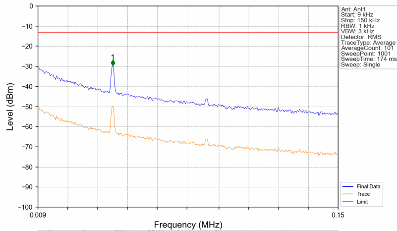
Band71_649.5MHz_AWGN_SISO_Ant1_NTNV
