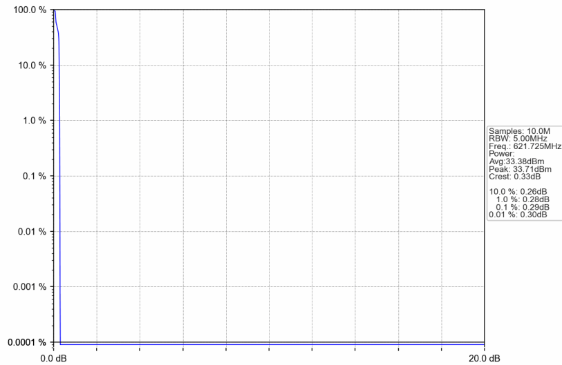
Band71_621.725MHz_GMSK_SISO_Ant1_NTNV_AGC+3
