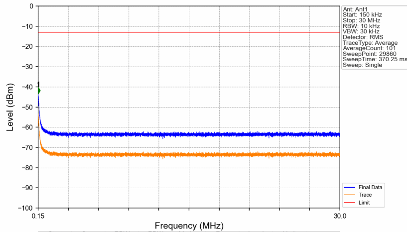
Band71_634.5MHz_GMSK_SISO_Ant1_NTNV
