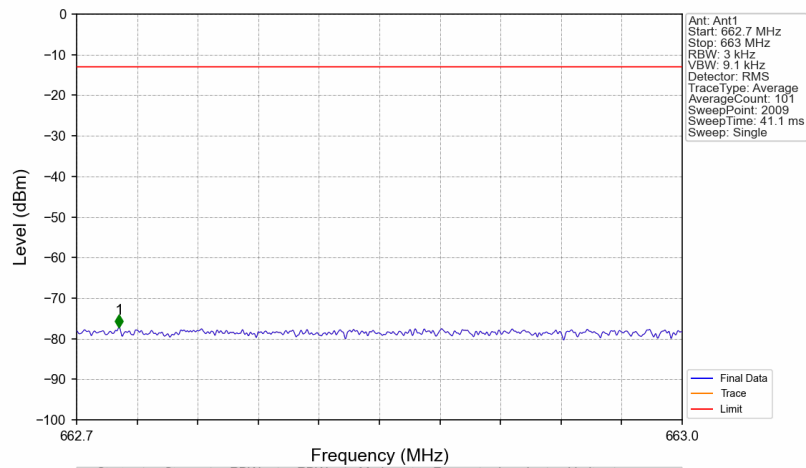
Band71_617.1MHz_GMSK_SISO_Ant1_NTNV_AGC+3
