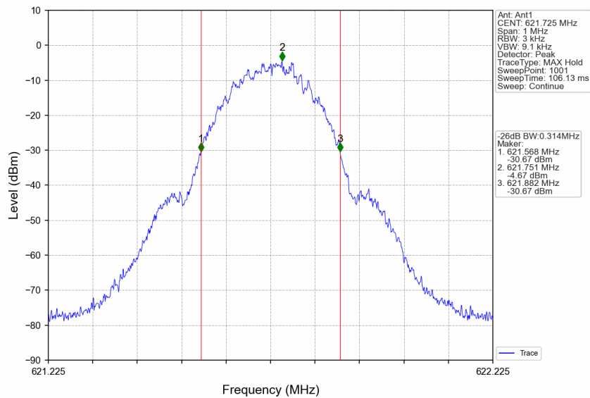
Band71_621.725MHz_GMSK_SISO_Ant1_NTNV_Input_AGC+3
