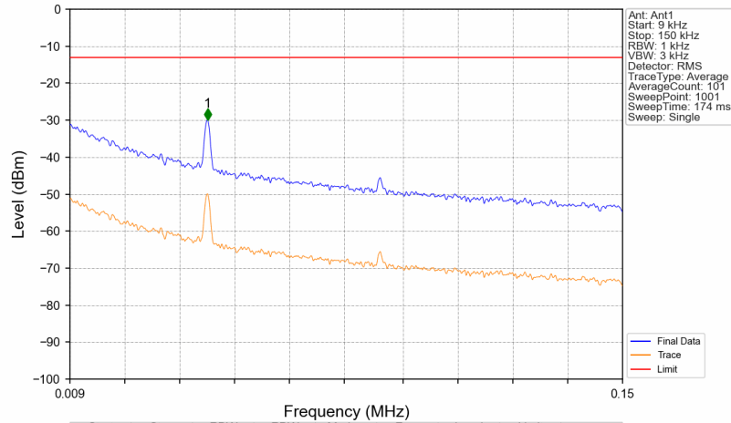
Band71_617.1MHz_GMSK_SISO_Ant1_NTNV
