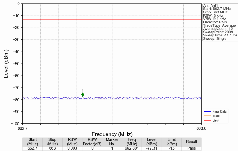
Band71_617.1MHz_GMSK_SISO_Ant1_NTNV_AGC
