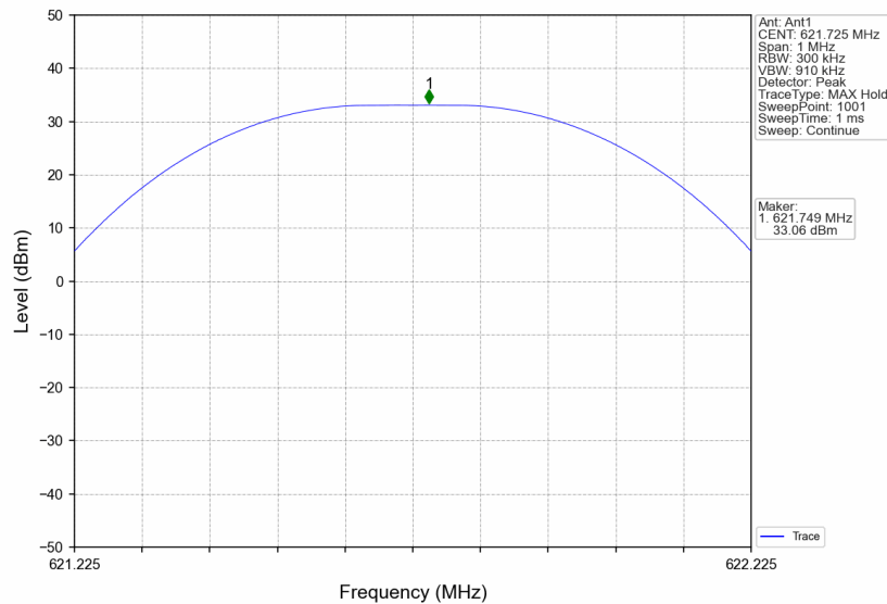
Band71_621.725MHz_GMSK_SISO_Ant1_NTNV_AGC+3
