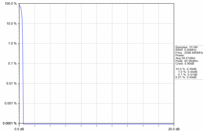
Band41_2596.88MHz_GMSK_SISO_Ant1_NTNV_AGC
