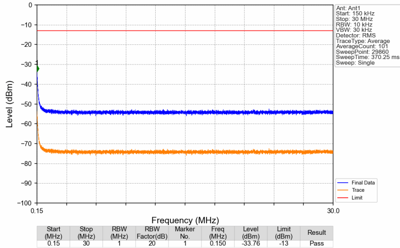
Band41_2593MHz_AWGN_SISO_Ant1_NTNV
