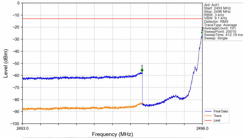
Band41_2496.1MHz_GMSK_SISO_Ant1_NTNV_AGC
