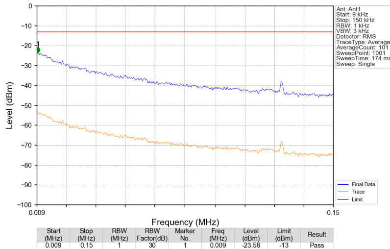
Band41_2593MHz_AWGN_SISO_Ant1_NTNV
