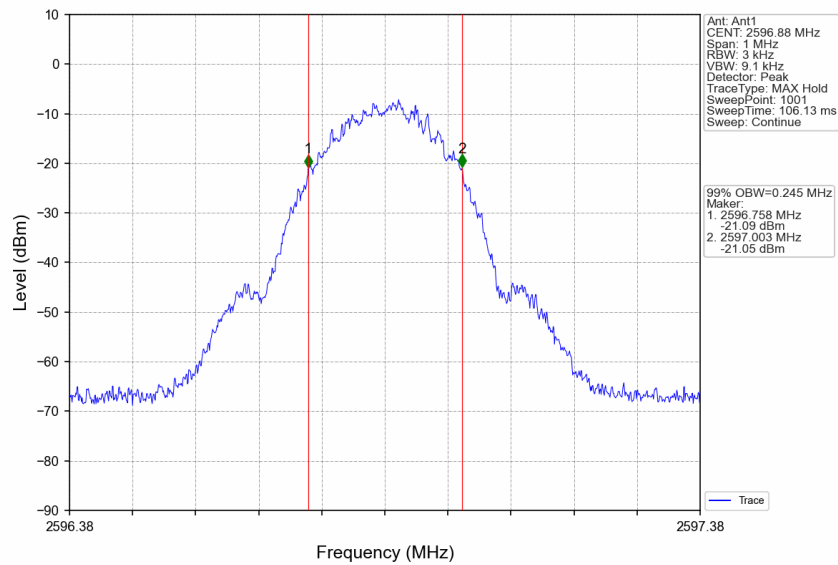
Band41_2596.88MHz_GMSK_SISO_Ant1_NTNV_Input_AGC+3
