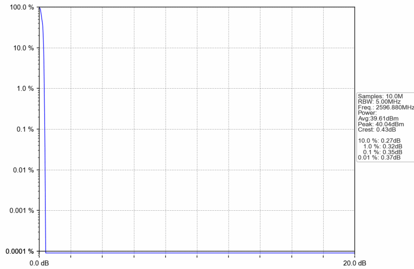
Band41_2596.88MHz_GMSK_SISO_Ant1_NTNV_AGC+3
