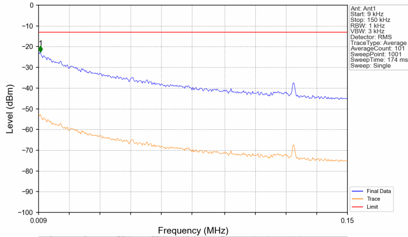
Band41_2593MHz_GMSK_SISO_Ant1_NTNV
