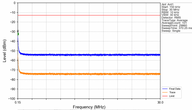
Band41_2593MHz_GMSK_SISO_Ant1_NTNV
