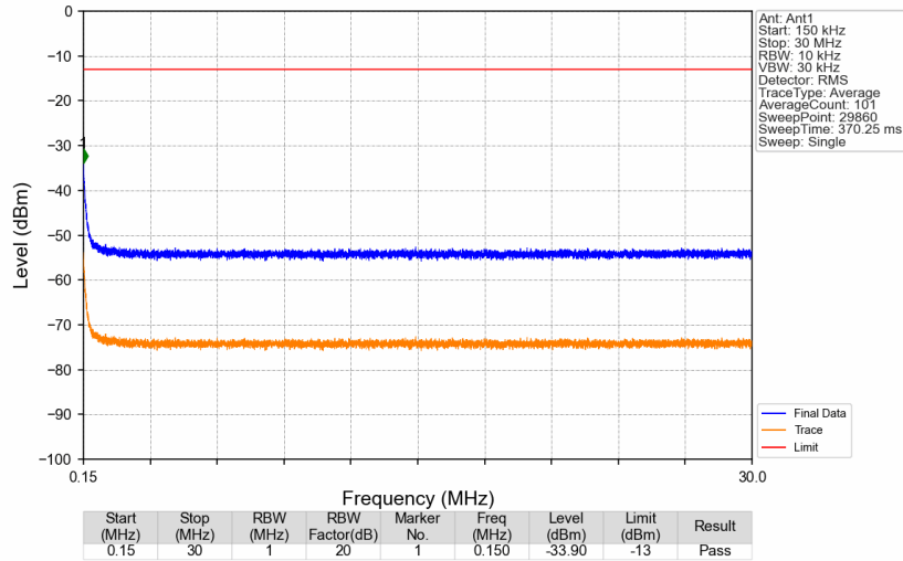
Band41_2689.9MHz_GMSK_SISO_Ant1_NTNV
