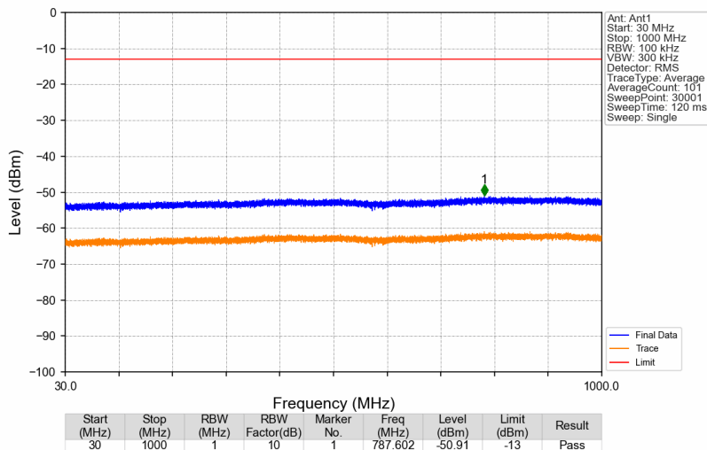
Band41_2593MHz_GMSK_SISO_Ant1_NTNV
