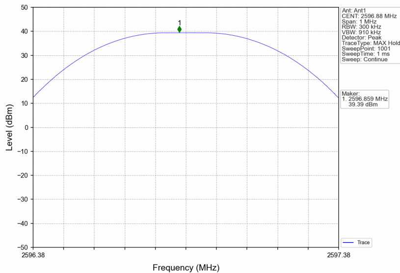
Band41_2596.88MHz_GMSK_SISO_Ant1_NTNV_AGC+3
