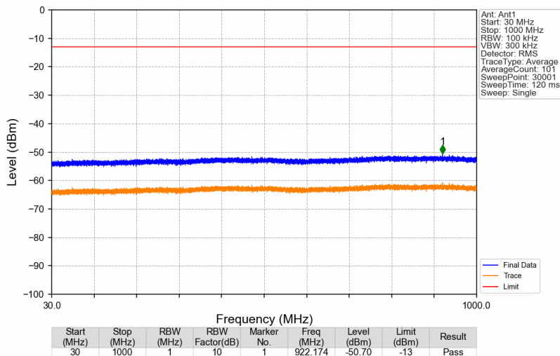
Band41_2496.1MHz_GMSK_SISO_Ant1_NTNV
