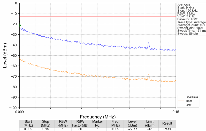
Band41_2689.9MHz_GMSK_SISO_Ant1_NTNV
