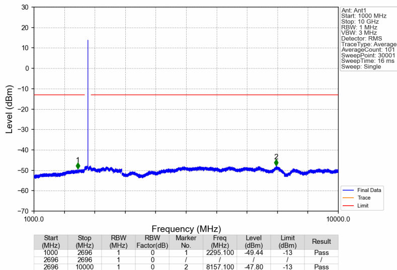
Band41_2593MHz_GMSK_SISO_Ant1_NTNV
