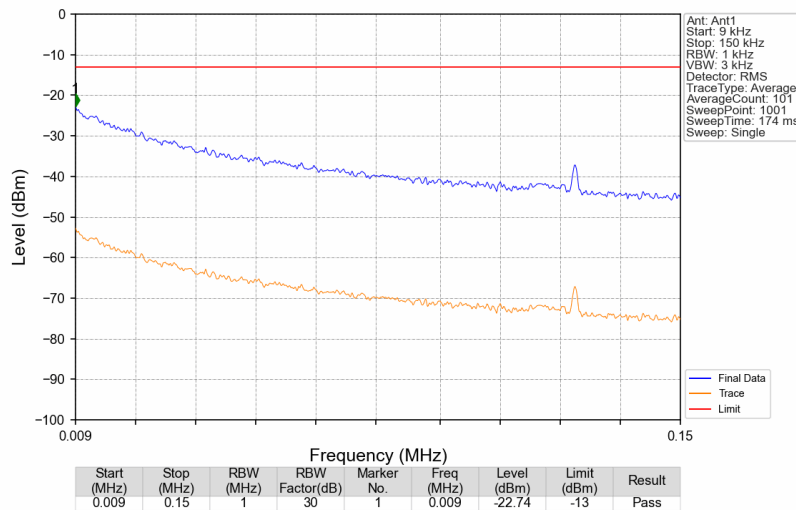
Band41_2496.1MHz_GMSK_SISO_Ant1_NTNV
