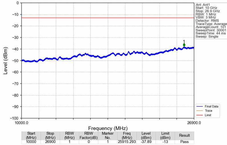
Band41_2498.5MHz_AWGN_SISO_Ant1_NTNV
