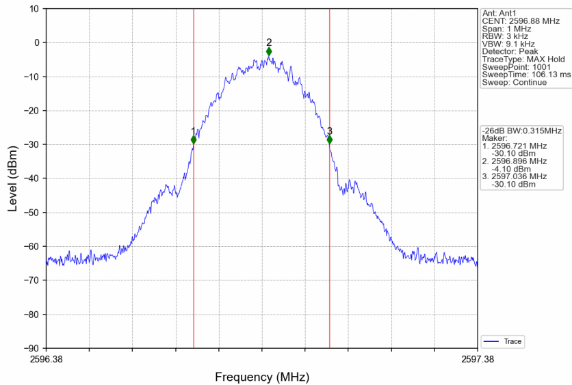
Band41_2596.88MHz_GMSK_SISO_Ant1_NTNV_Input_AGC+3
