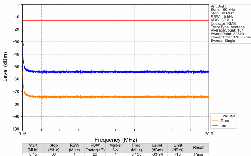
Band41_2496.1MHz_GMSK_SISO_Ant1_NTNV
