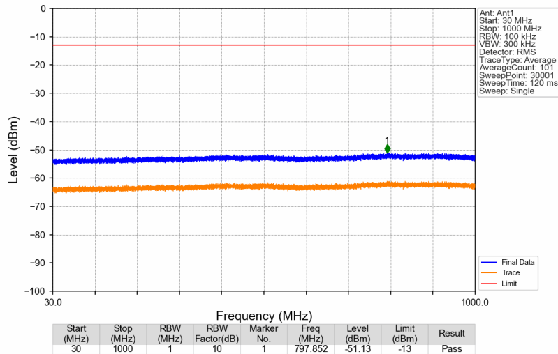
Band41_2593MHz_AWGN_SISO_Ant1_NTNV
