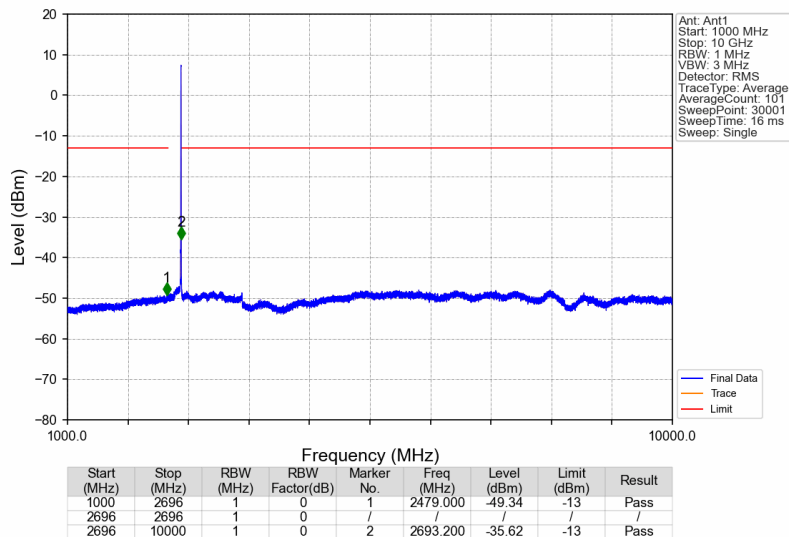
Band41_2687.5MHz_AWGN_SISO_Ant1_NTNV
