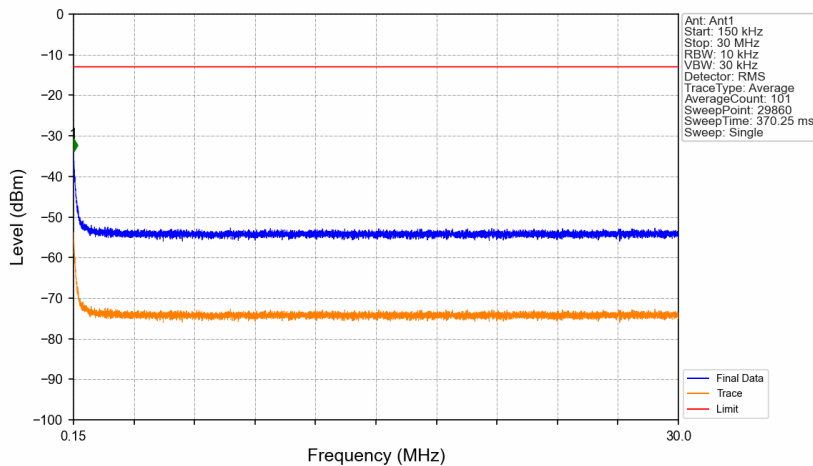
Band41_2687.5MHz_AWGN_SISO_Ant1_NTNV
