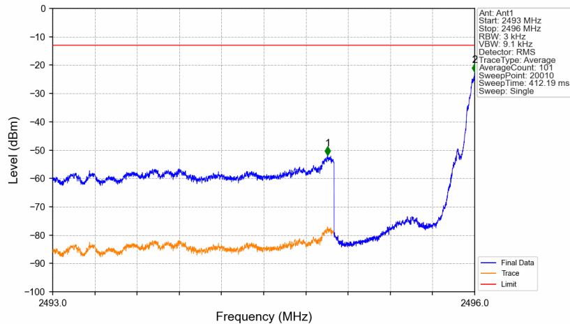
Band41_2496.1MHz_GMSK_SISO_Ant1_NTNV_AGC+3
