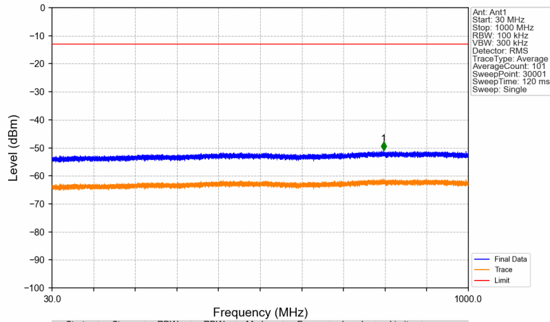
Band41_2498.5MHz_AWGN_SISO_Ant1_NTNV
