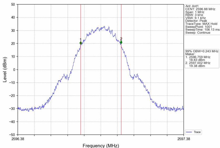
Band41_2596.88MHz_GMSK_SISO_Ant1_NTNV_Output_AGC+3
