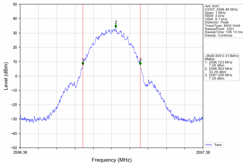
Band41_2596.88MHz_GMSK_SISO_Ant1_NTNV_Output_AGC+3
