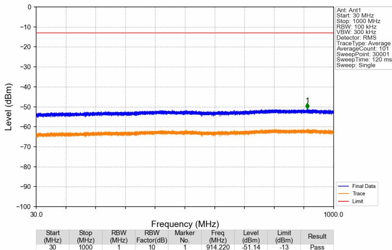
Band41_2687.5MHz_AWGN_SISO_Ant1_NTNV
