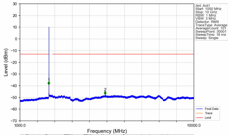
Band41_2498.5MHz_AWGN_SISO_Ant1_NTNV
