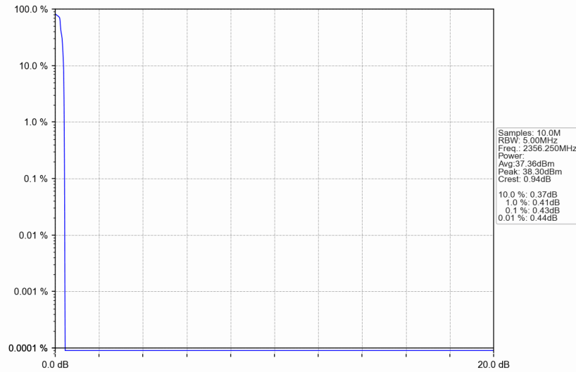
Band30_2356.25MHz_GMSK_SISO_Ant1_NTNV_AGC
