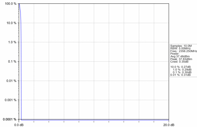
Band30_2356.25MHz_GMSK_SISO_Ant1_NTNV_AGC+3
