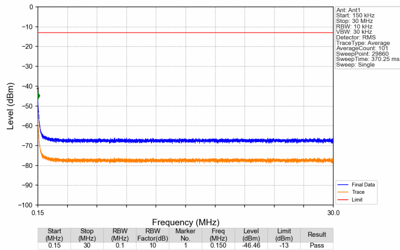
Band26b_893.9MHz_GMSK_SISO_Ant1_NTNV
