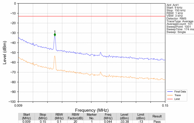
Band26b_891.5MHz_AWGN_SISO_Ant1_NTNV
