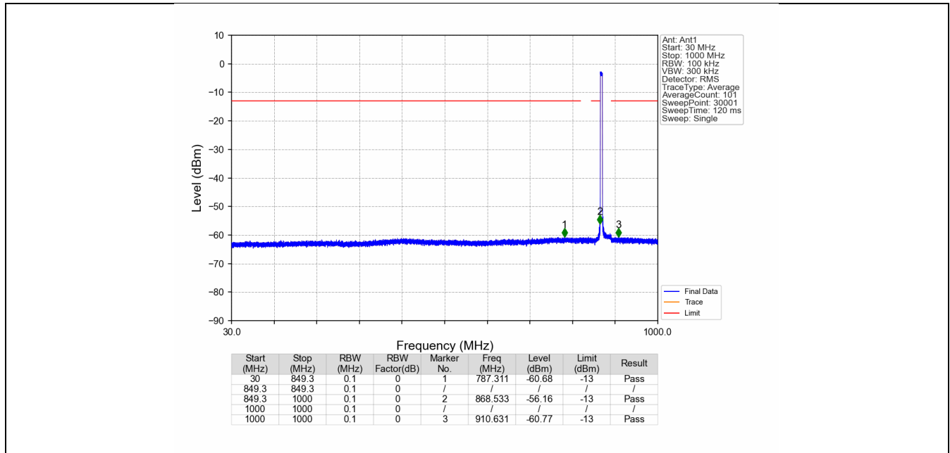
Band26b_871.5MHz_AWGN_SISO_Ant1_NTNV
