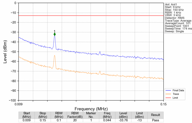
Band26b_893.9MHz_GMSK_SISO_Ant1_NTNV
