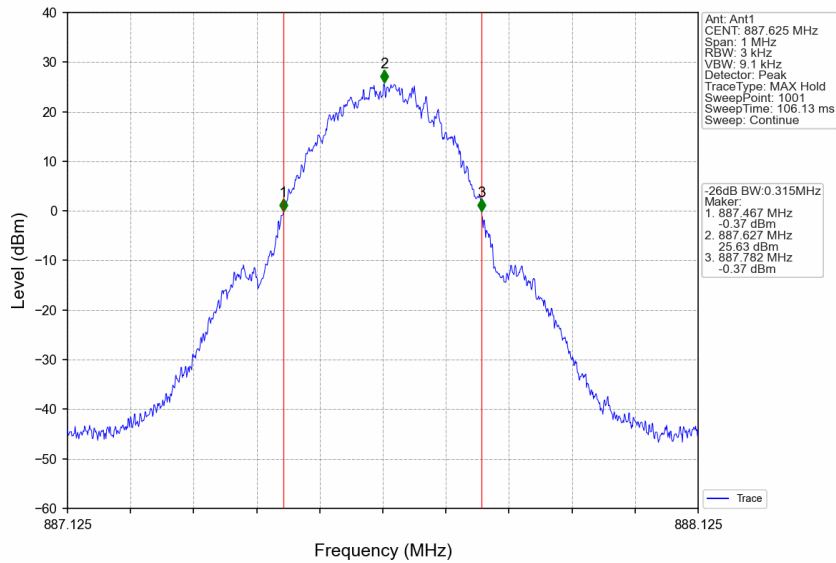
Band26b_887.625MHz_GMSK_SISO_Ant1_NTNV_Output_AGC+3
