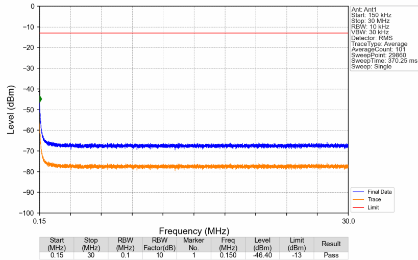
Band26b_881.5MHz_GMSK_SISO_Ant1_NTNV
