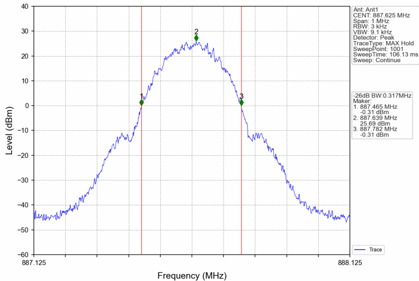
Band26b_887.625MHz_GMSK_SISO_Ant1_NTNV_Output_AGC+3
