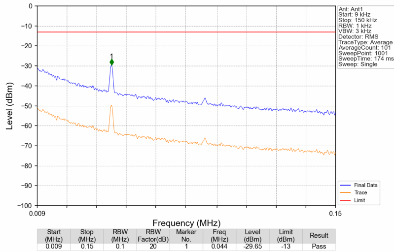
Band26a_865.5MHz_GMSK_SISO_Ant1_NTNV
