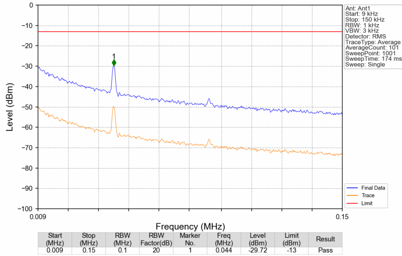
Band26a_868.9MHz_GMSK_SISO_Ant1_NTNV
