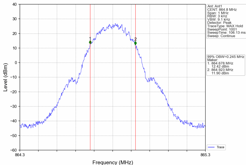
Band26a_864.8MHz_GMSK_SISO_Ant1_NTNV_Output_AGC+3
