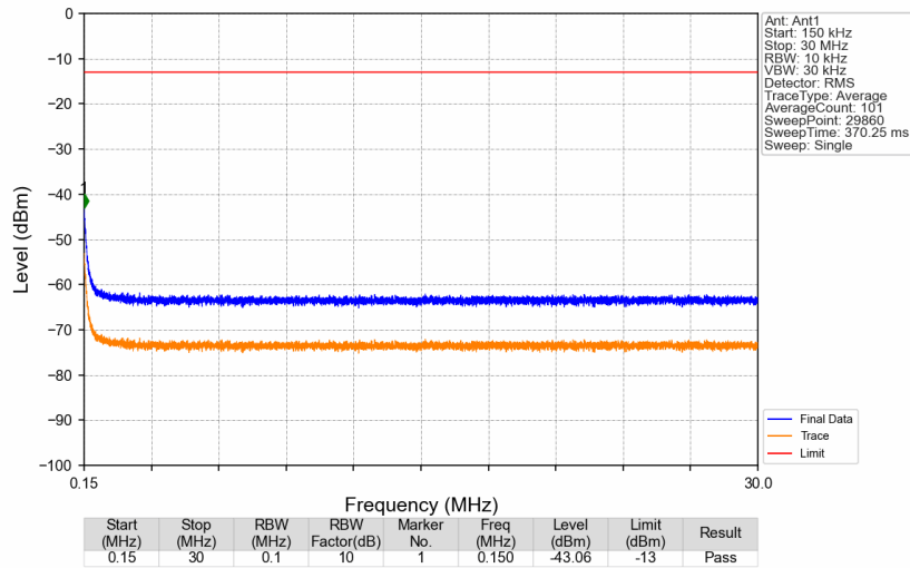
Band26a_862.1MHz_GMSK_SISO_Ant1_NTNV
