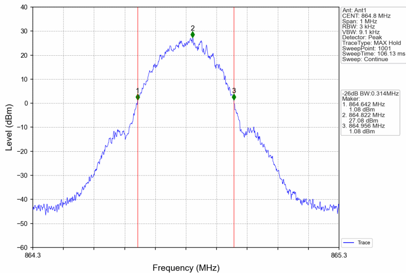
Band26a_864.8MHz_GMSK_SISO_Ant1_NTNV_Output_AGC+3
