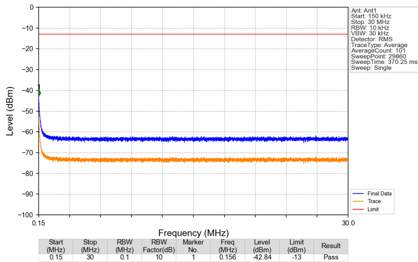
Band26a_865.5MHz_GMSK_SISO_Ant1_NTNV
