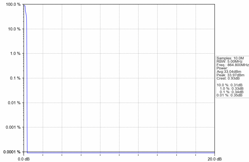
Band26a_864.8MHz_GMSK_SISO_Ant1_NTNV_AGC
