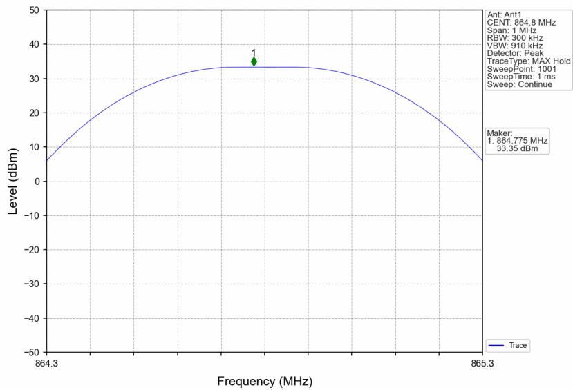
Band26a_864.8MHz_GMSK_SISO_Ant1_NTNV_AGC+3
