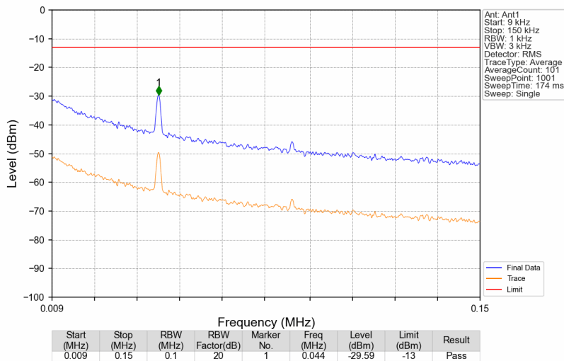
Band26a_866.5MHz_AWGN_SISO_Ant1_NTNV
