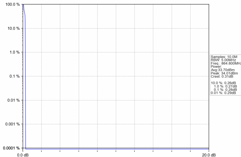
Band26a_864.8MHz_GMSK_SISO_Ant1_NTNV_AGC+3
