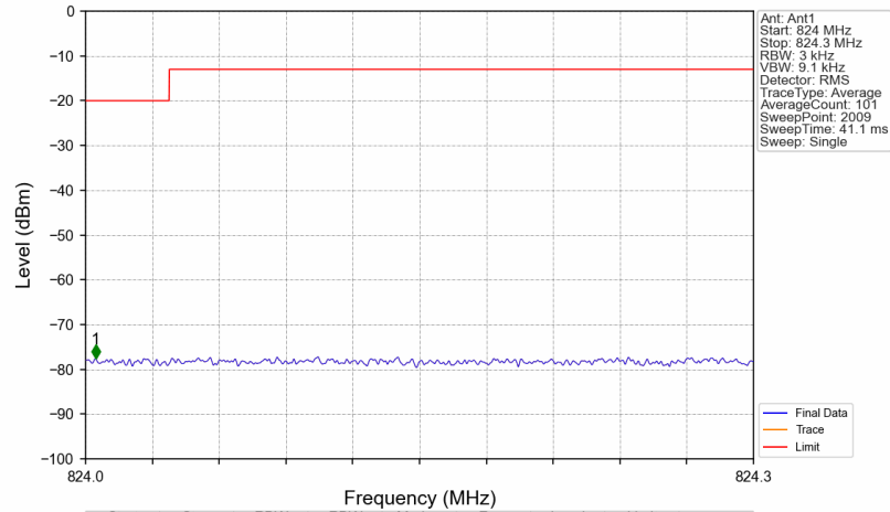
Band26a_868.9MHz_GMSK_SISO_Ant1_NTNV_AGC
