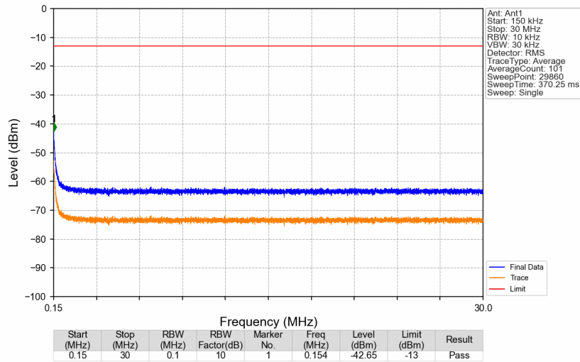
Band26a_868.9MHz_GMSK_SISO_Ant1_NTNV
