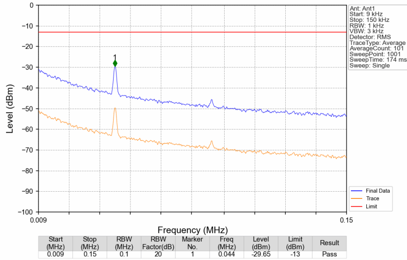
Band26a_862.1MHz_GMSK_SISO_Ant1_NTNV
