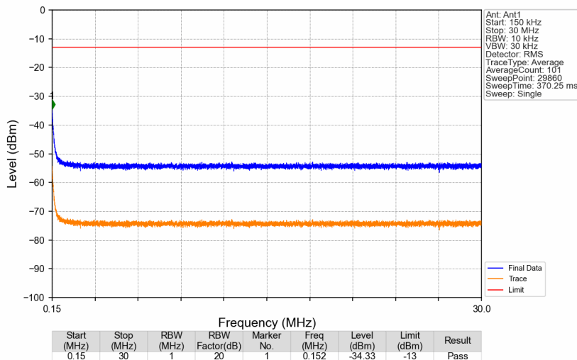
Band25_1962.5MHz_GMSK_SISO_Ant1_NTNV
