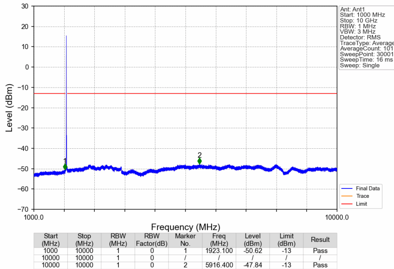
Band25_1962.5MHz_GMSK_SISO_Ant1_NTNV
