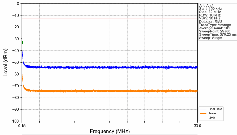
Band25_1992.5MHz_AWGN_SISO_Ant1_NTNV
