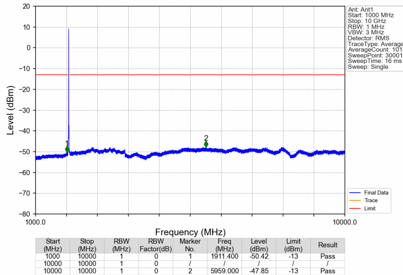
Band25_1962.5MHz_AWGN_SISO_Ant1_NTNV
