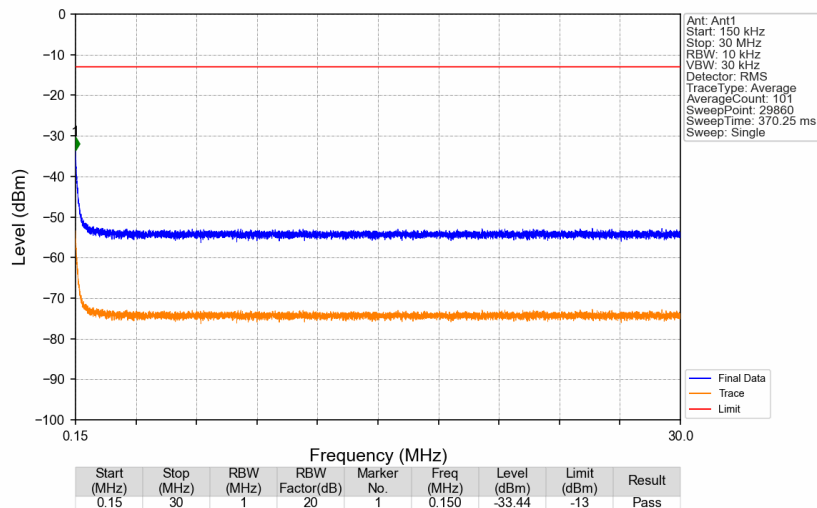
Band25_1930.1MHz_GMSK_SISO_Ant1_NTNV
