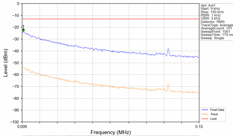
Band25_1930.1MHz_GMSK_SISO_Ant1_NTNV
