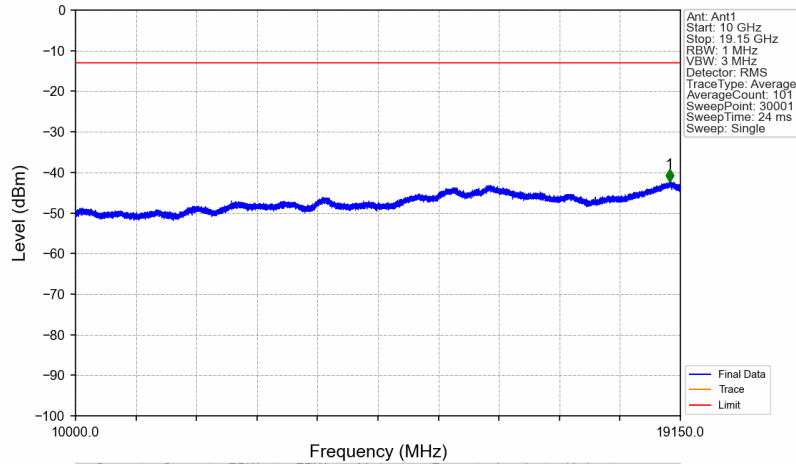
Band25_1992.5MHz_AWGN_SISO_Ant1_NTNV
