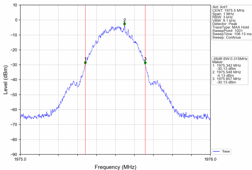
Band25_1975.5MHz_GMSK_SISO_Ant1_NTNV_Input_AGC+3
