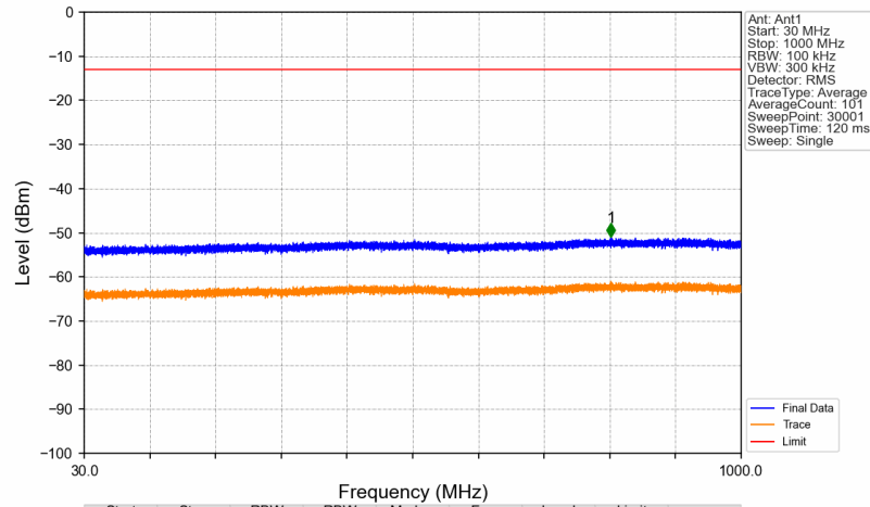
Band25_1932.5MHz_AWGN_SISO_Ant1_NTNV
