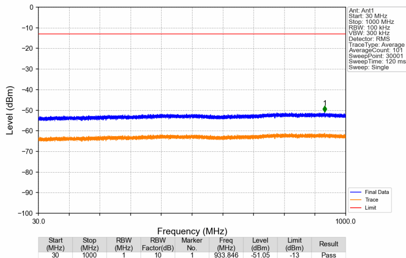
Band25_1994.9MHz_GMSK_SISO_Ant1_NTNV
