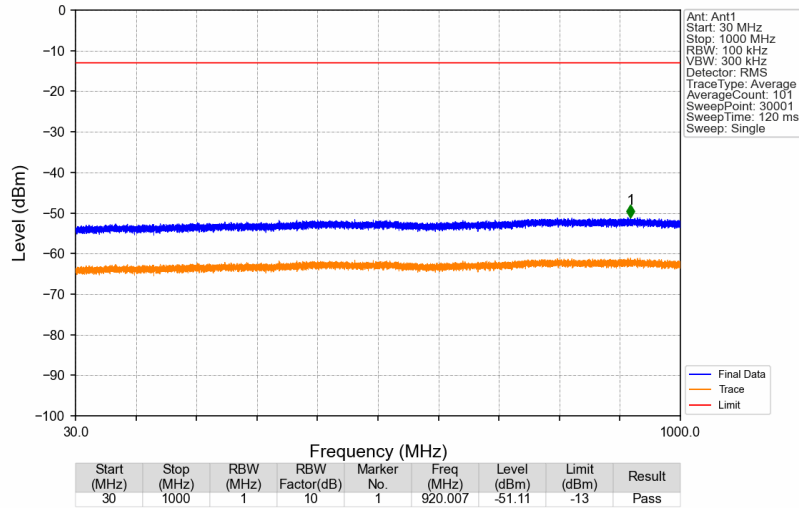
Band25_1962.5MHz_GMSK_SISO_Ant1_NTNV
