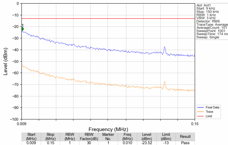
Band25_1994.9MHz_GMSK_SISO_Ant1_NTNV
