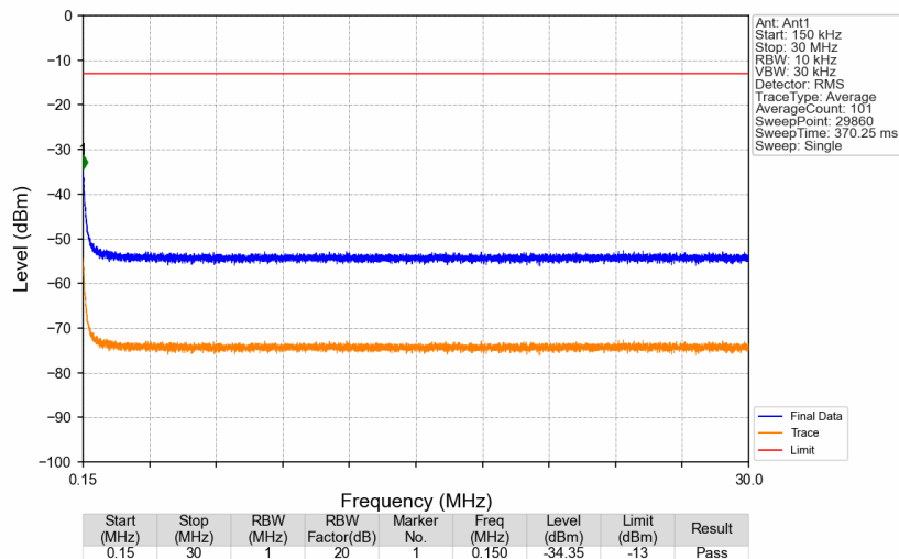
Band25_1994.9MHz_GMSK_SISO_Ant1_NTNV
