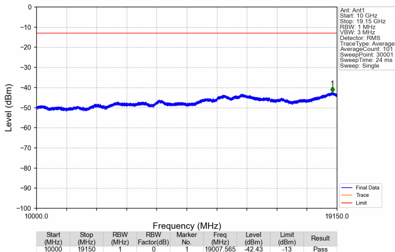
Band25_1932.5MHz_AWGN_SISO_Ant1_NTNV
