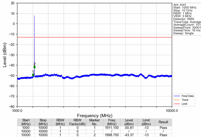
Band25_1992.5MHz_AWGN_SISO_Ant1_NTNV
