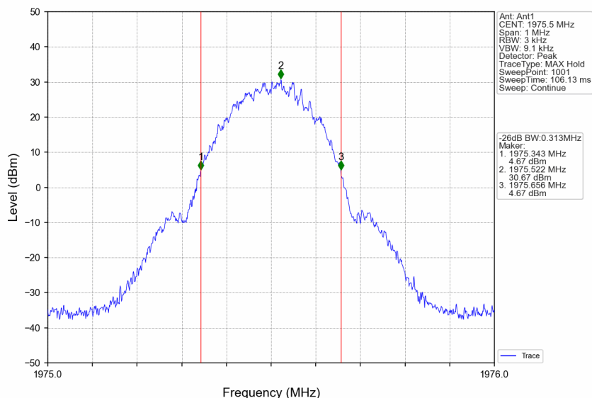
Band25_1975.5MHz_GMSK_SISO_Ant1_NTNV_Output_AGC+3
