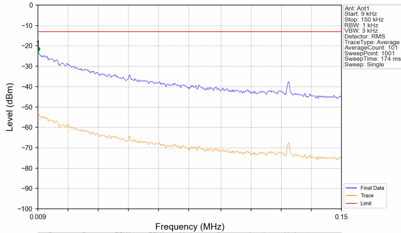
Band25_1992.5MHz_AWGN_SISO_Ant1_NTNV
