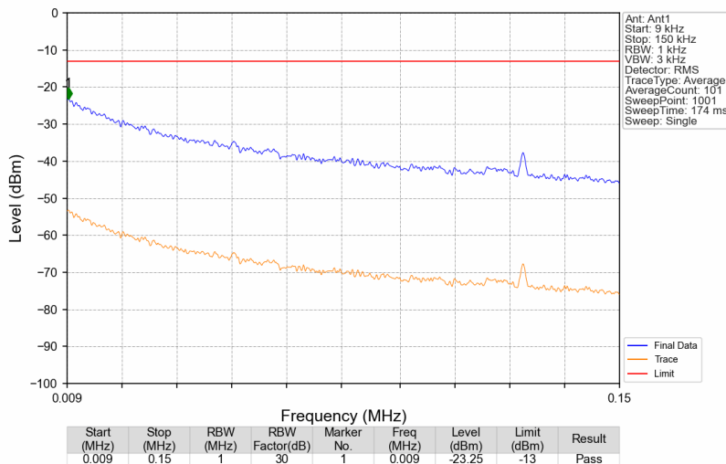
Band25_1962.5MHz_AWGN_SISO_Ant1_NTNV
