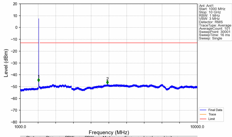
Band25_1932.5MHz_AWGN_SISO_Ant1_NTNV
