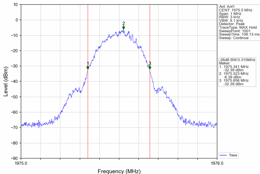
Band25_1975.5MHz_GMSK_SISO_Ant1_NTNV_Input_AGC+3
