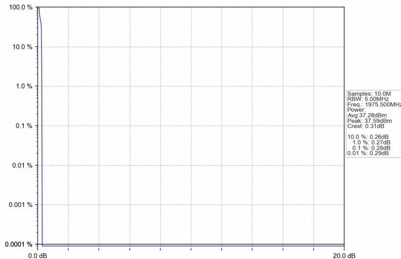
Band25_1975.5MHz_GMSK_SISO_Ant1_NTNV_AGC+3
