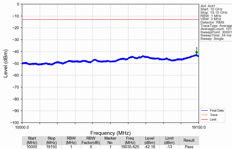
Band25_1962.5MHz_AWGN_SISO_Ant1_NTNV
