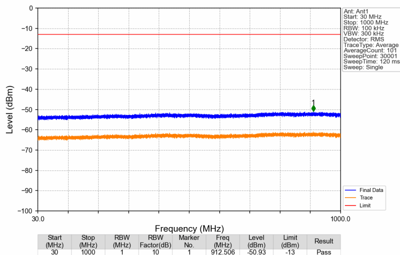
Band25_1930.1MHz_GMSK_SISO_Ant1_NTNV
