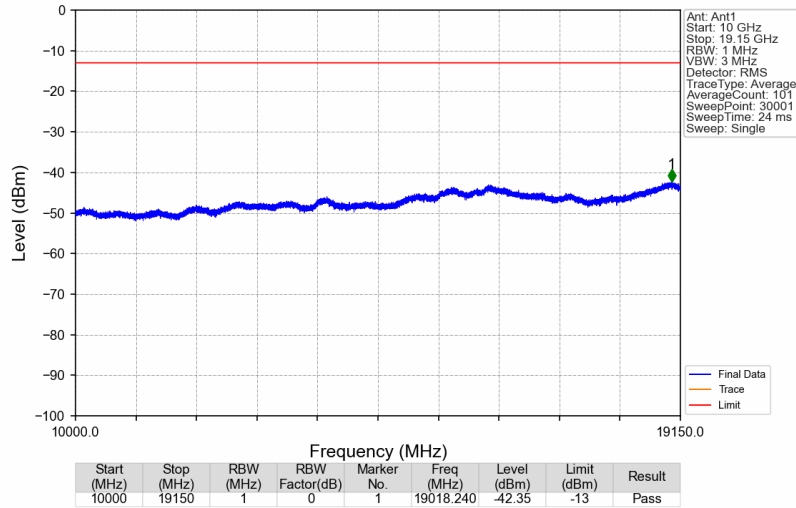
Band25_1962.5MHz_GMSK_SISO_Ant1_NTNV
