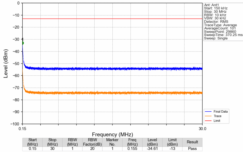
Band25_1962.5MHz_AWGN_SISO_Ant1_NTNV
