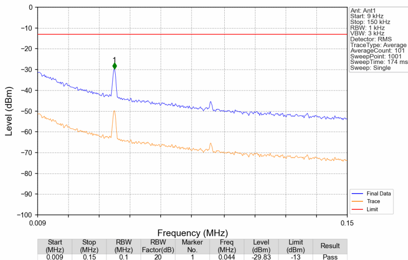
Band13_755.9MHz_GMSK_SISO_Ant1_NTNV
