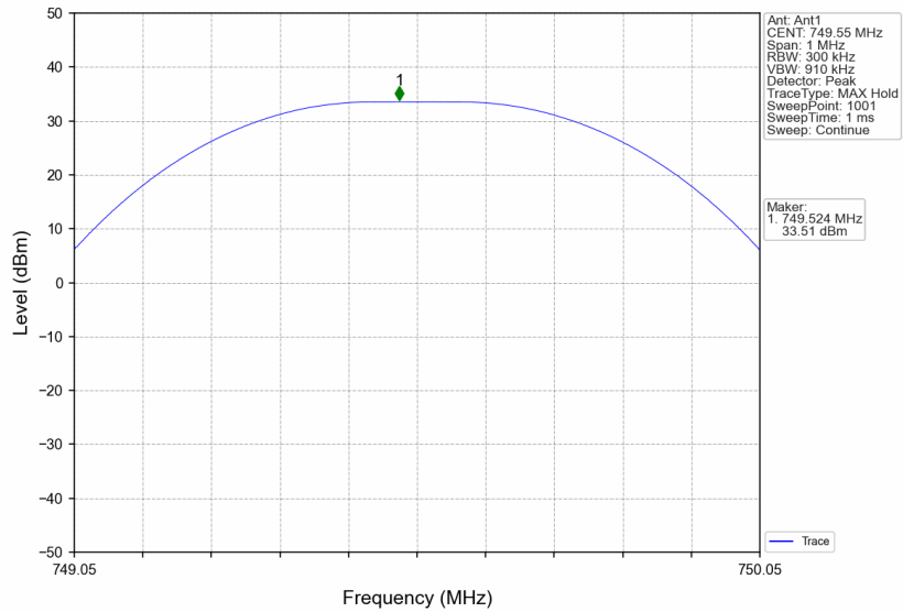
Band13_749.55MHz_GMSK_SISO_Ant1_NTNV_AGC+3
