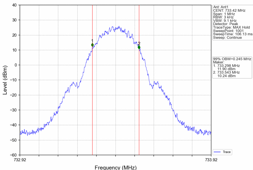
Band12_733.42MHz_GMSK_SISO_Ant1_NTNV_Output_AGC+3
