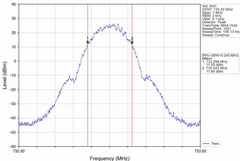
Band12_733.42MHz_GMSK_SISO_Ant1_NTNV_Output_AGC+3
