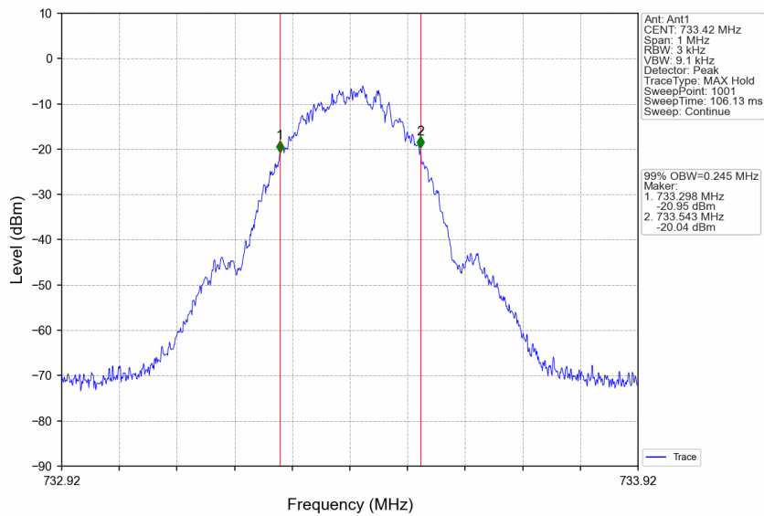
Band12_733.42MHz_GMSK_SISO_Ant1_NTNV_Input_AGC+3
