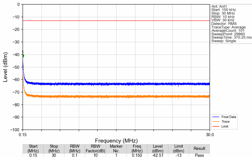
Band12_737.5MHz_AWGN_SISO_Ant1_NTNV
