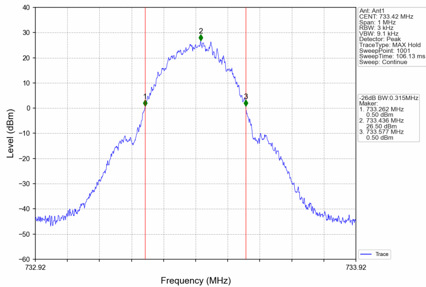
Band12_733.42MHz_GMSK_SISO_Ant1_NTNV_Output_AGC+3
