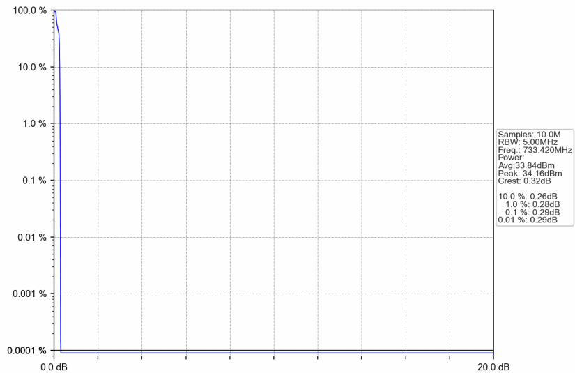
Band12_733.42MHz_GMSK_SISO_Ant1_NTNV_AGC+3
