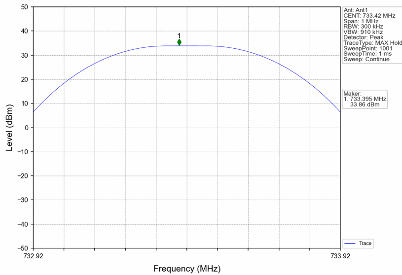
Band12_733.42MHz_GMSK_SISO_Ant1_NTNV_AGC+3
