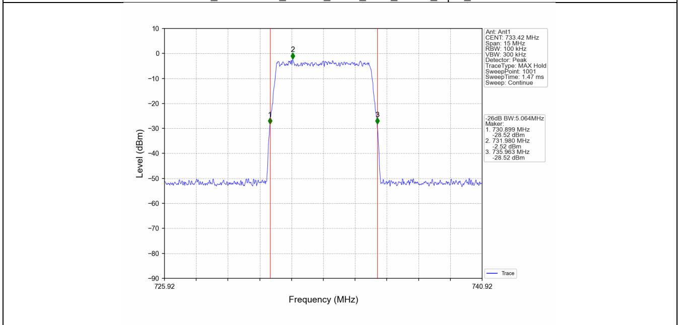
Band12_733.42MHz_AWGN_SISO_Ant1_NTNV_Input_AGC+3
