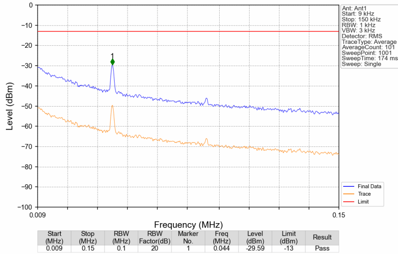
Band12_743.5MHz_AWGN_SISO_Ant1_NTNV
