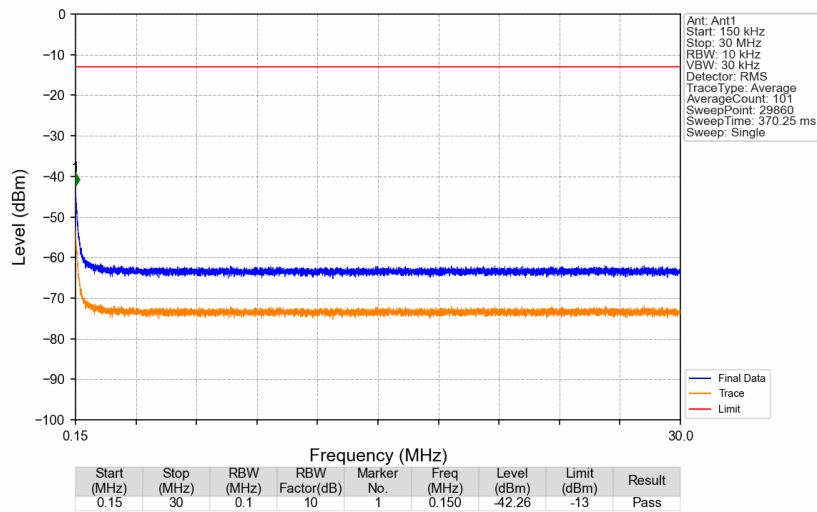
Band12_745.9MHz_GMSK_SISO_Ant1_NTNV
