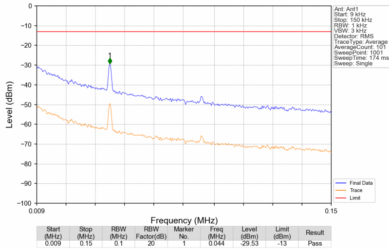
Band12_745.9MHz_GMSK_SISO_Ant1_NTNV
