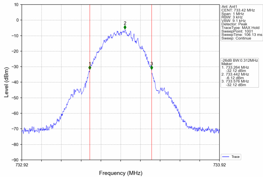
Band12_733.42MHz_GMSK_SISO_Ant1_NTNV_Input_AGC+3
