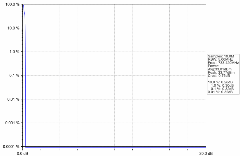
Band12_733.42MHz_GMSK_SISO_Ant1_NTNV_AGC
