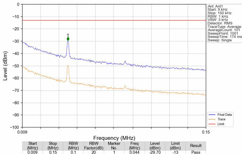
Band12_737.5MHz_AWGN_SISO_Ant1_NTNV
