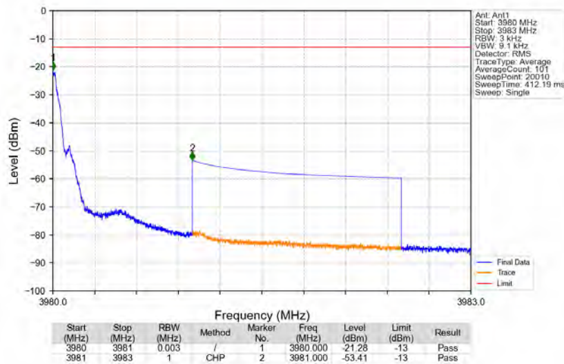
Bandn77a_3979.8MHz_GMSK_SISO_Ant1_NTNV_AGC+3
