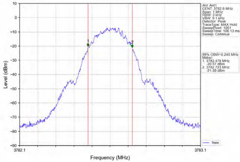
Bandn77a_3782.6MHz_GMSK_SISO_Ant1_NTNV_Input_AGC+3
