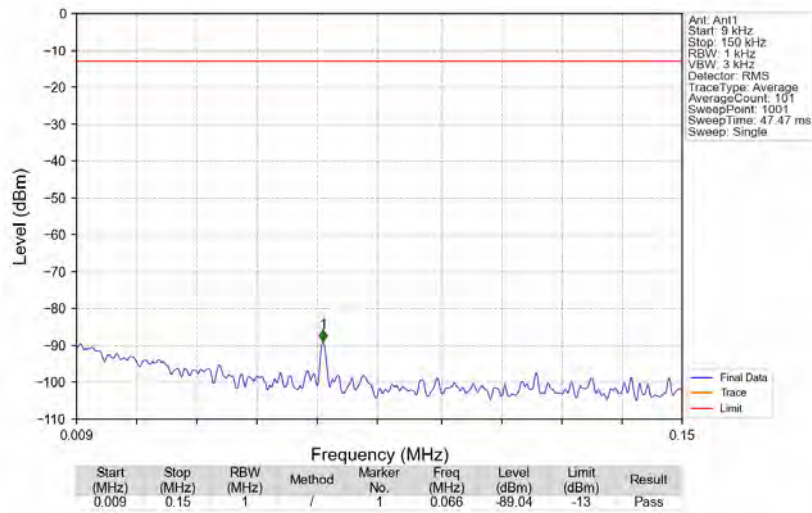
Bandn77a_3840MHz_AWGN_SISO_Ant1_NTNV
