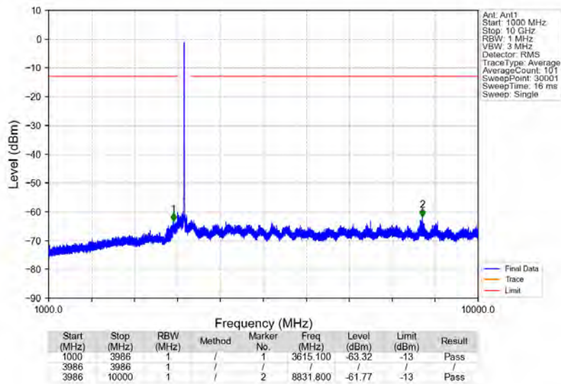
Bandn77a_3840MHz_AWGN_SISO_Ant1_NTNV
