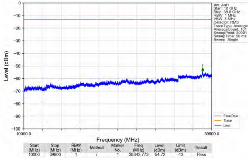
Bandn77a_3977.5MHz_AWGN_SISO_Ant1_NTNV
