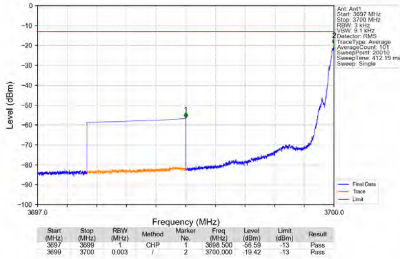
Bandn77a_3700.2MHz_GMSK_SISO_Ant1_NTNV_AGC
