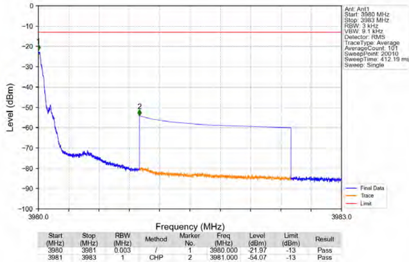
Bandn77a_3979.8MHz_GMSK_SISO_Ant1_NTNV_AGC
