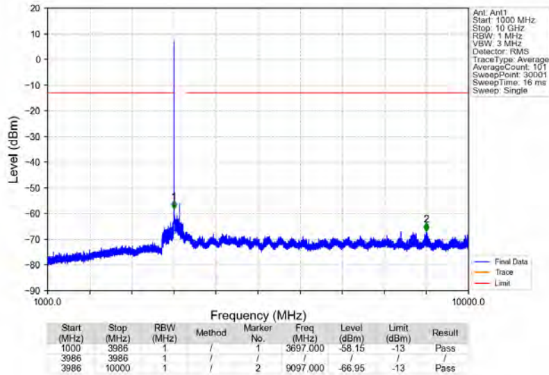
Bandn77a_3700.2MHz_GMSK_SISO_Ant1_NTNV
