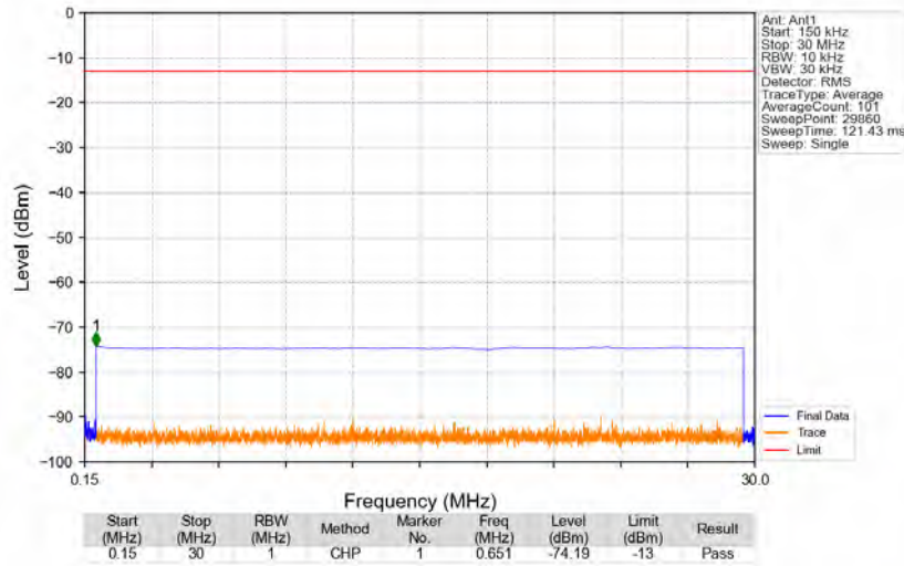
Bandn77a_3840MHz_AWGN_SISO_Ant1_NTNV
