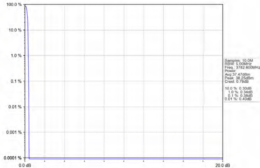
Bandn77a_3782.6MHz_GMSK_SISO_Ant1_NTNV_AGC
