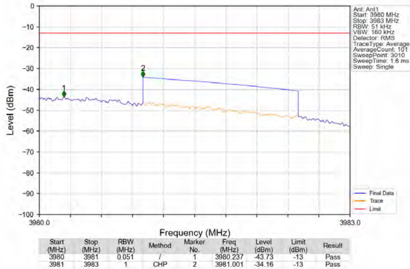
Bandn77a_3977.5MHz_AWGN_SISO_Ant1_NTNV_AGC
