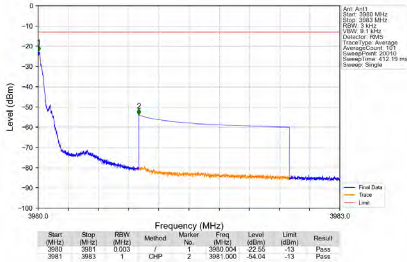
Bandn77a_3979.8MHz_GMSK_SISO_Ant1_NTNV_AGC
