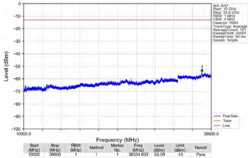
Bandn77a_3840MHz_GMSK_SISO_Ant1_NTNV
