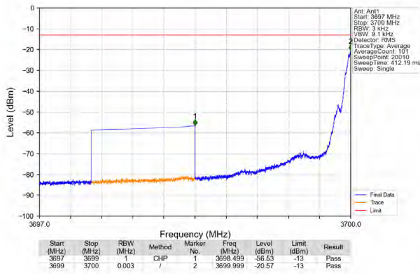
Bandn77a_3700.2MHz_GMSK_SISO_Ant1_NTNV_AGC+3
