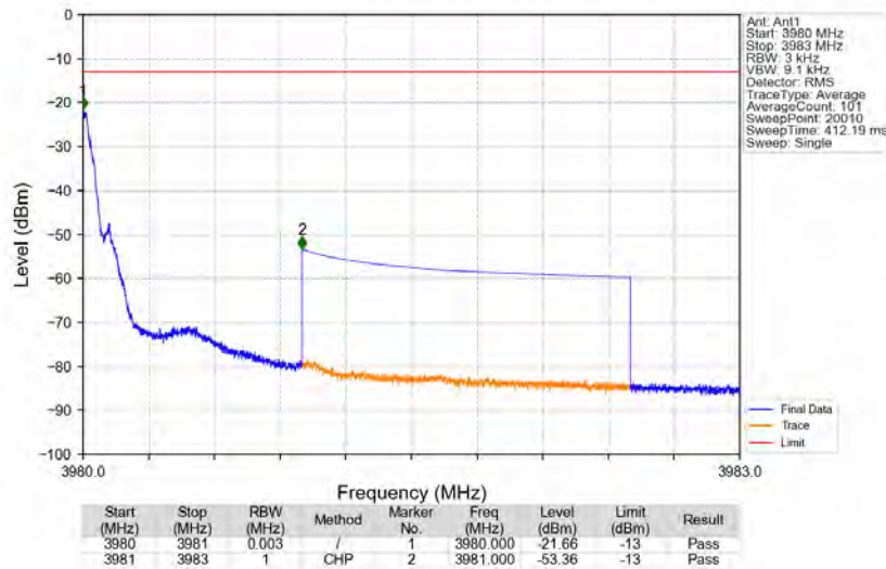
Bandn77a_3979.8MHz_GMSK_SISO_Ant1_NTNV_AGC+3
