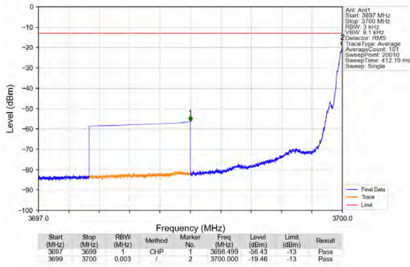
Bandn77a_3700.2MHz_GMSK_SISO_Ant1_NTNV_AGC+3
