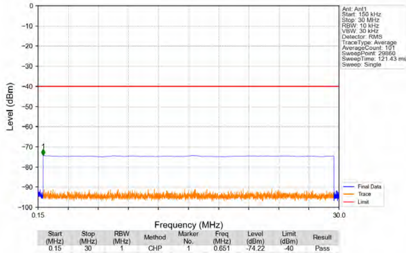
Bandn78e_3500MHz_AWGN_SISO_Ant1_NTNV
