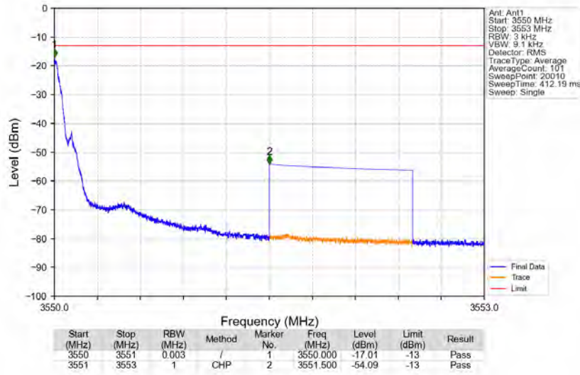
Bandn78e_3549.8MHz_GMSK_SISO_Ant1_NTNV_AGC
