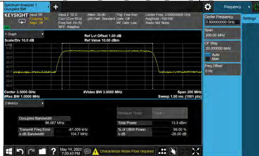
Bandn78e_3500MHz_AWGN_SISO_Ant1_NTNV_Input_AGC+3
