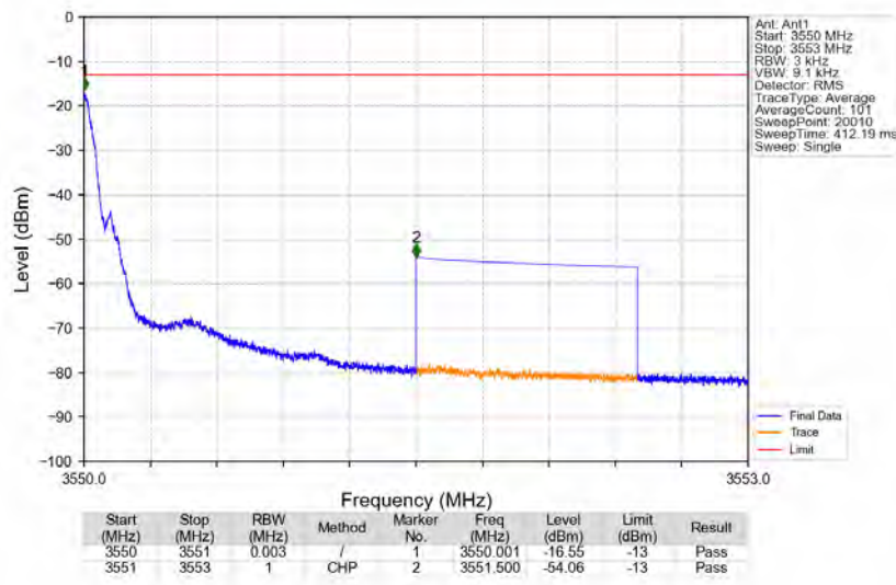
Bandn78e_3549.8MHz_GMSK_SISO_Ant1_NTNV_AGC+3
