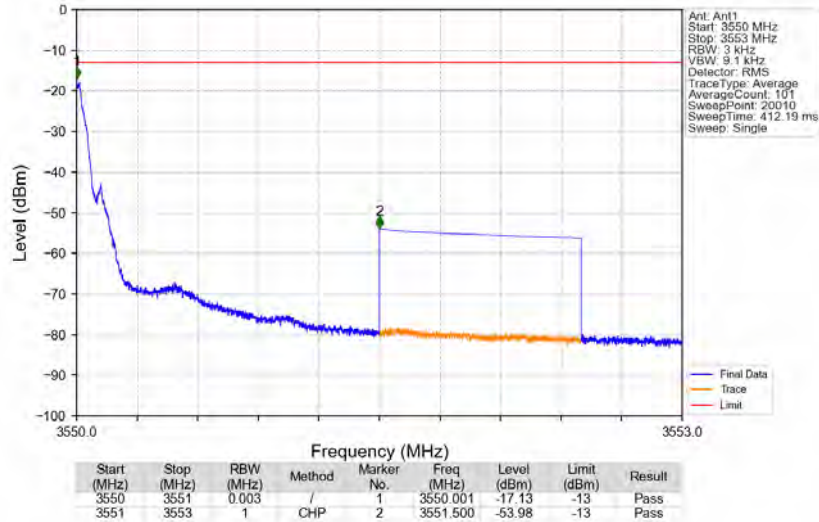
Bandn78e_3549.8MHz_GMSK_SISO_Ant1_NTNV_AGC
