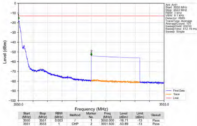
Bandn78e_3549.8MHz_GMSK_SISO_Ant1_NTNV_AGC+3
