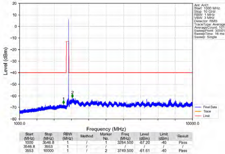
Bandn78e_3549.8MHz_GMSK_SISO_Ant1_NTNV
