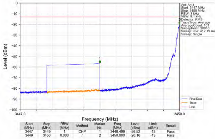
Bandn78e_3450.2MHz_GMSK_SISO_Ant1_NTNV_AGC
