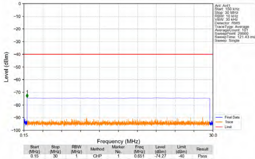
Bandn78e_3450.2MHz_GMSK_SISO_Ant1_NTNV
