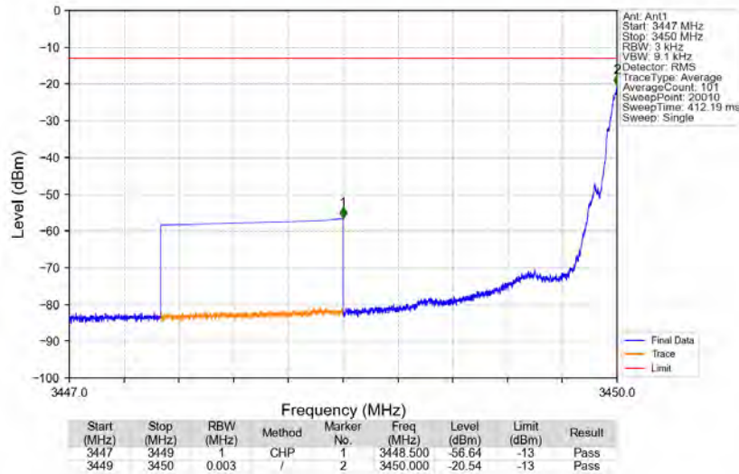
Bandn78e_3450.2MHz_GMSK_SISO_Ant1_NTNV_AGC
