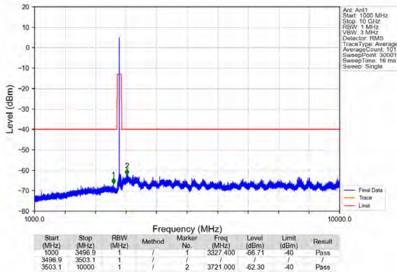
Bandn78e_3500MHz_GMSK_SISO_Ant1_NTNV
