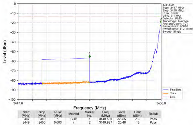
Bandn78e_3450.2MHz_GMSK_SISO_Ant1_NTNV_AGC+3
