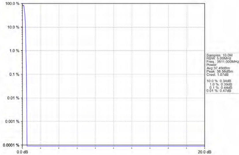
Bandn78e_3511MHz_GMSK_SISO_Ant1_NTNV_AGC
