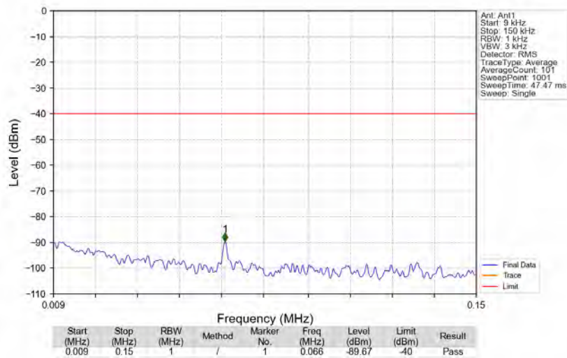
Bandn78e_3450.2MHz_GMSK_SISO_Ant1_NTNV
