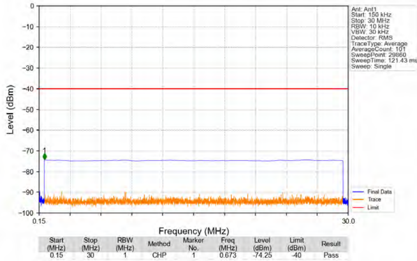
Bandn78e_3549.8MHz_GMSK_SISO_Ant1_NTNV
