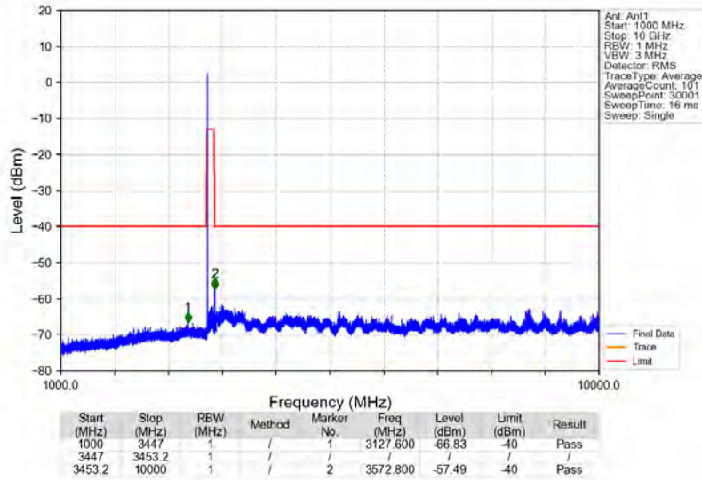
Bandn78e_3450.2MHz_GMSK_SISO_Ant1_NTNV
