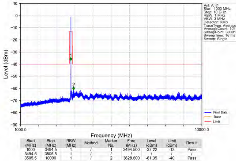
Bandn78e_3500MHz_AWGN_SISO_Ant1_NTNV
