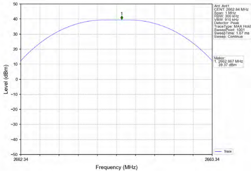
Band41_2662.84MHz_GMSK_SISO_Ant1_NTNV_AGC+3
