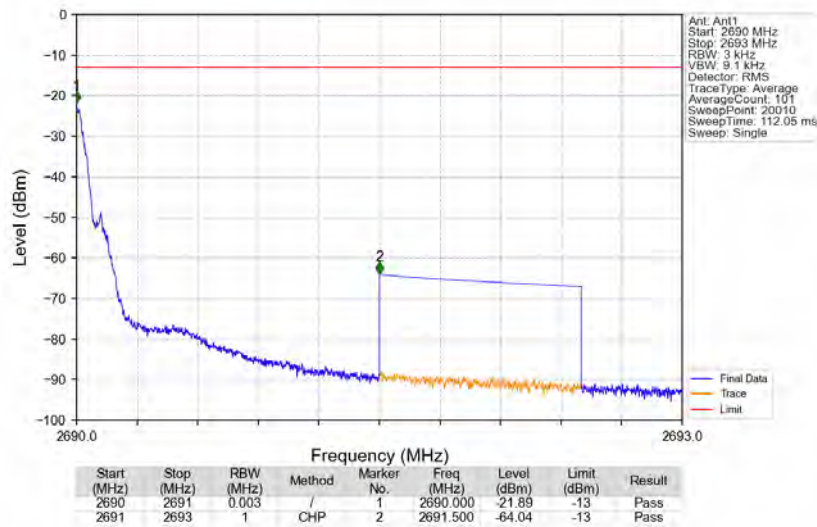
Band41_2689.8MHz_GMSK_SISO_Ant1_NTNV_AGC+3
