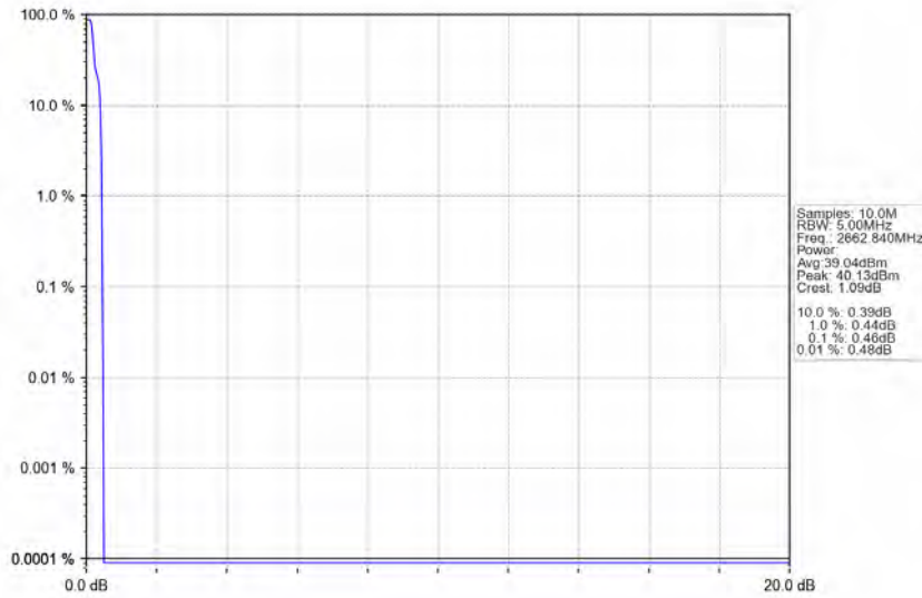
Band41_2662.84MHz_GMSK_SISO_Ant1_NTNV_AGC
