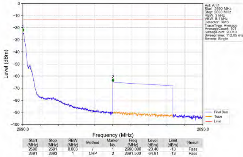
Band41_2689.8MHz_GMSK_SISO_Ant1_NTNV_AGC
