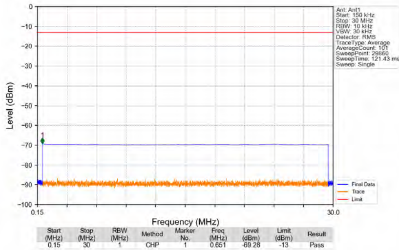
Band41_2689.8MHz_GMSK_SISO_Ant1_NTNV
