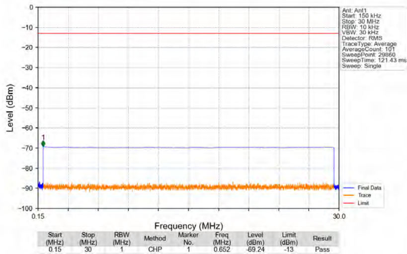
Band41_2687.5MHz_AWGN_SISO_Ant1_NTNV
