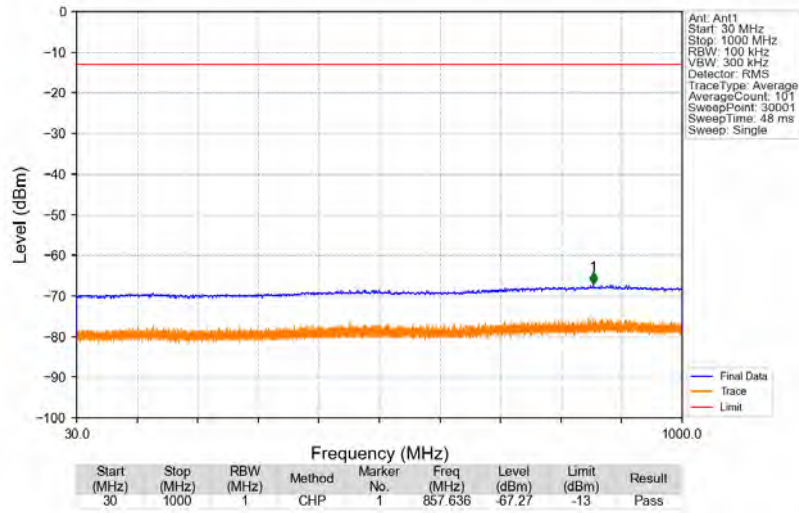
Band41_2593MHz_GMSK_SISO_Ant1_NTNV
