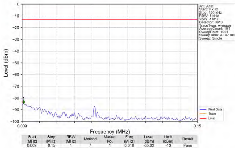
Band41_2593MHz_AWGN_SISO_Ant1_NTNV
