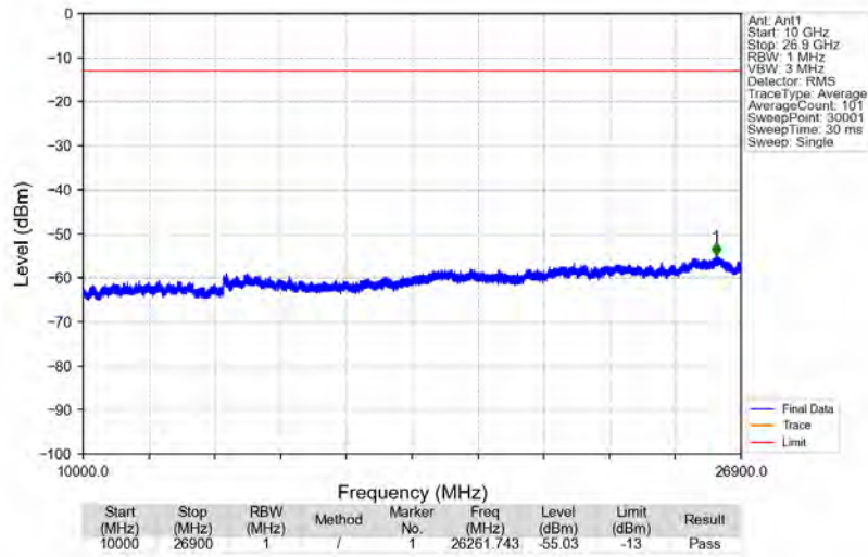
Band41_2593MHz_AWGN_SISO_Ant1_NTNV
