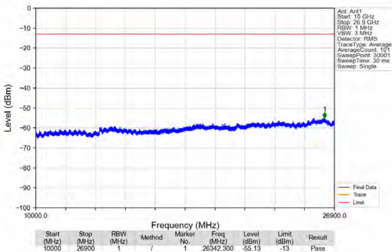
Band41_2496.2MHz_GMSK_SISO_Ant1_NTNV
