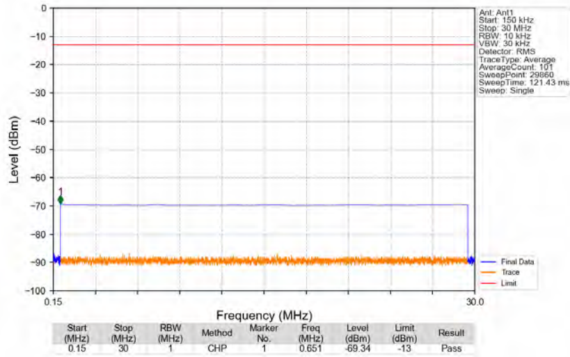
Band41_2593MHz_AWGN_SISO_Ant1_NTNV
