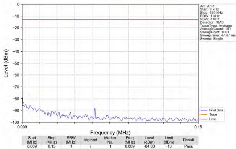
Band41_2496.2MHz_GMSK_SISO_Ant1_NTNV
