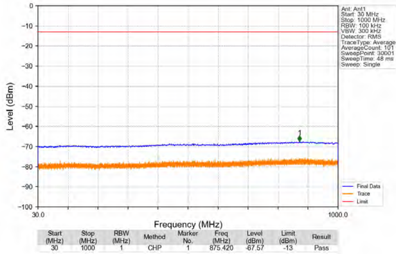
Band41_2687.5MHz_AWGN_SISO_Ant1_NTNV
