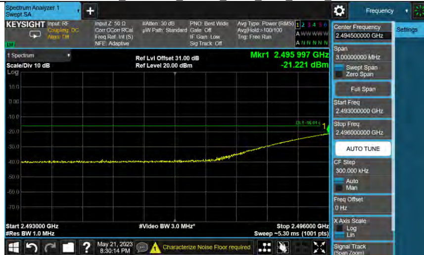
Band41_2546MHz_AWGN_SISO_Ant1_NTNV_AGC+3
