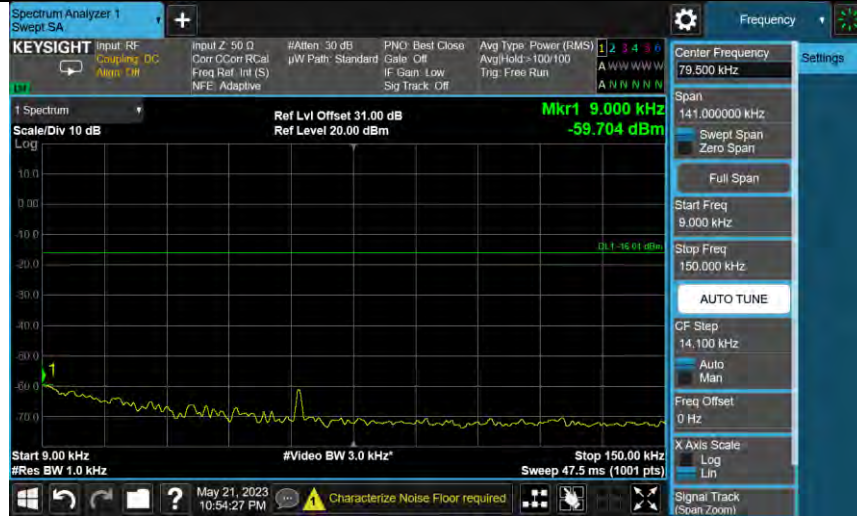
Band41_2640MHz_AWGN_SISO_Ant1_NTNV
