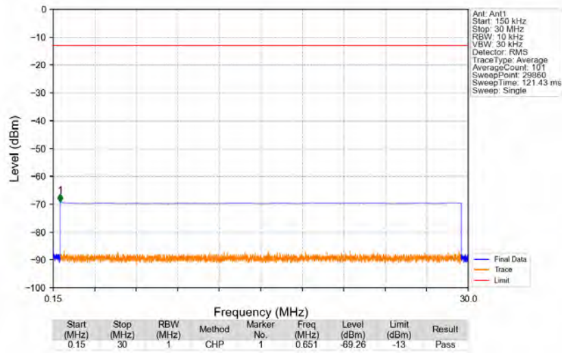
Band41_2496.2MHz_GMSK_SISO_Ant1_NTNV
