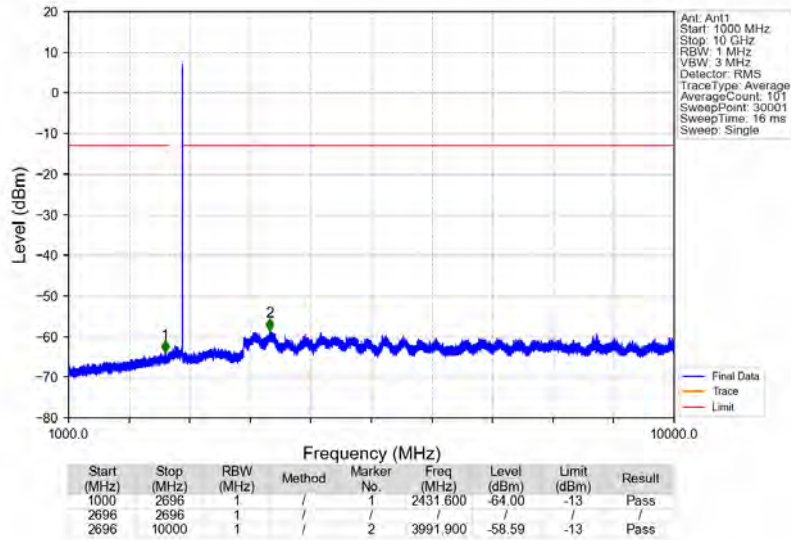
Band41_2689.8MHz_GMSK_SISO_Ant1_NTNV
