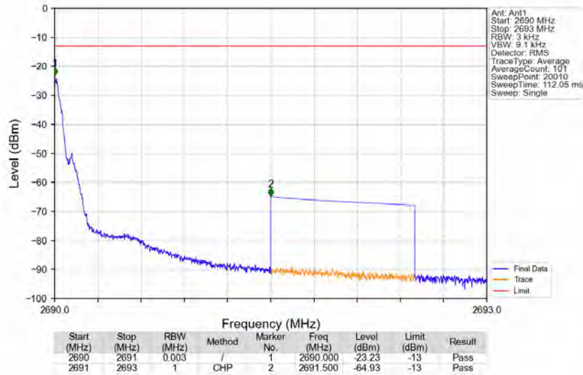
Band41_2689.8MHz_GMSK_SISO_Ant1_NTNV_AGC
