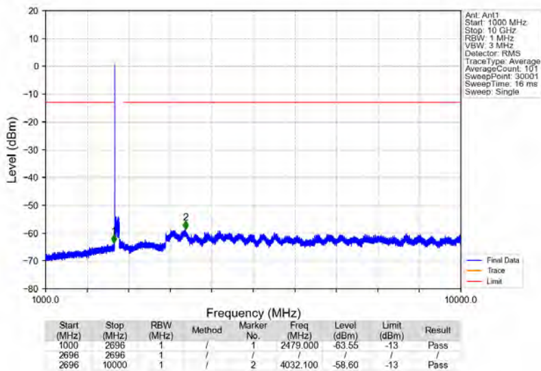
Band41_2496.2MHz_GMSK_SISO_Ant1_NTNV
