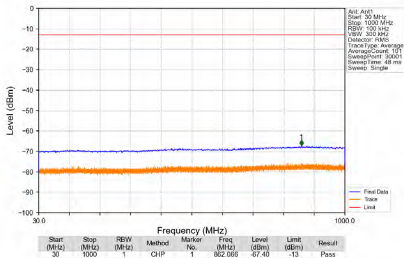
Band41_2689.8MHz_GMSK_SISO_Ant1_NTNV
