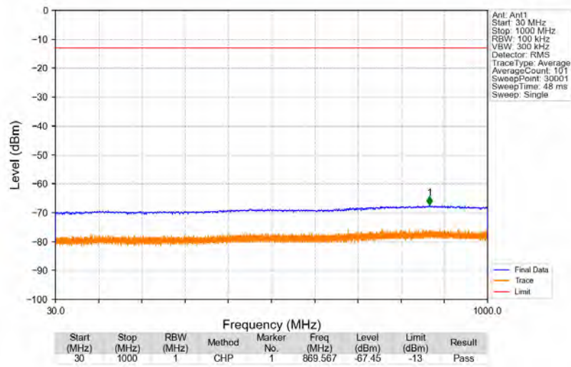
Band41_2496.2MHz_GMSK_SISO_Ant1_NTNV
