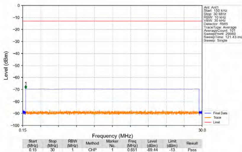
Band41_2593MHz_GMSK_SISO_Ant1_NTNV
