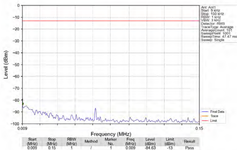
Band41_2689.8MHz_GMSK_SISO_Ant1_NTNV
