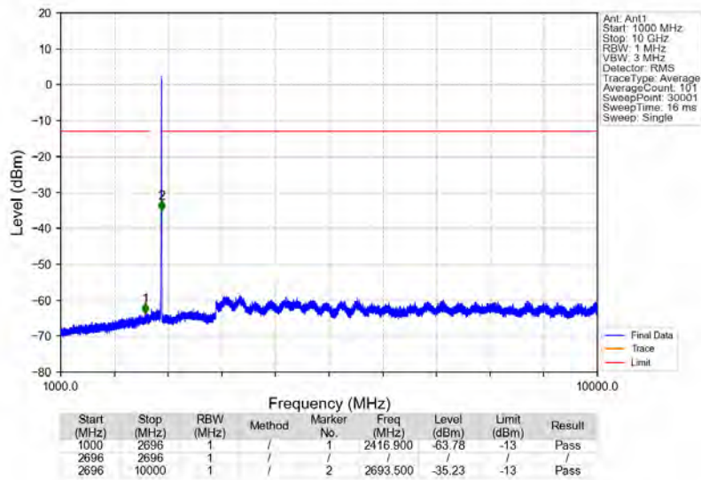
Band41_2687.5MHz_AWGN_SISO_Ant1_NTNV
