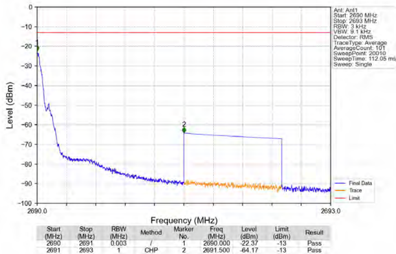
Band41_2689.8MHz_GMSK_SISO_Ant1_NTNV_AGC+3
