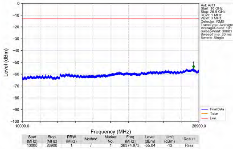
Band41_2498.5MHz_AWGN_SISO_Ant1_NTNV
