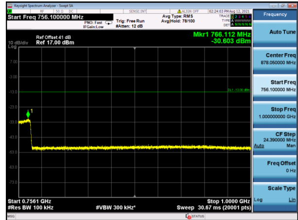
756.1-1000MHz
