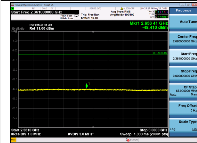
2361-3000MHz
