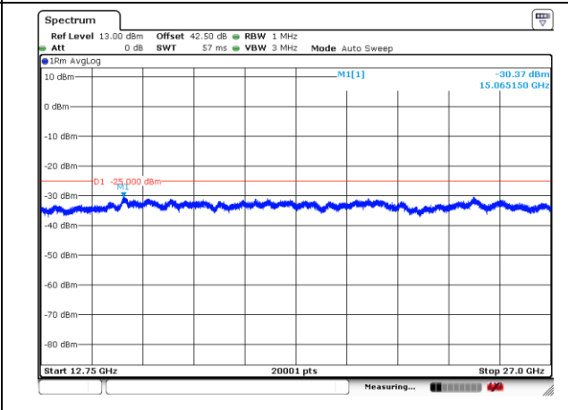
12750-27000MHz
