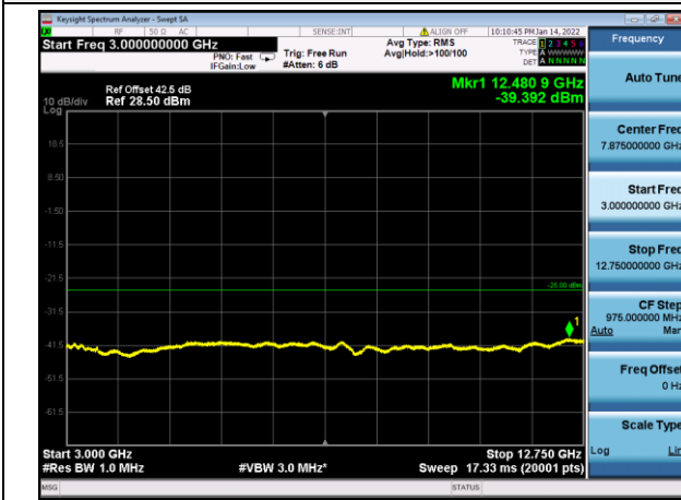
3000-12750MHz
