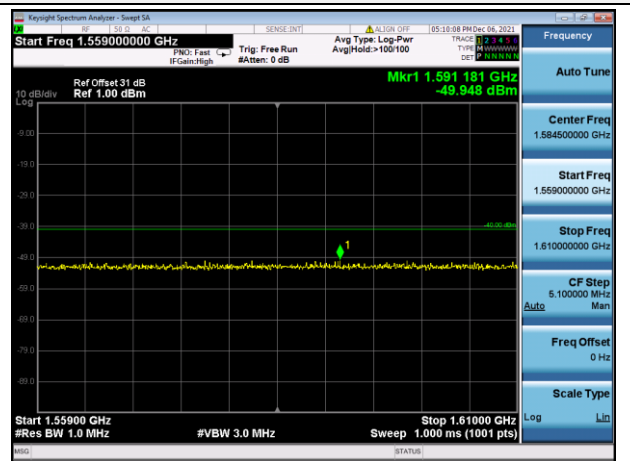
1559-1610MHz
