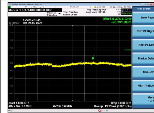
1-9GHz
