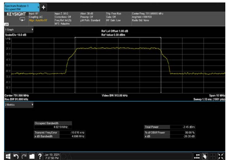
Figure 248: 256QAM 5MHz; 751.5MHz B.W, 30kHz INPUT
