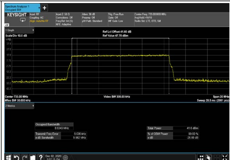
Figure 360: 64QAM 10MHz B.W; 733.0MHz output 4G
