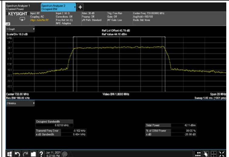
Figure 308: 256QAM 10MHz B.W; 733.0MHz, 30kHz OUTPUT
