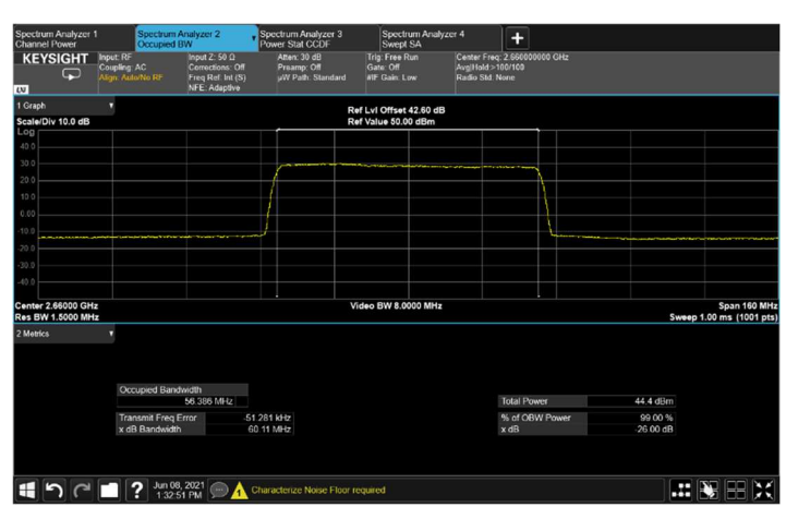
Figure 166: output 64QAM 60MHz B.W.; 2660.0MHz, 60kHz
