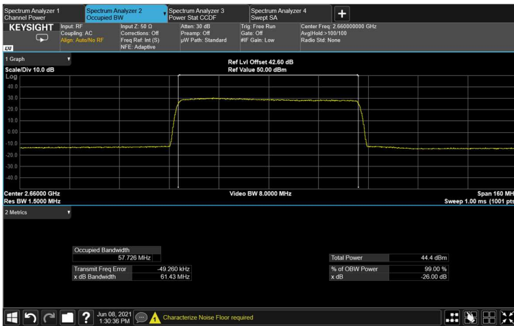
Figure 165: output 64QAM 60MHz B.W.; 2660.0MHz, 30kHz
