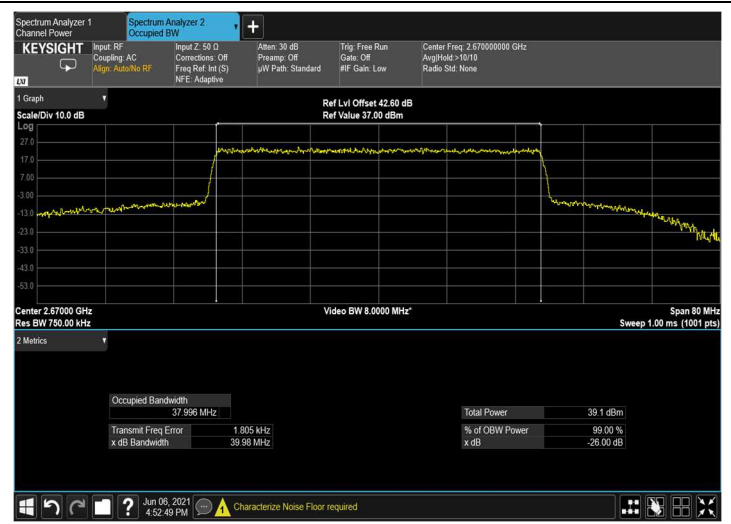
Figure 189: output QPSK 40MHz B.W.; 2670.0MHz, 30kHz
