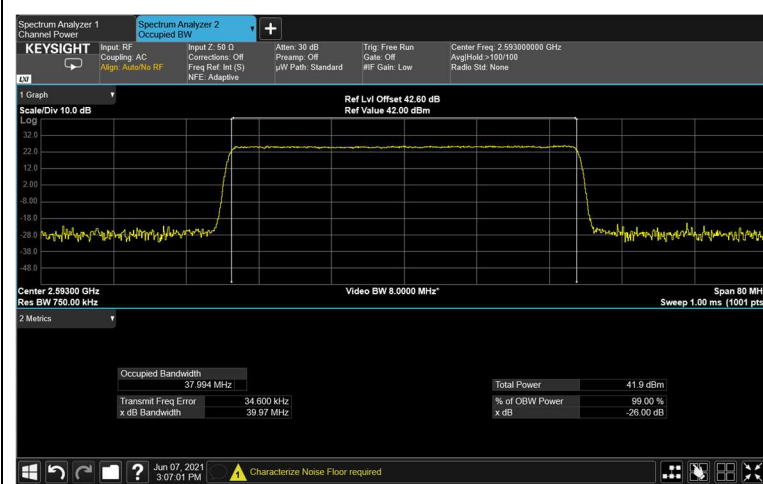
Figure 171: output 256QAM 40MHz B.W.; 2593.0MHz, 30kHz
