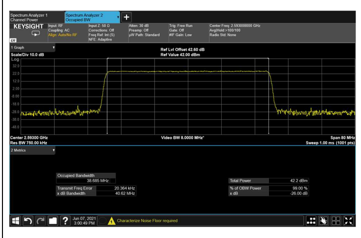
Figure 170: output 256QAM 40MHz B.W.; 2593.0MHz, 15kHz
