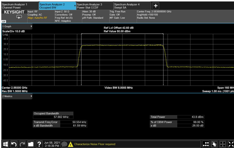
Figure 163: output 64QAM 60MHz B.W.; 2593.0MHz, 30kHz
