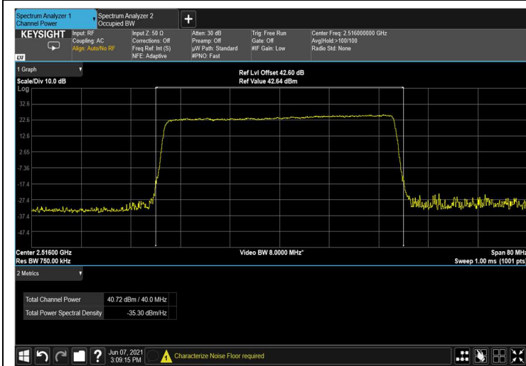
Figure 40: 256QAM 40MHz B.W.; 2516.0MHz, 60kHz
