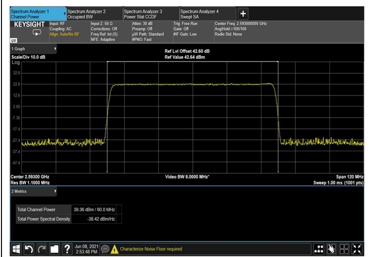
Figure 50: 256QAM 60MHz B.W.; 2593.0MHz, 60kHz
