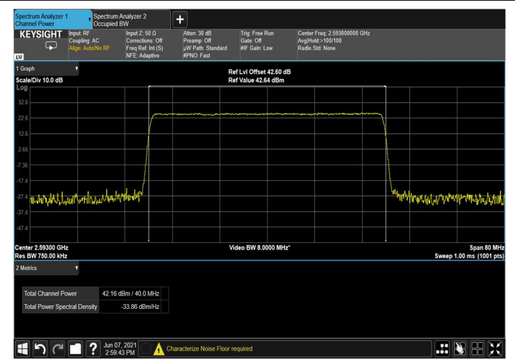
Figure 41: 256QAM 40MHz B.W.; 2593.0MHz, 15kHz
