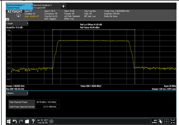
Figure 54: 256QAM 10MHz B.W.; 1962.5MHz, 30kHz
