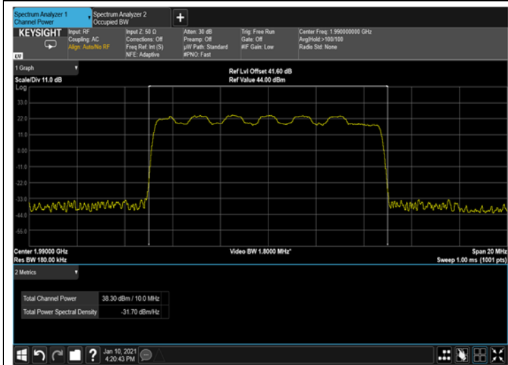
Figure 19: 16QAM 10MHz B.W.; 1990MHz, 15kHz
