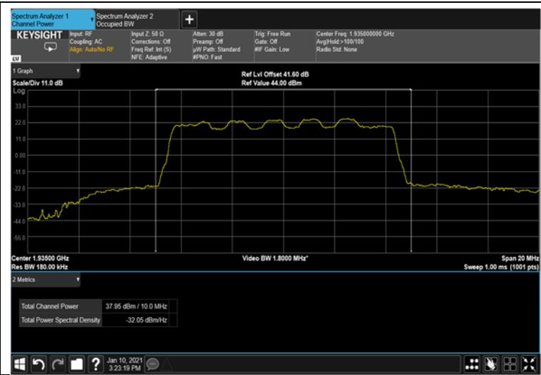
Figure 16: 16QAM 10MHz B.W.; 1935MHz, 30kHz
