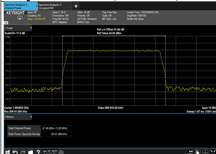
Figure 49: 256QAM 5MHz B.W.; 1992.5MHz, 15kHz
