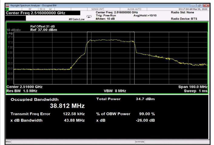
Figure 378: 64QAM 40MHz B.W.; 2516.0MHz, 15kHz Output
