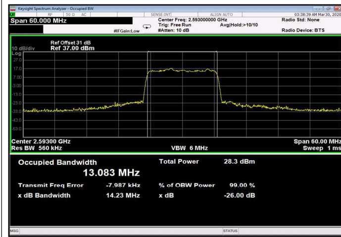
Figure 365: 64QAM 15MHz B.W.; 2593.0MHz, 60kHz Output
