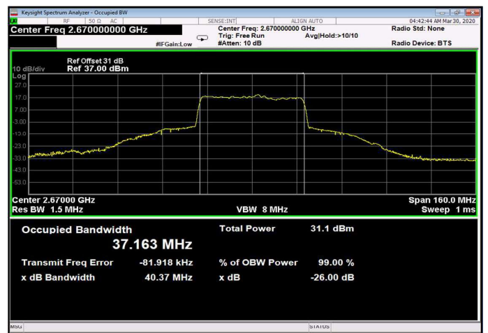
Figure 386: 64QAM 40MHz B.W.; 2670.0MHz, 60kHz Output
