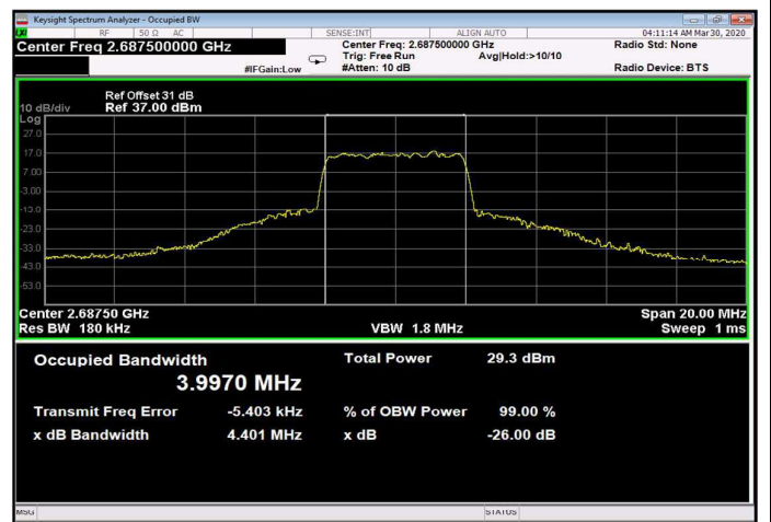
Figure 350: 64QAM 5MHz B.W.; 2687.5MHz, 30kHz Output
