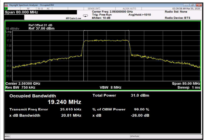
Figure 372: 64QAM 20MHz B.W.; 2593.0MHz, 15kHz Output
