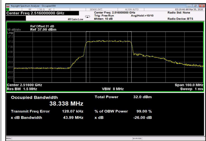
Figure 379: 64QAM 40MHz B.W.; 2516.0MHz, 30kHz Output
