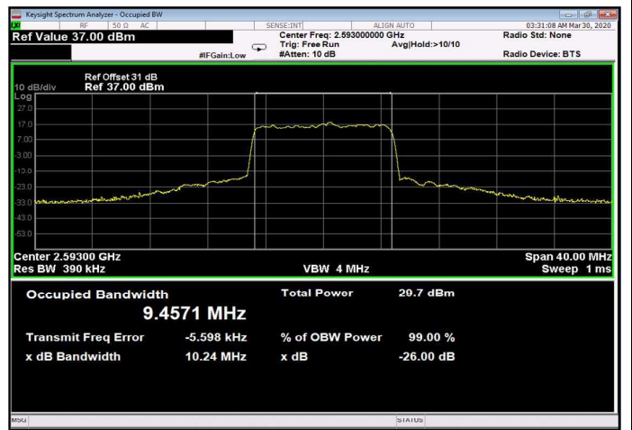
Figure 354: 64QAM 10MHz B.W.; 2593.0MHz, 15kHz Output
