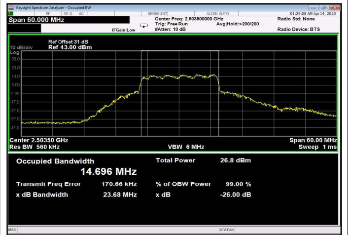
Figure 312: 16QAM 15MHz B.W.; 2503.5MHz, 15kHz Output
