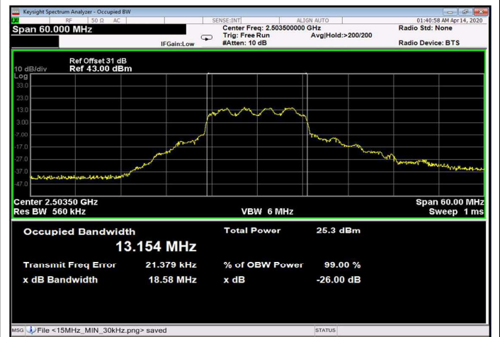
Figure 314: 16QAM 15MHz B.W.; 2503.5MHz, 60kHz Output
