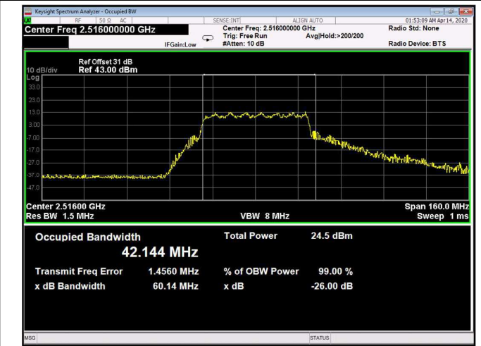
Figure 330: 16QAM 40MHz B.W.; 2516.0MHz, 15kHz Output
