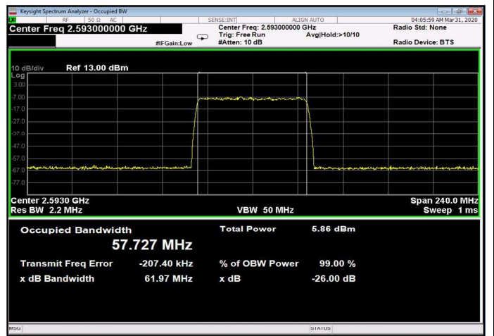
Figure 294: 256QAM 60MHz B.W.; 2593.0MHz, 60kHz Input
