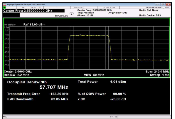
Figure 296: 256QAM 60MHz B.W.; 2660.0MHz, 60kHz Input
