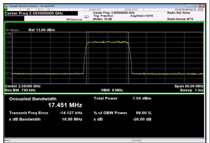
Figure 278: 256QAM 20MHz B.W.; 2593.0MHz, 60kHz Input
