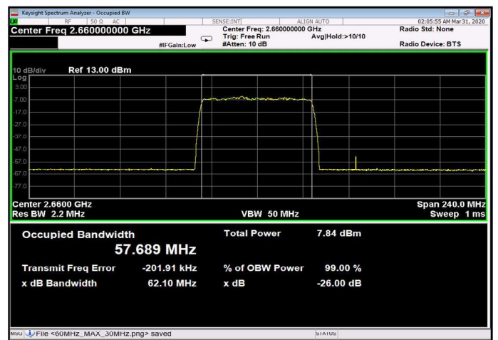
Figure 248: 64QAM 60MHz B.W.; 2660.0MHz, 60kHz Input
