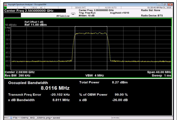
Figure 212: 64QAM 10MHz B.W.; 2593.0MHz, 60kHz Input
