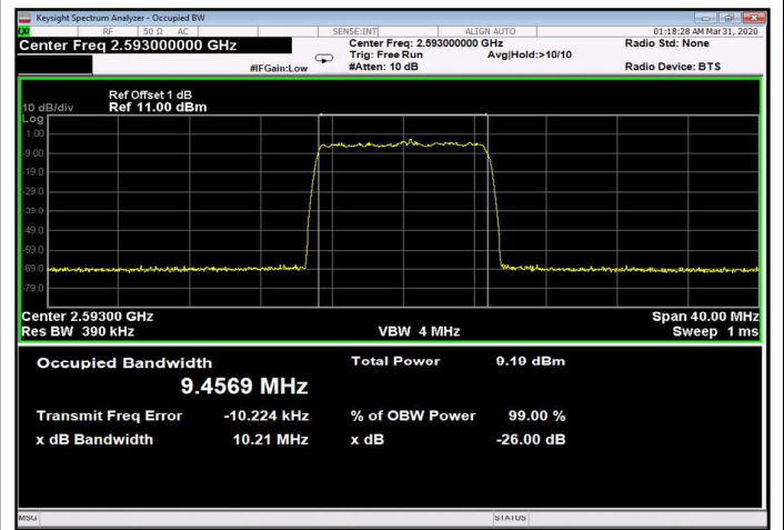
Figure 210: 64QAM 10MHz B.W.; 2593.0MHz, 15kHz Input
