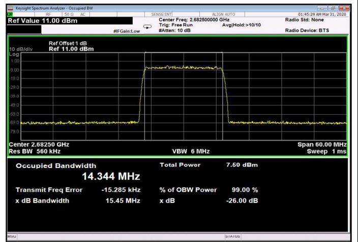
Figure 222: 64QAM 15MHz B.W.; 2682.5MHz, 15kHz Input
