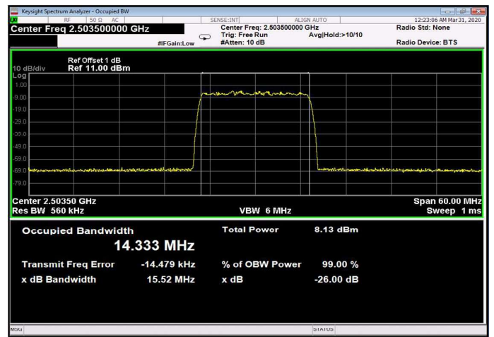
Figure 216: 64QAM 15MHz B.W.; 2503.5MHz, 15kHz Input
