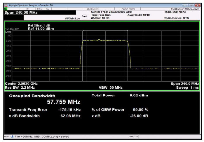
Figure 246: 64QAM 60MHz B.W.; 2593.0MHz, 60kHz Input
