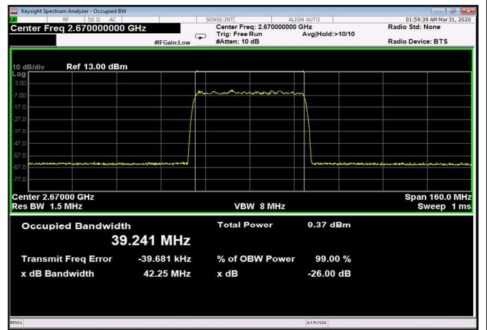
Figure 240: 64QAM 40MHz B.W.; 2670.0MHz, 15kHz Input
