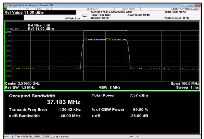
Figure 236: 64QAM 40MHz B.W.; 2516.0MHz, 60kHz Input
