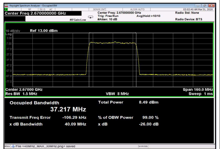
Figure 242: 64QAM 40MHz B.W.; 2670.0MHz, 60kHz Input
