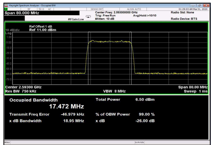
Figure 230: 64QAM 20MHz B.W.; 2593.0MHz, 60kHz Input
