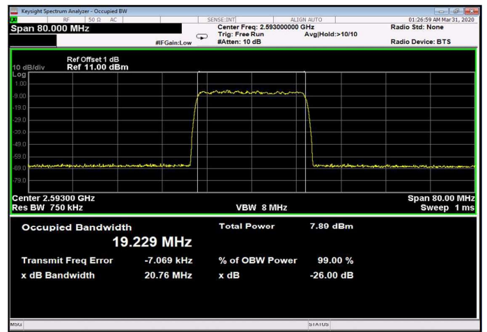
Figure 228: 64QAM 20MHz B.W.; 2593.0MHz, 15kHz Input
