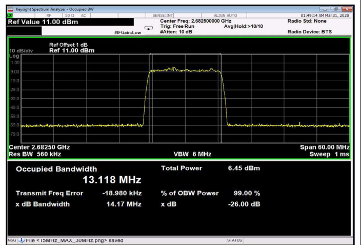
Figure 224: 64QAM 15MHz B.W.; 2682.5MHz, 60kHz Input
