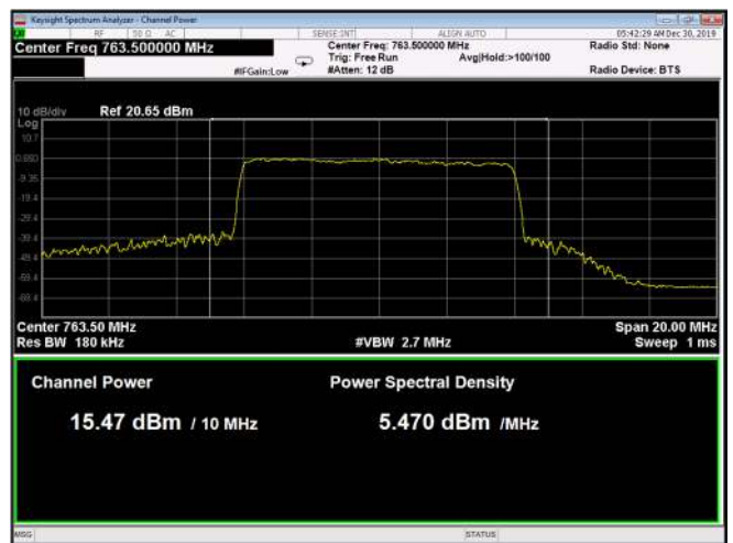
Figure 50: 256QAM 10MHz B.W.; 763.5MHz, 60kHz
