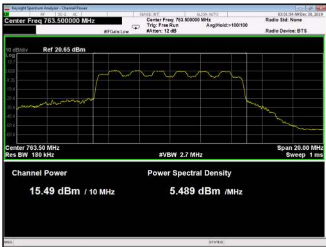
Figure 33: 64QAM 10MHz B.W.; 763.5MHz, 15kHz
