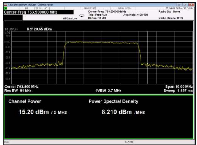
Figure 42: 256QAM 5MHz B.W.; 763.5MHz, 30kHz
