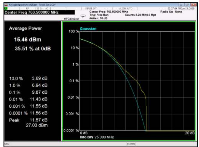
Figure 96: QPSK 10MHz B.W.; 763.5MHz, 60kHz
