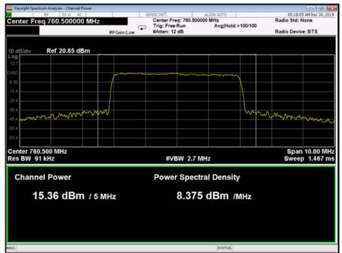
Figure 40: 256QAM 5MHz B.W.; 760.5MHz, 30kHz
