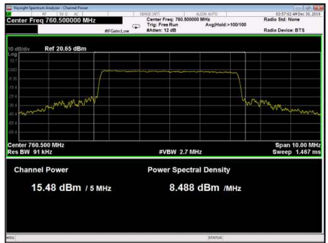
Figure 54: QPSK 5MHz B.W.; 760.5MHz, 15kHz
