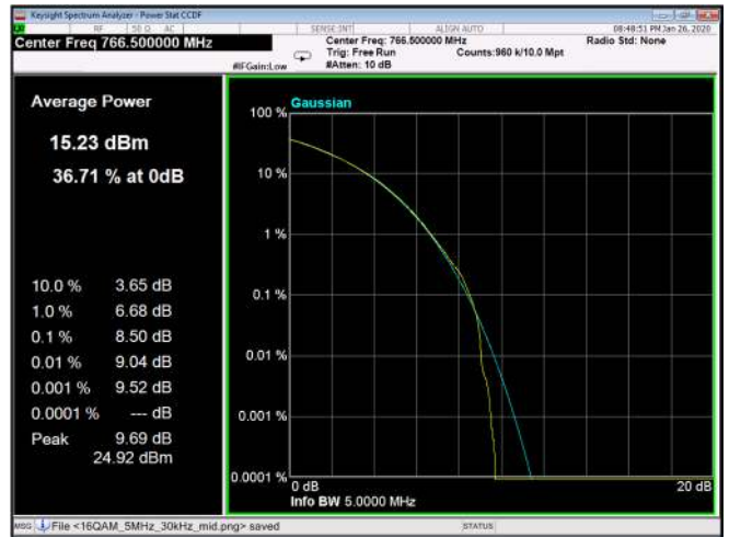
Figure 72: 16QAM 5MHz B.W.; 766.5MHz, 30kHz
