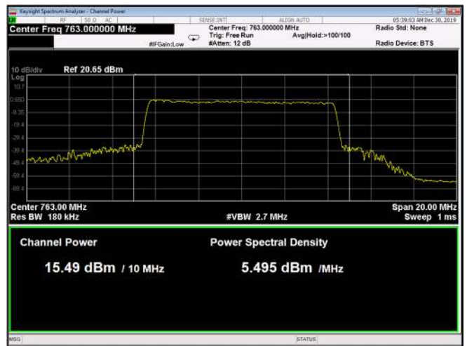
Figure 46: 256QAM 10MHz B.W.; 763.0MHz, 30kHz
