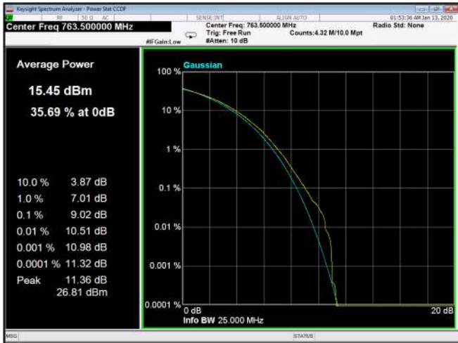
Figure 81: 64QAM 10MHz B.W.; 763.5MHz, 30kHz
