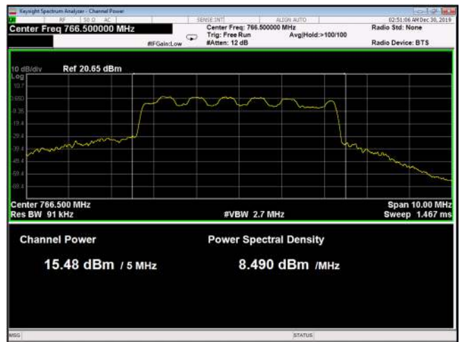
Figure 28: 64QAM 5MHz B.W.; 766.5MHz, 15kHz
