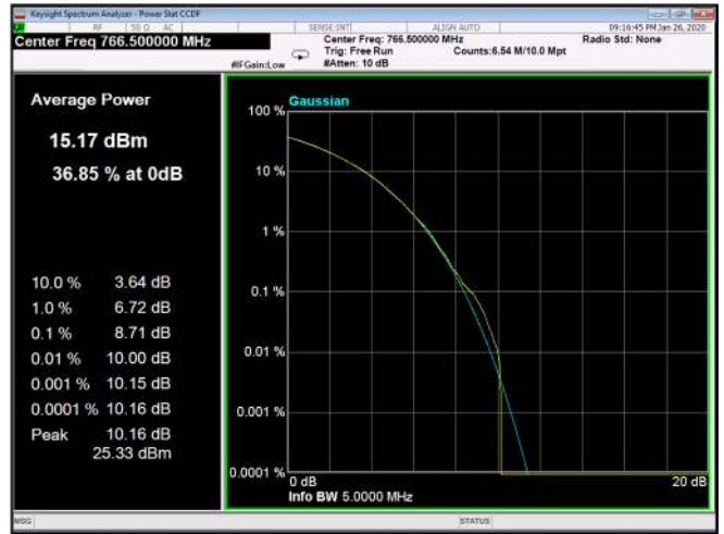
Figure 70: 16QAM 5MHz B.W.; 766.5MHz, 15kHz
