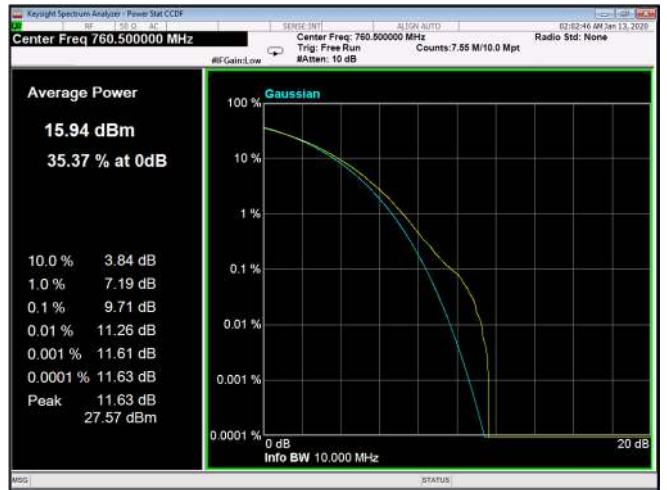
Figure 90: QPSK 5MHz B.W.; 760.5MHz, 15kHz
