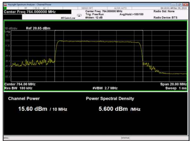
Figure 66: QPSK 10MHz B.W.; 764.0MHz, 15kHz
