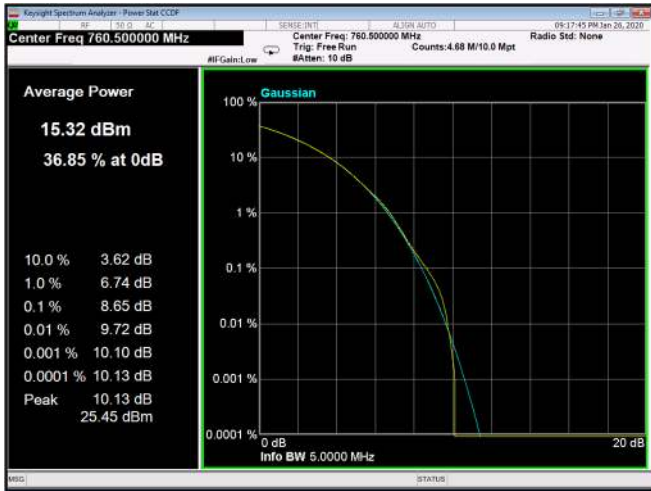
Figure 69: 16QAM 5MHz B.W.; 760.5MHz, 15kHz
