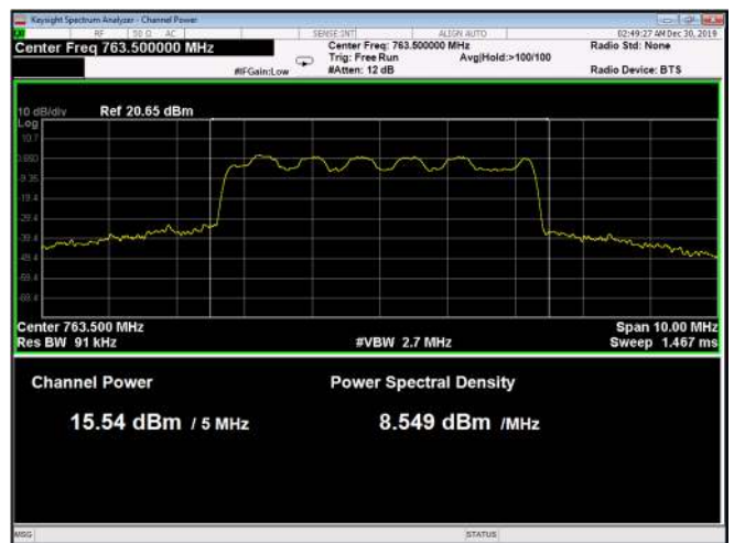
Figure 26: 64QAM 5MHz B.W.; 763.5MHz, 15kHz
