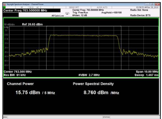
Figure 56: QPSK 5MHz B.W.; 763.5MHz, 15kHz
