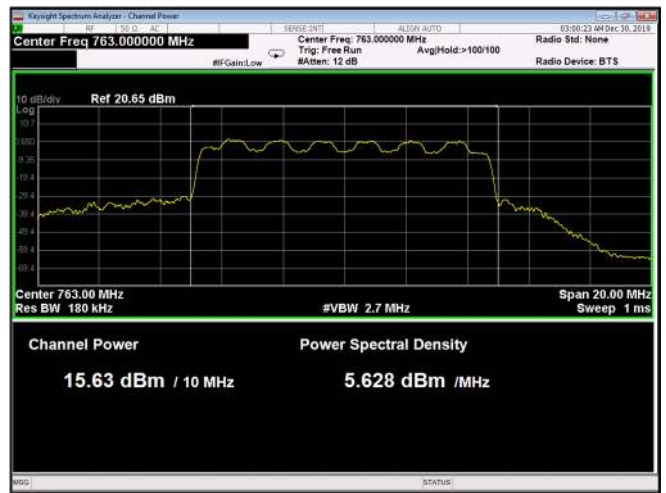
Figure 30: 64QAM 10MHz B.W.; 763.0MHz, 15kHz
