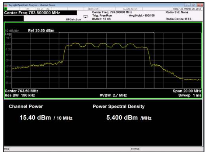
Figure 34: 64QAM 10MHz B.W.; 763.5MHz, 30kHz
