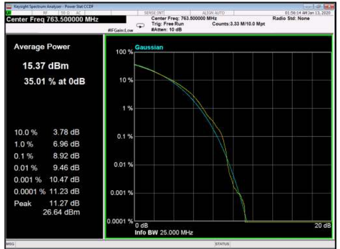
Figure 82: 64QAM 10MHz B.W.; 763.5MHz, 60kHz
