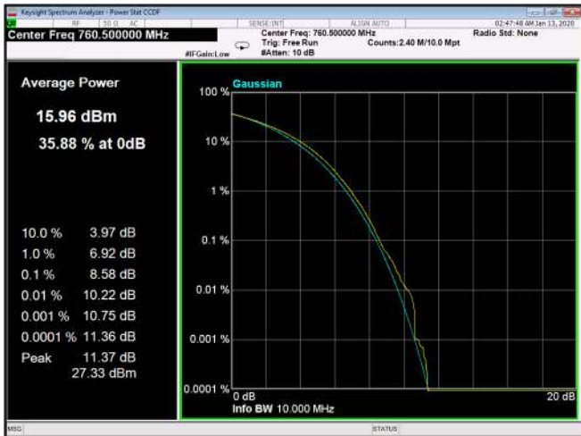
Figure 83: 256QAM 5MHz B.W.; 760.5MHz, 15kHz
