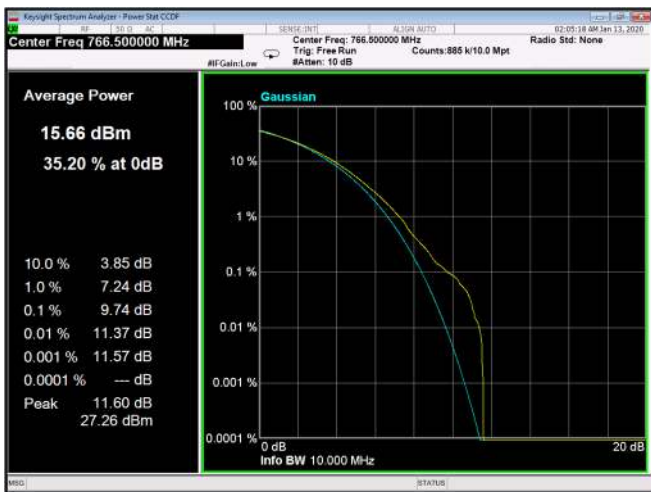
Figure 91: QPSK 5MHz B.W.; 766.5MHz, 15kHz
