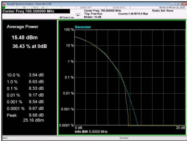
Figure 71: 16QAM 5MHz B.W.; 760.5MHz, 30kHz
