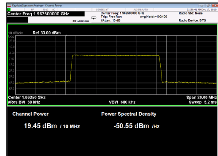
Figure 217: QPSK 10MHz B.W.; 1962.5MHz, 30kHz
