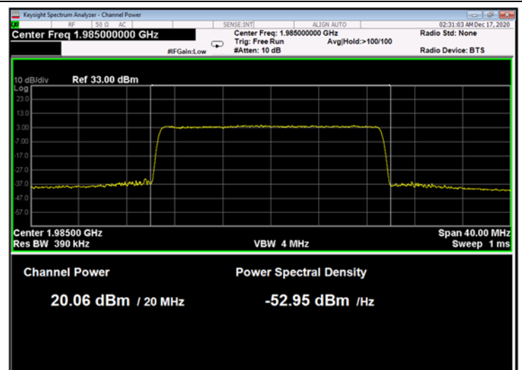
Figure 238: QPSK 20MHz B.W.; 1985.0MHz, 30kHz
