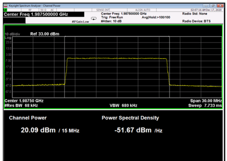
Figure 228: QPSK 15MHz B.W.; 1987.5MHz, 15kHz
