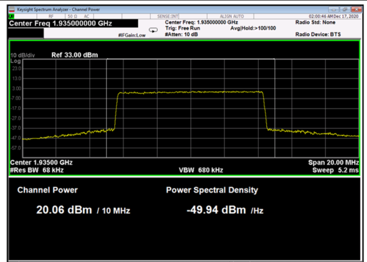
Figure 214: QPSK 10MHz B.W.; 1935.0MHz, 30kHz
