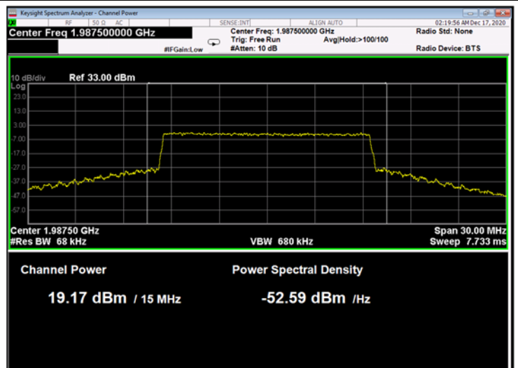
Figure 230: QPSK 15MHz B.W.; 1987.5MHz, 60kHz
