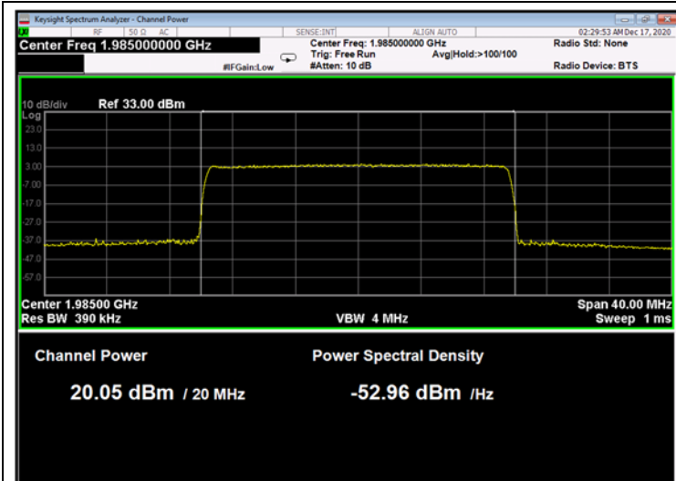
Figure 237: QPSK 20MHz B.W.; 1985.0MHz, 15kHz
