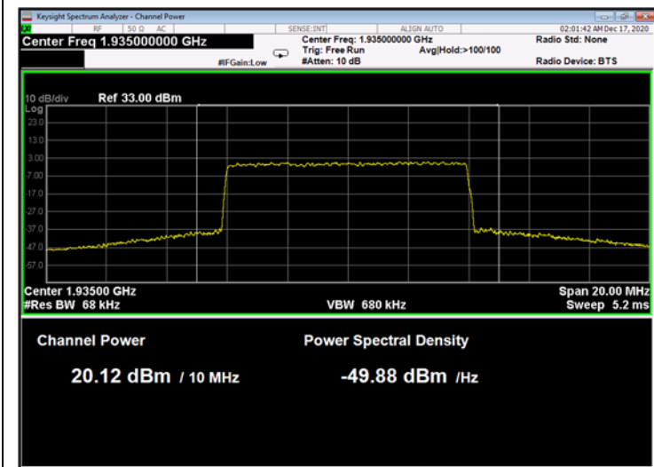
Figure 215: QPSK 10MHz B.W.; 1935.0MHz, 60kHz
