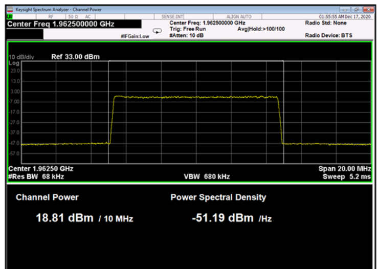
Figure 216: QPSK 10MHz B.W.; 1962.5MHz, 15kHz
