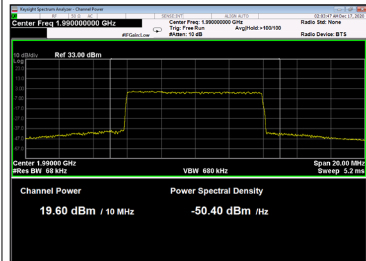
Figure 221: QPSK 10MHz B.W.; 1990.0MHz, 60kHz
