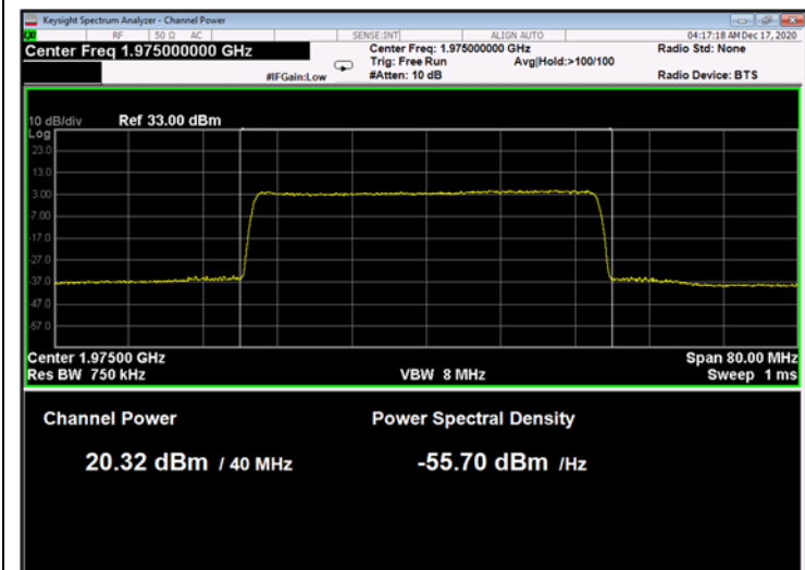
Figure 257: QPSK 40MHz B.W.; 1975.0MHz, 60kHz
