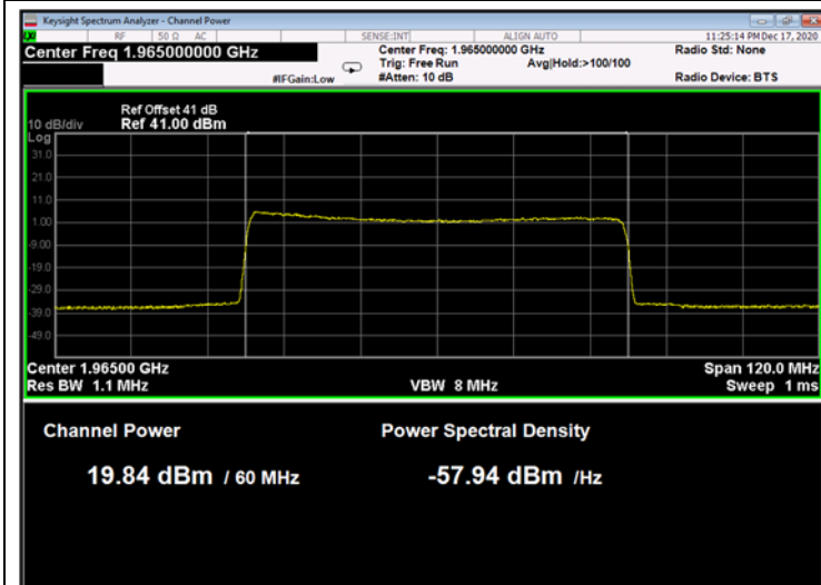
Figure 205: 256QAM 60MHz B.W.; 1965.0MHz, 30kHz
