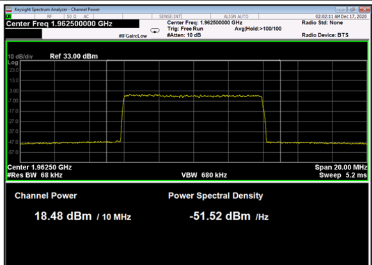
Figure 218: QPSK 10MHz B.W.; 1962.5MHz, 60kHz
