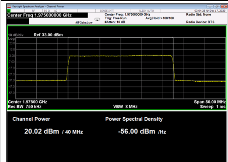
Figure 255: QPSK 40MHz B.W.; 1975.0MHz, 15kHz
