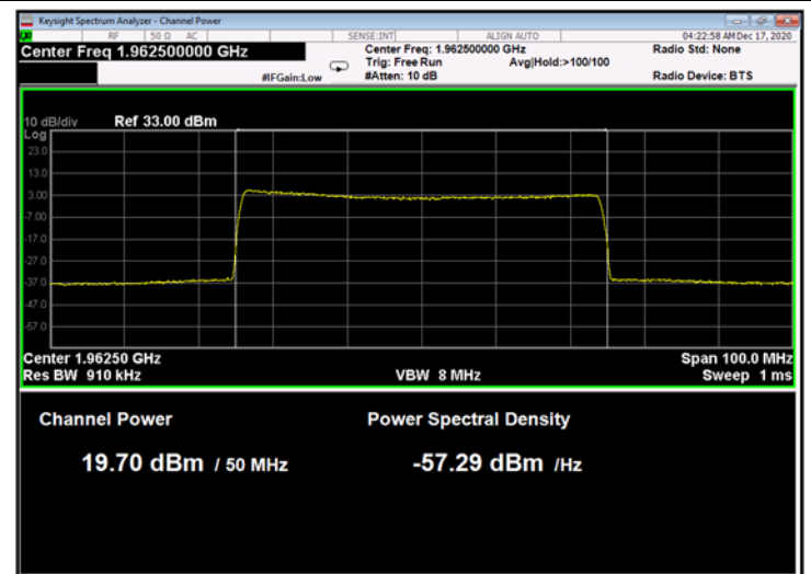
Figure 262: QPSK 50MHz B.W.; 1962.5MHz, 30kHz
