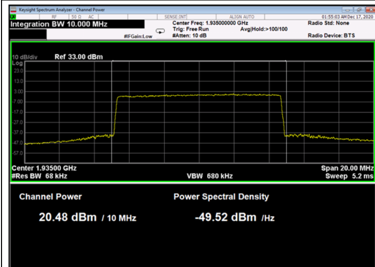
Figure 213: QPSK 10MHz B.W.; 1935.0MHz, 15kHz
