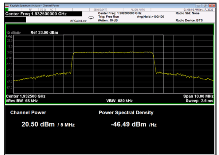
Figure 208: QPSK 5MHz B.W.; 1932.5MHz, 30kHz
