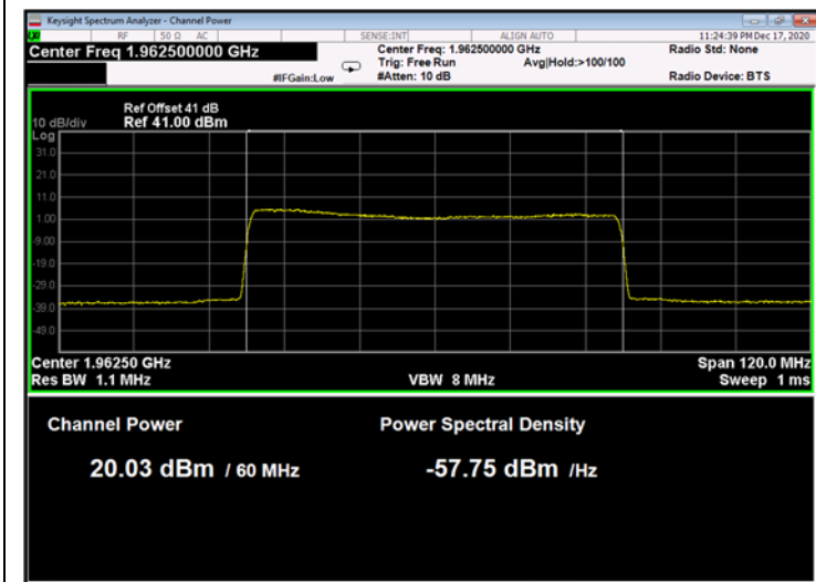
Figure 203: 256QAM 60MHz B.W.; 1962.5MHz, 30kHz
