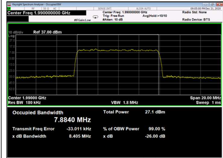
Figure 683: 256QAM 10MHz B.W.; 1990.0MHz, 60kHz - Output
