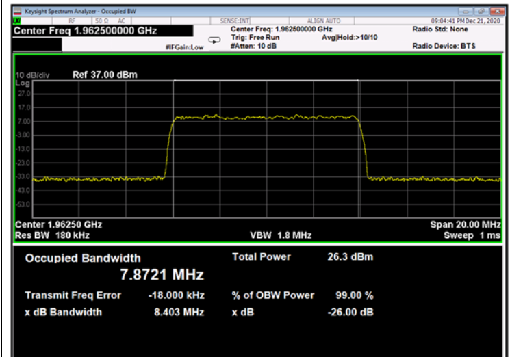
Figure 680: 256QAM 10MHz B.W.; 1962.5MHz, 60kHz - Output
