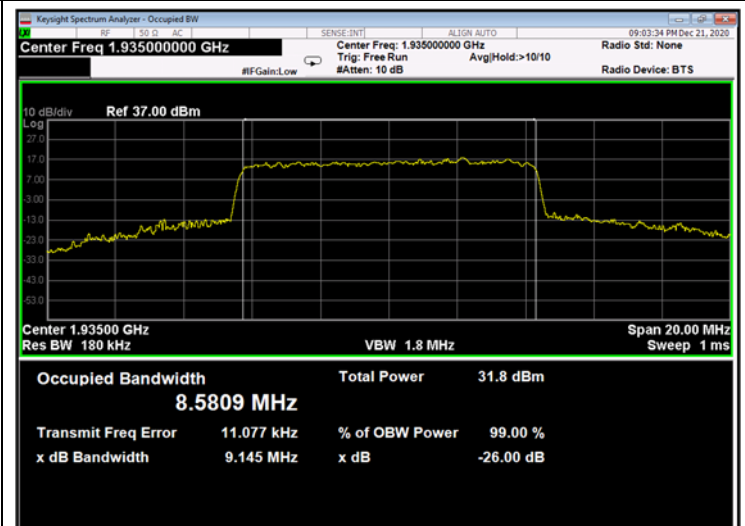
Figure 676: 256QAM 10MHz B.W.; 1935.0MHz, 30kHz - Output
