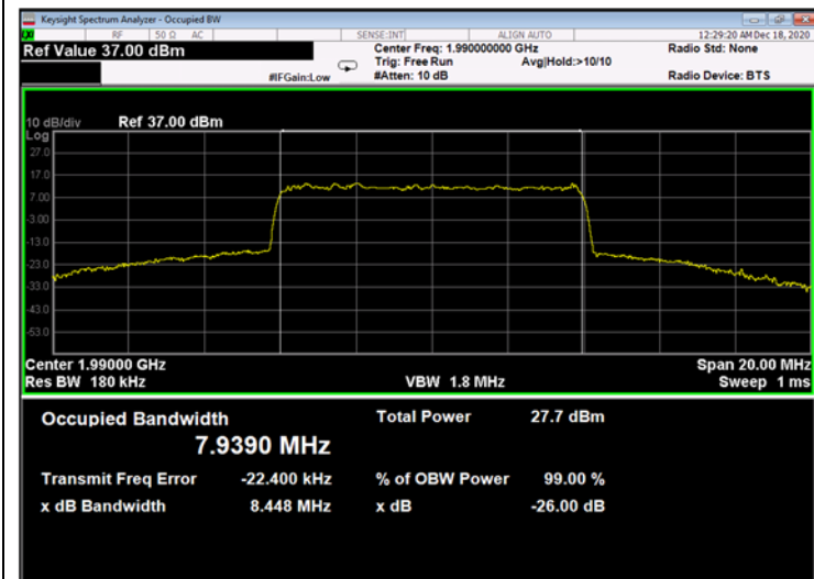
Figure 749: QPSK 10MHz B.W.; 1990.0MHz, 60kHz - Output
