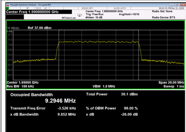
Figure 681: 256QAM 10MHz B.W.; 1990.0MHz, 15kHz - Output
