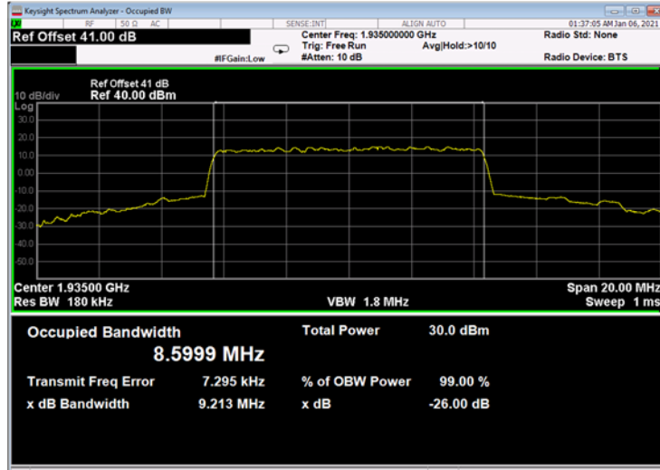
Figure 742: QPSK 10MHz B.W.; 1935.0MHz, 30kHz - Output
