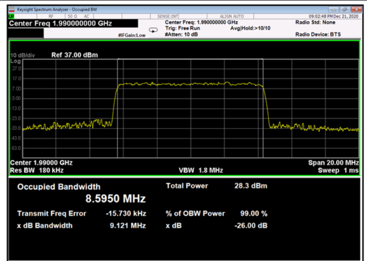
Figure 682: 256QAM 10MHz B.W.; 1990.0MHz, 30kHz - Output
