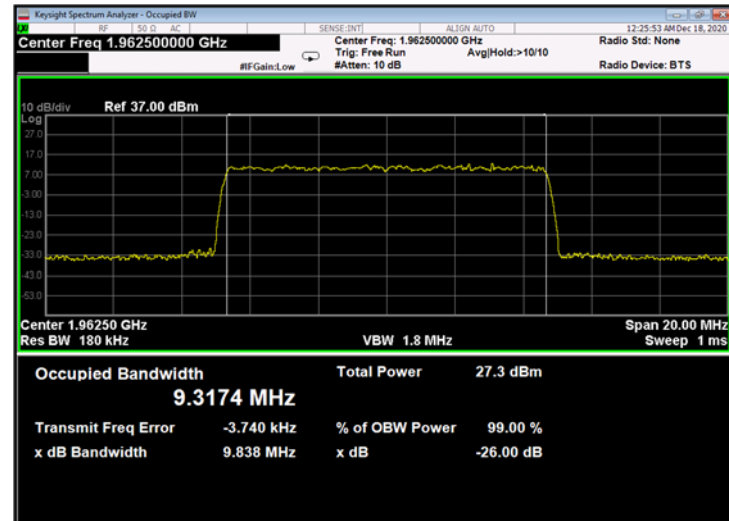
Figure 744: QPSK 10MHz B.W.; 1962.5MHz, 15kHz - Output
