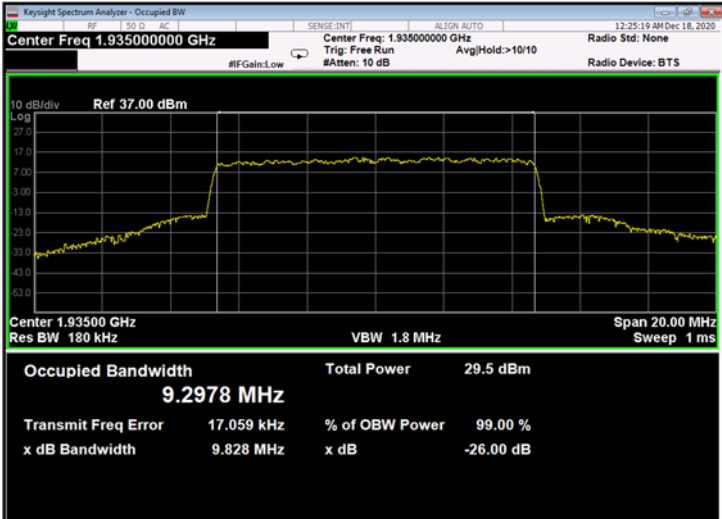
Figure 741: QPSK 10MHz B.W.; 1935.0MHz, 15kHz - Output
