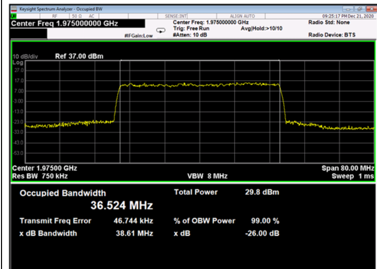
Figure 719: 256QAM 40MHz B.W.; 1975.0MHz, 60kHz - Output
