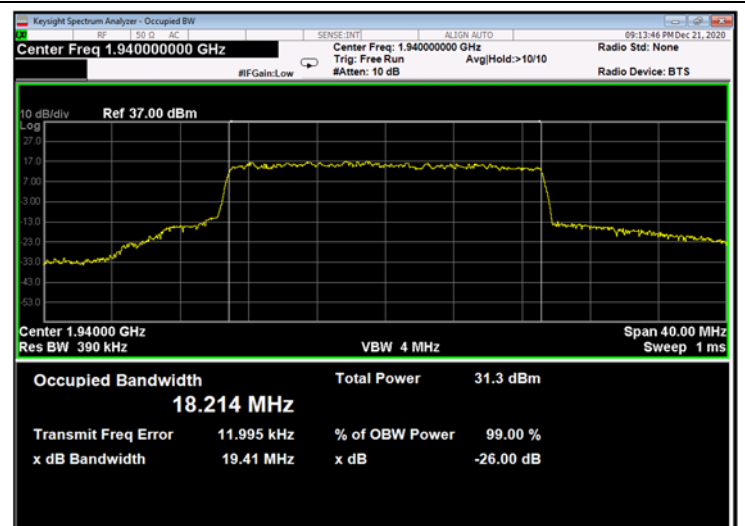
Figure 694: 256QAM 20MHz B.W.; 1940.0MHz, 30kHz - Output
