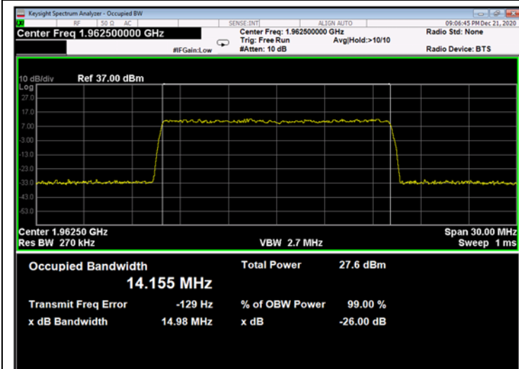
Figure 687: 256QAM 15MHz B.W.; 1962.5MHz, 15kHz - Output
