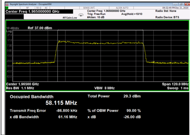
Figure 733: 256QAM 60MHz B.W.; 1965.0MHz, 30kHz - Output
