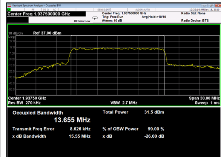
Figure 751: QPSK 15MHz B.W.; 1937.5MHz, 30kHz - Output
