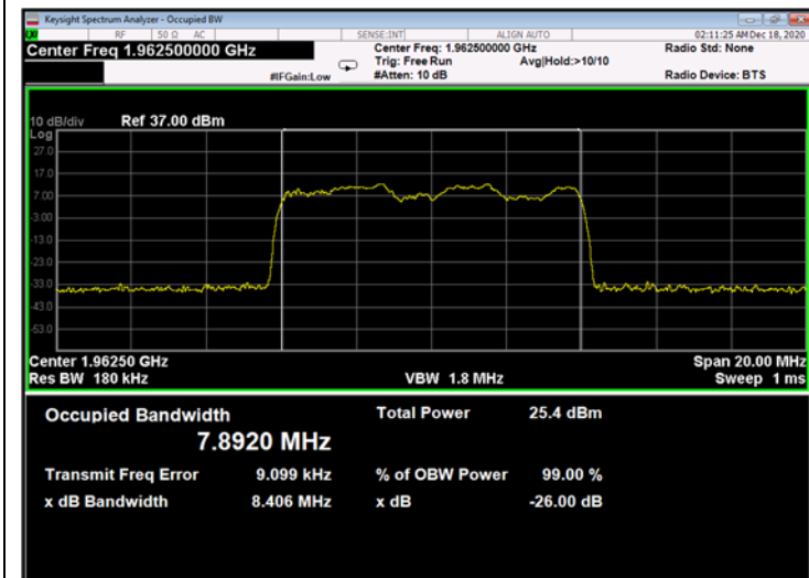
Figure 551: 16QAM 10MHz B.W.; 1962.5MHz, 60kHz - Output
