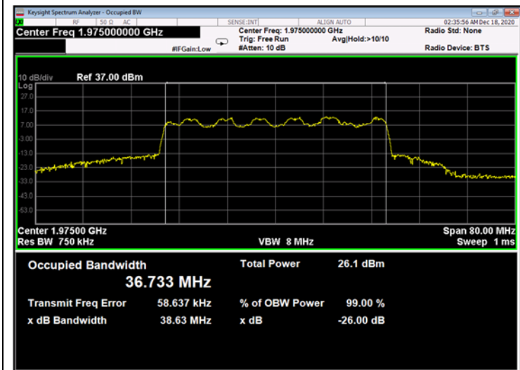
Figure 587: 16QAM 40MHz B.W.; 1975.0MHz, 60kHz - Output
