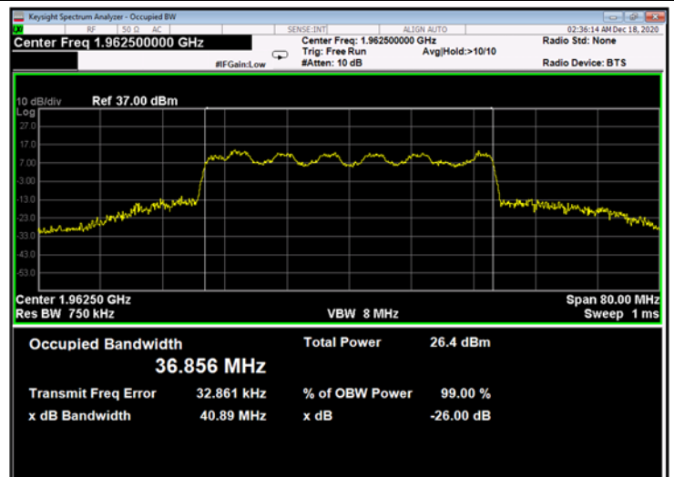
Figure 584: 16QAM 40MHz B.W.; 1962.5MHz, 60kHz - Output
