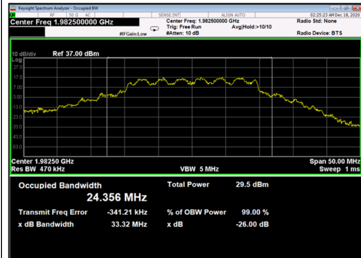
Figure 577: 16QAM 25MHz B.W.; 1982.5MHz, 30kHz - Output
