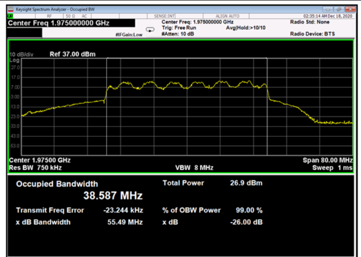
Figure 586: 16QAM 40MHz B.W.; 1975.0MHz, 30kHz - Output
