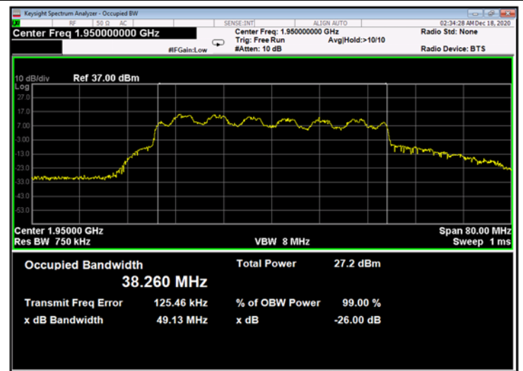
Figure 580: 16QAM 40MHz B.W.; 1950.0MHz, 30kHz - Output
