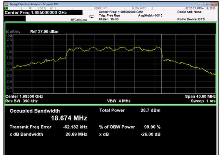
Figure 568: 16QAM 20MHz B.W.; 1985.0MHz, 30kHz - Output
