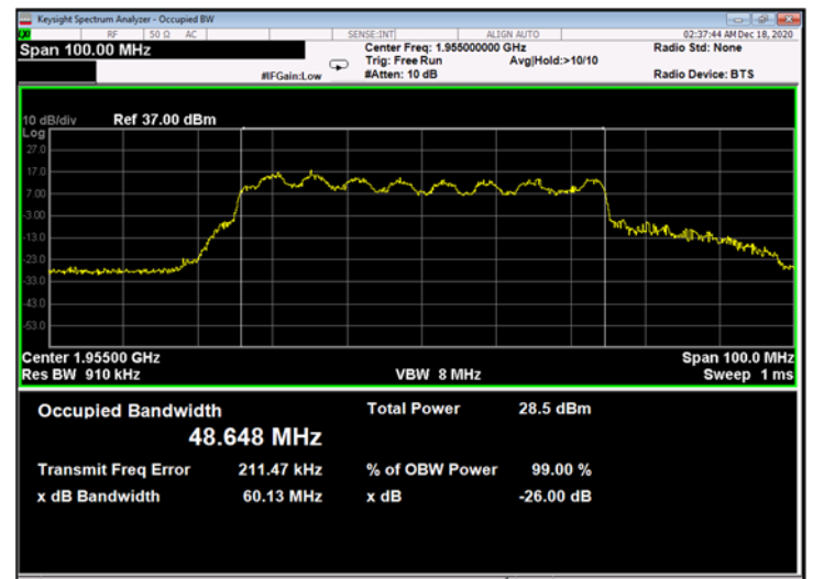
Figure 588: 16QAM 50MHz B.W.; 1955.0MHz, 15kHz - Output
