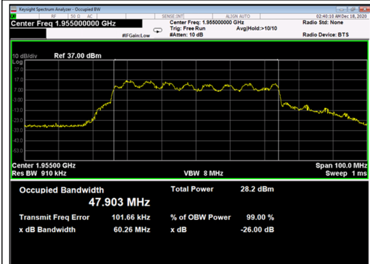
Figure 589: 16QAM 50MHz B.W.; 1955.0MHz, 30kHz - Output
