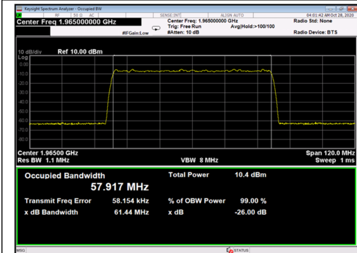
Figure 469: 256QAM 60MHz B.W.; 1965.0MHz, 30kHz - Input
