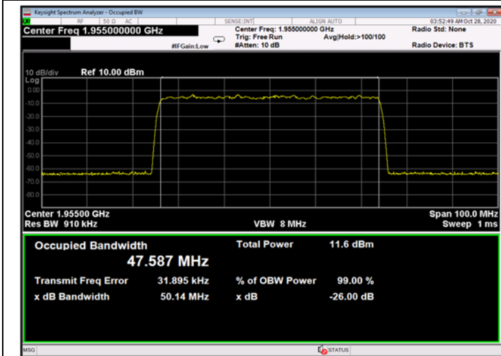
Figure 457: 256QAM 50MHz B.W.; 1955.0MHz, 30kHz - Input
