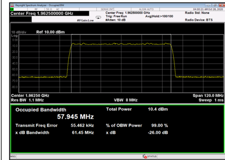
Figure 467: 256QAM 60MHz B.W.; 1962.5MHz, 30kHz - Input
