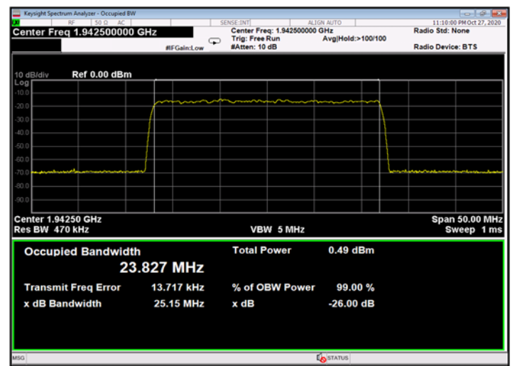
Figure 504: QPSK 25MHz B.W.; 1942.5MHz, 15kHz - Input
