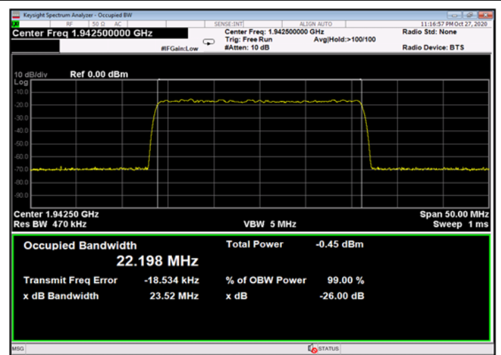
Figure 506: QPSK 25MHz B.W.; 1942.5MHz, 60kHz - Input
