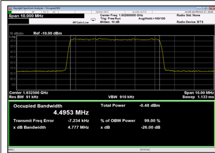
Figure 471: QPSK 5MHz B.W.; 1932.5MHz, 15kHz - Input
