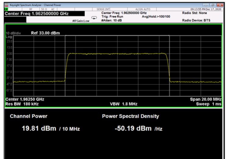
Figure 84: 64QAM 10MHz B.W.; 1962.5MHz, 15kHz
