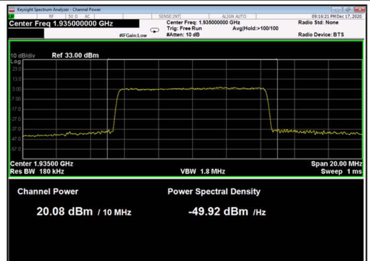
Figure 82: 64QAM 10MHz B.W.; 1935.0MHz, 30kHz
