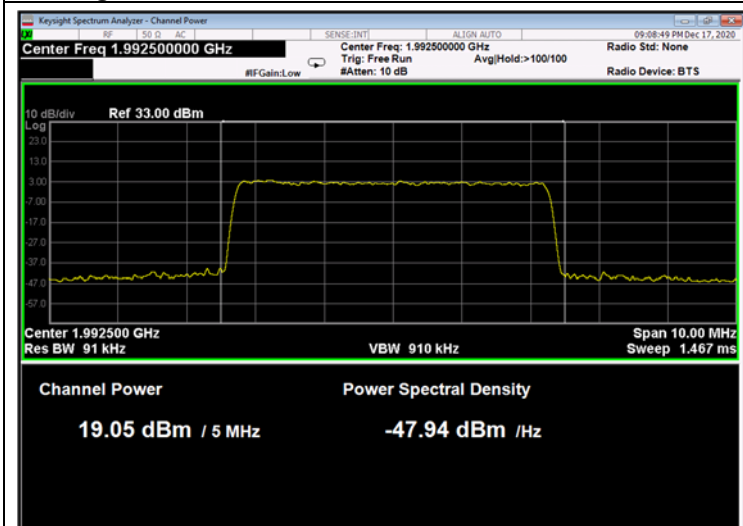
Figure 79: 64QAM 5MHz B.W.; 1992.5MHz, 15kHz
