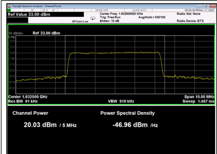
Figure 75: 64QAM 5MHz B.W.; 1932.5MHz, 15kHz
