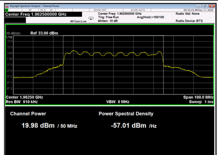
Figure 64: 16QAM 50MHz B.W.; 1962.5MHz, 30kHz
