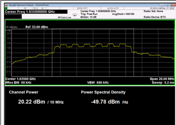
Figure 15: 16QAM 10MHz B.W.; 1935.00MHz, 15kHz
