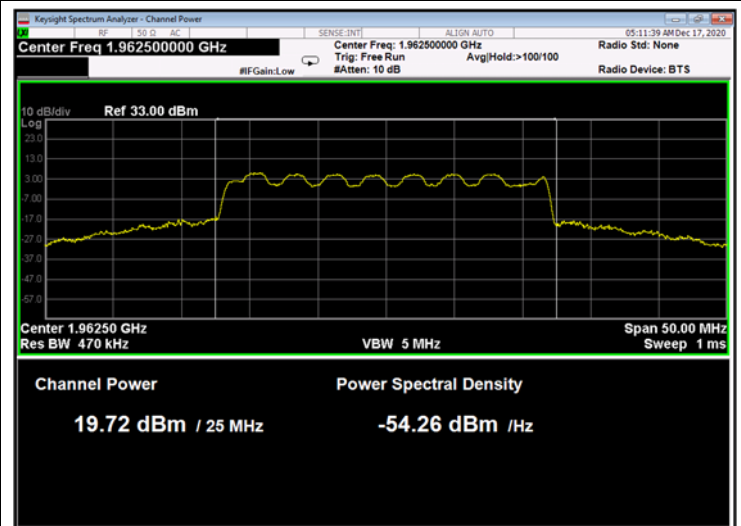
Figure 46: 16QAM 25MHz B.W.; 1962.5MHz, 30kHz
