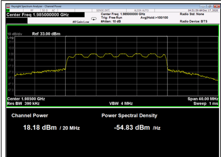
Figure 39: 16QAM 20MHz B.W.; 1985.0MHz, 15kHz
