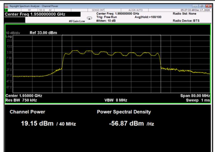
Figure 52: 16QAM 40MHz B.W.; 1950.0MHz, 30kHz
