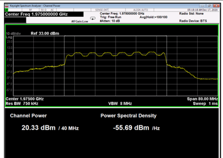
Figure 58: 16QAM 40MHz B.W.; 1975.0MHz, 30kHz
