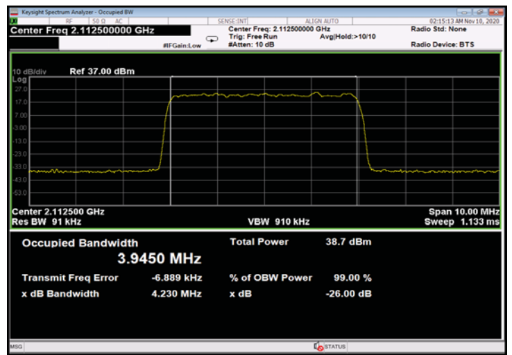
Figure 340: 64QAM 5MHz B.W.; 2112.5MHz, 30kHz - Input
