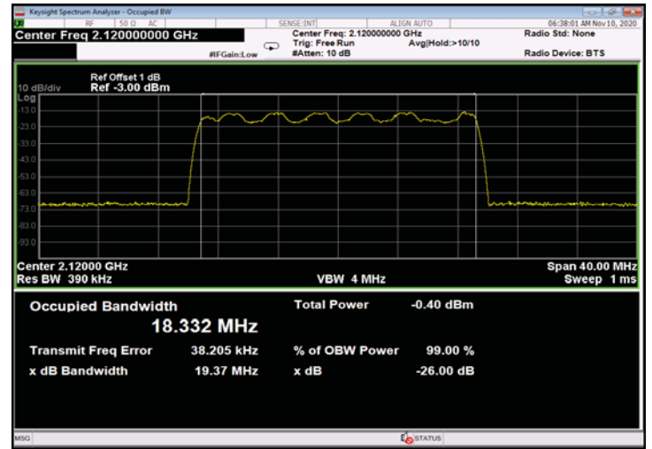
Figure 298: 16QAM 20MHz B.W.; 2120.0MHz, 30kHz - Input
