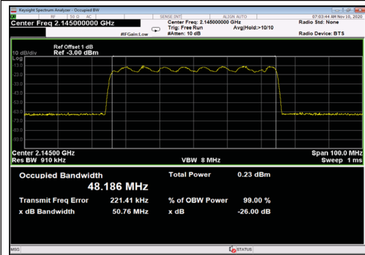
Figure 327: 16QAM 50MHz B.W.; 2145.0MHz, 15kHz - Input
