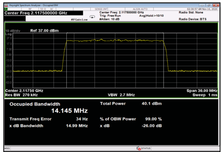
Figure 354: 64QAM 15MHz B.W.; 2117.5MHz, 15kHz - Input
