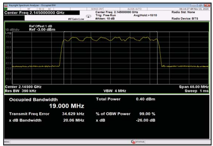
Figure 300: 16QAM 20MHz B.W.; 2145.0MHz, 15kHz - Input
