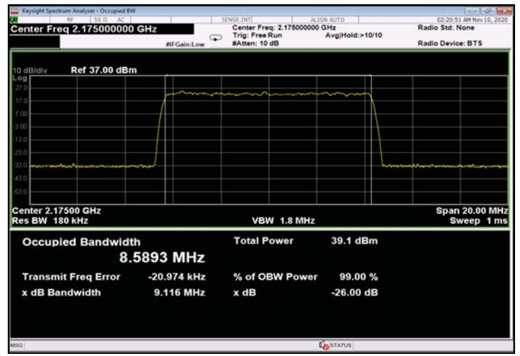
Figure 352: 64QAM 10MHz B.W.; 2175.0MHz, 30kHz - Input
