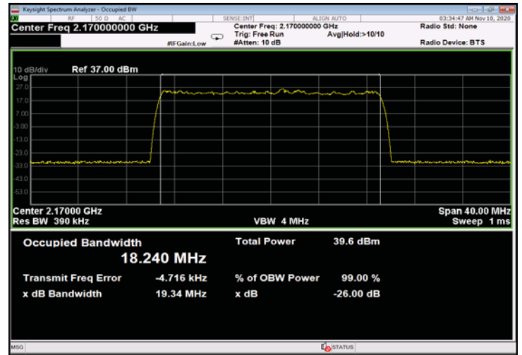
Figure 370: 64QAM 20MHz B.W.; 2170.0MHz, 30kHz - Input
