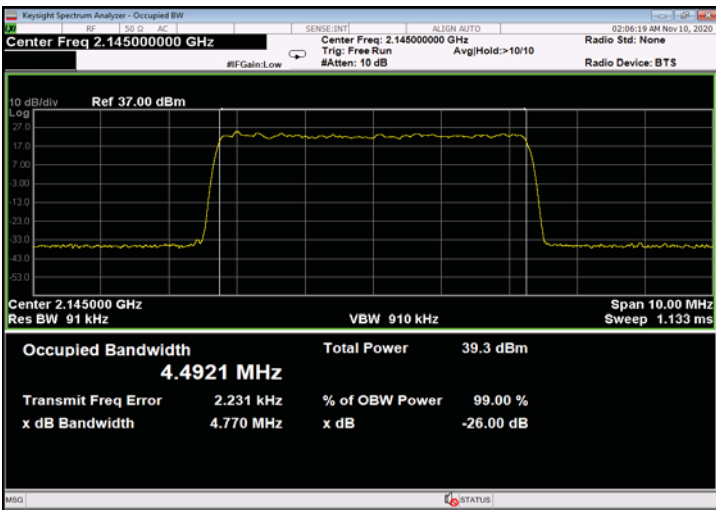
Figure 341: 64QAM 5MHz B.W.; 2145.0MHz, 15kHz - Input
