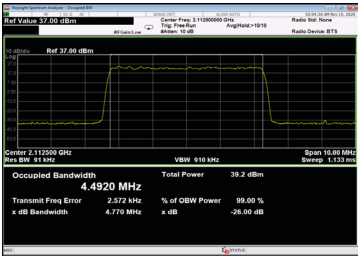
Figure 339: 64QAM 5MHz B.W.; 2112.5MHz, 15kHz - Input
