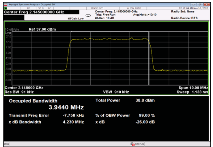
Figure 342: 64QAM 5MHz B.W.; 2145.0MHz, 30kHz - Input
