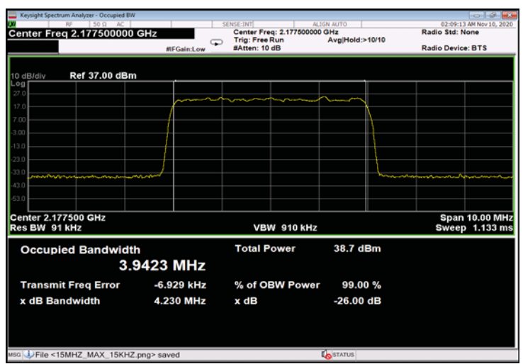
Figure 344: 64QAM 5MHz C.S.; 2177.5MHz, 30kHz - Input
