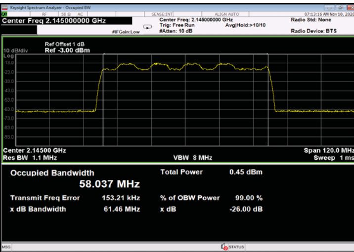
Figure 335: 16QAM 60MHz B.W.; 2145.0MHz, 30kHz - Input
