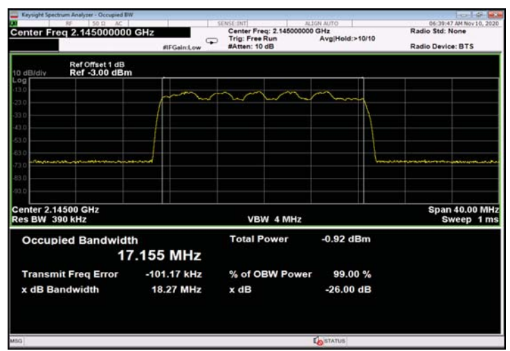
Figure 302: 16QAM 20MHz B.W.; 2145.0MHz, 60kHz - Input
