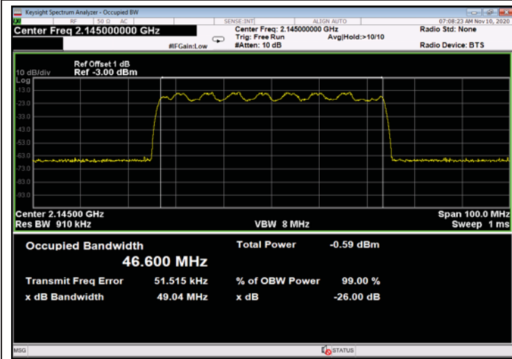
Figure 329: 16QAM 50MHz B.W.; 2145.0MHz, 60kHz - Input
