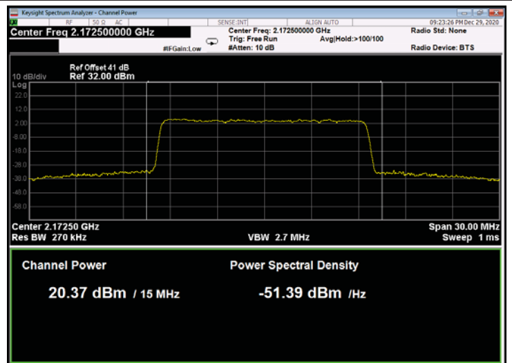
Figure 164: 256QAM 15MHz B.W.; 2172.5MHz, 60kHz
