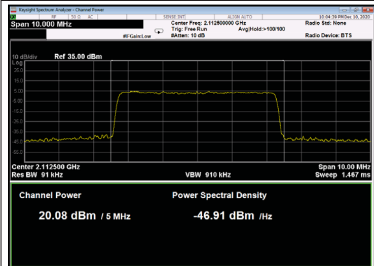
Figure 141: 256QAM 5MHz B.W.; 2112.5MHz, 15kHz
