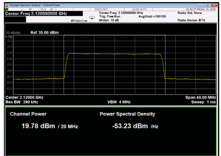
Figure 166: 256QAM 20MHz B.W.; 2120.0MHz, 30kHz
