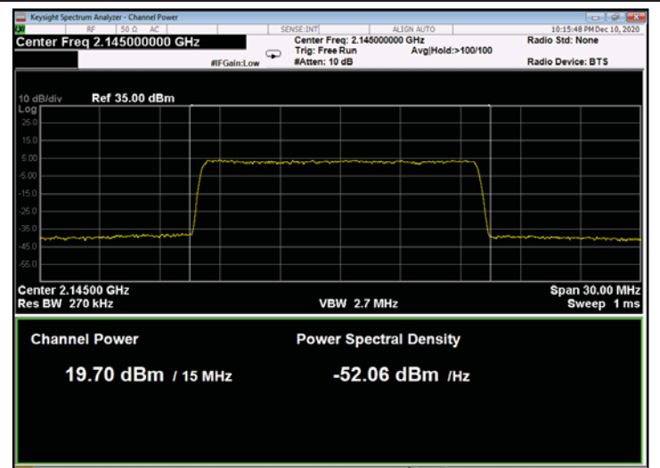
Figure 160: 256QAM 15MHz B.W.; 2145.0MHz, 30kHz
