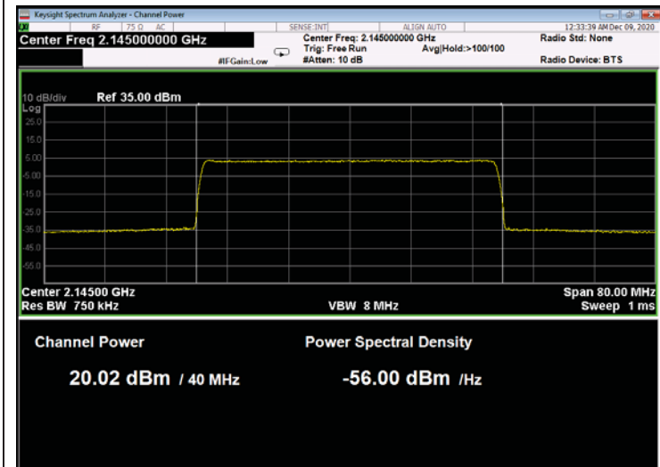
Figure 121: 64QAM 40MHz B.W.; 2145.0MHz, 30kHz
