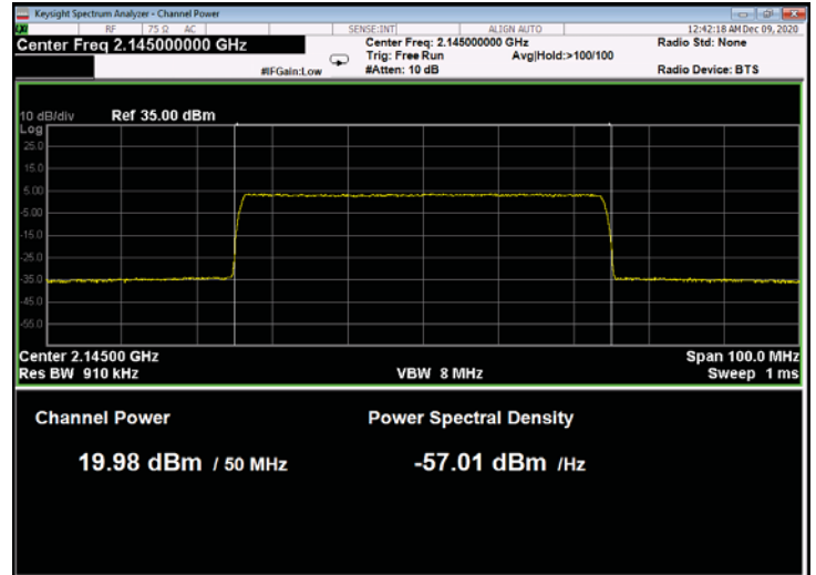
Figure 130: 64QAM 50MHz B.W.; 2145.0MHz, 30kHz
