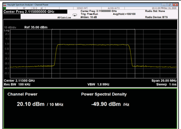
Figure 148: 256QAM 10MHz B.W.; 2115.0MHz, 30kHz
