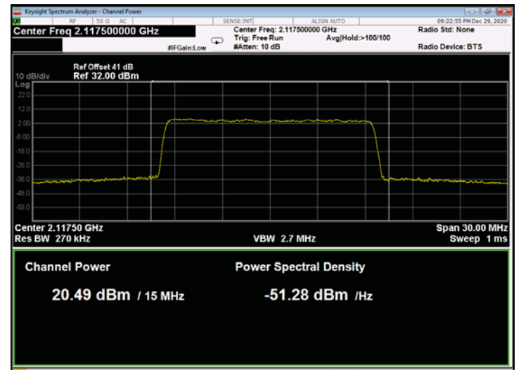
Figure 158: 256QAM 15MHz B.W.; 2117.5MHz, 60kHz
